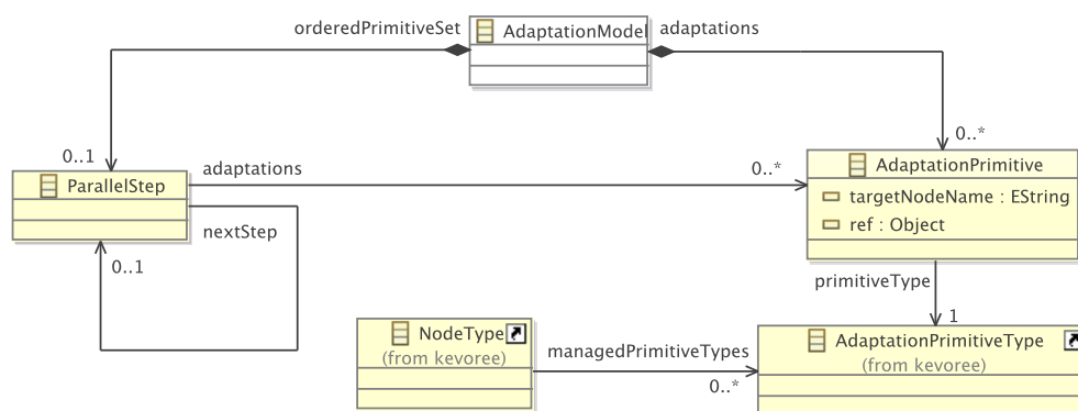
FIGURE 6.6 – Méta-modèle d'adaptation
