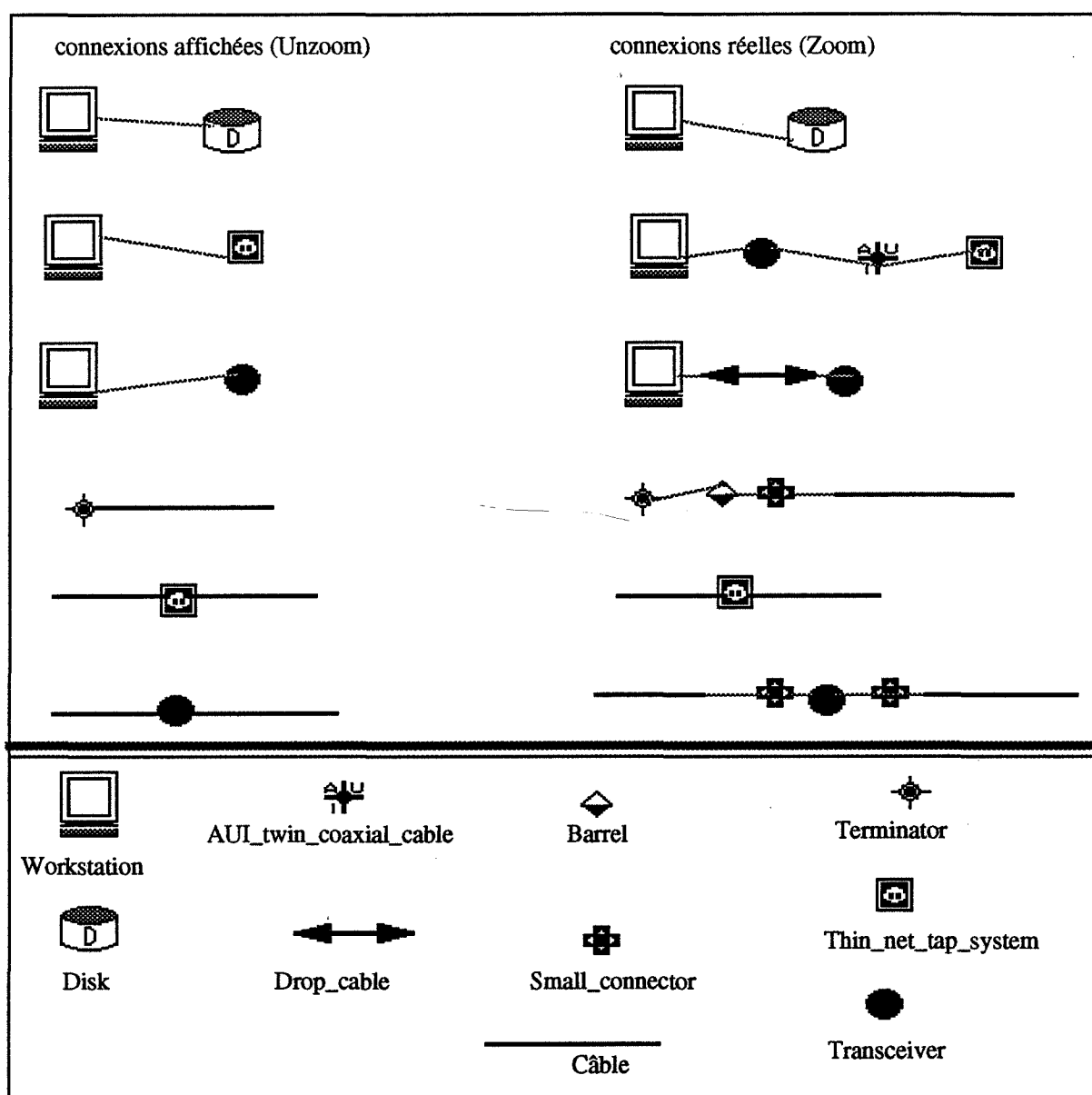
Figure 46: Les connexions
