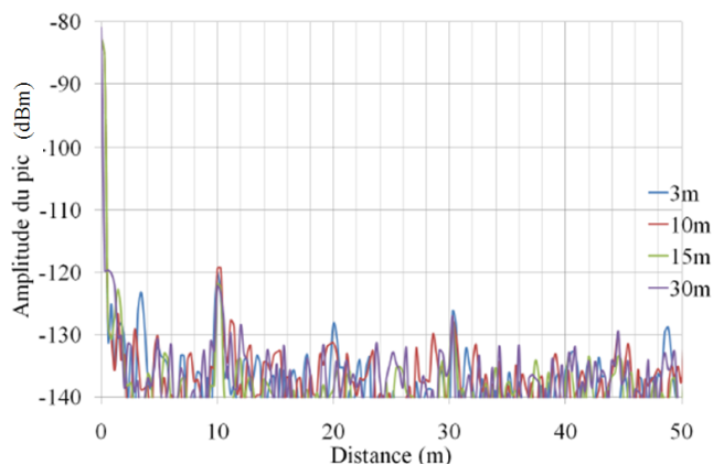
FIGURE 4.19 – Estimation de la distance maximale de détection de C3
