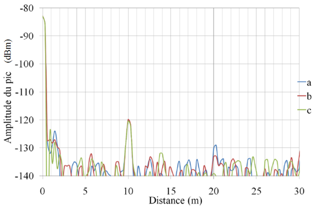
FIGURE 48 – Détection de la clé à molette à 15 m (Objet 8)
