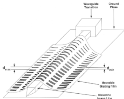
FIGURE 1.17 – LWA à balayage mécanique et fréquentiel[34]
