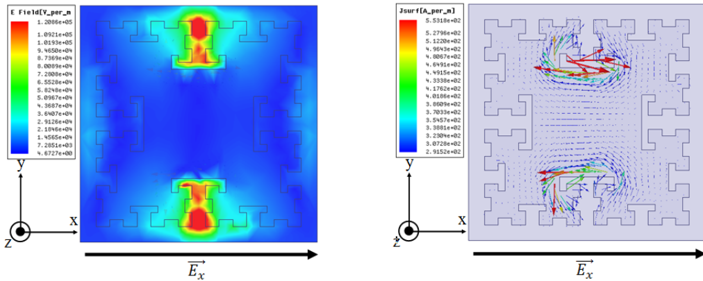
FIGURE 2.60 – Courant surfacic et champ électrique du patch fractal troisième itération
