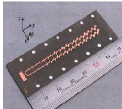
FIGURE 1.36 – Réseau linéaire de patchs inclinés de 45°[81]
