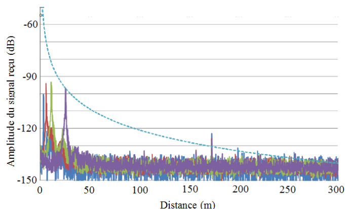
FIGURE 4.14 – Estimation de la distance de détection
