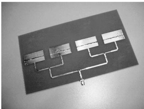
FIGURE 1.35 – Réseau linéaire de patchs avec diviseur de puissance[80]
