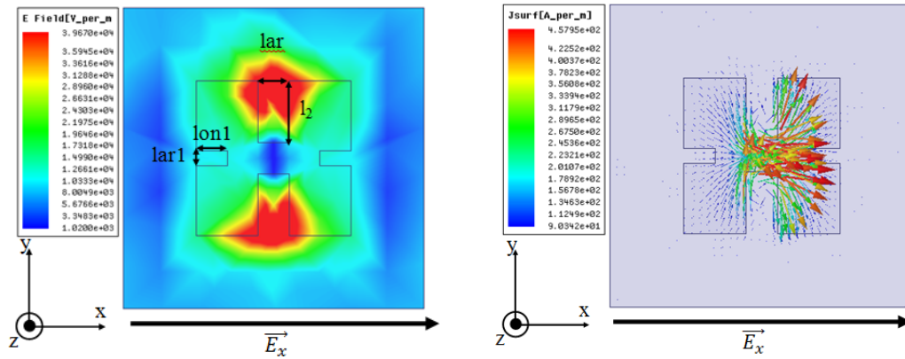
FIGURE 2.49 – Courant surfacique et champ électrique sur le patch à fentes débouchantes polarisé horizontalement
