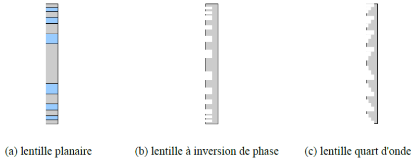
FIGURE 1.24 – Lentilles zonées
