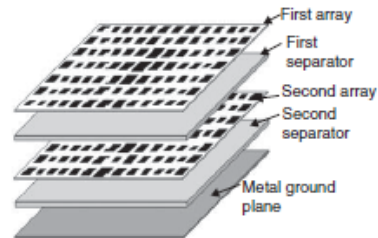
FIGURE 1.43 – Exemples de reflectarray multi-couches[18]
