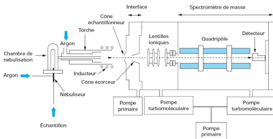
Annexe n°2 - Figure 2: Schéma de principe de l'ICP-MS
