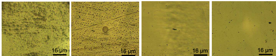
Figure 1.4-4 : Images de microscopie optique représentatives des condensats observés sur les lames de quartz pour une température comprise entre 1050^\circ C et 200^\circ C des essais B-1 (au-dessus) et B-2 (au-dessous) - grossissement \times 10
