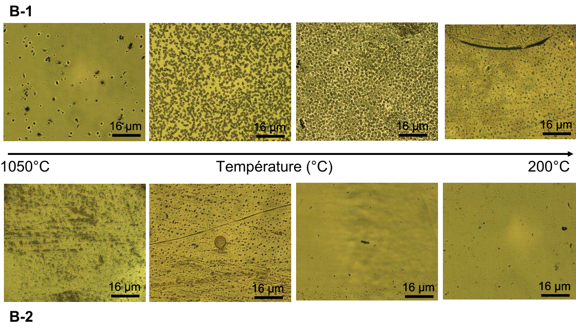
Figure 1.4-4 : Images de microscopie optique représentatives des condensats observés sur les lames de quartz pour une température comprise entre 1050 °C et 200 °C des essais B-1 (au-dessus) et B-2 (au-dessous) - grossissement \times 10
