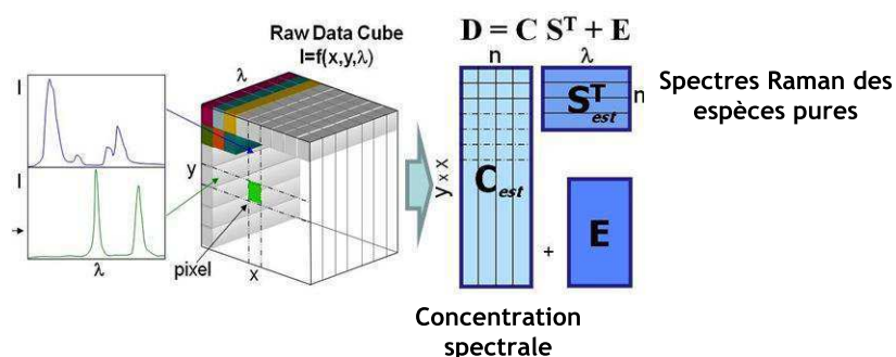
Annexe n°2 - Figure 11 : Représentation de la conversion de spectres de pixels (données expérimentales) en la matrice des spectres D utilisée dans la procédure SIMPLISMAX [1]
