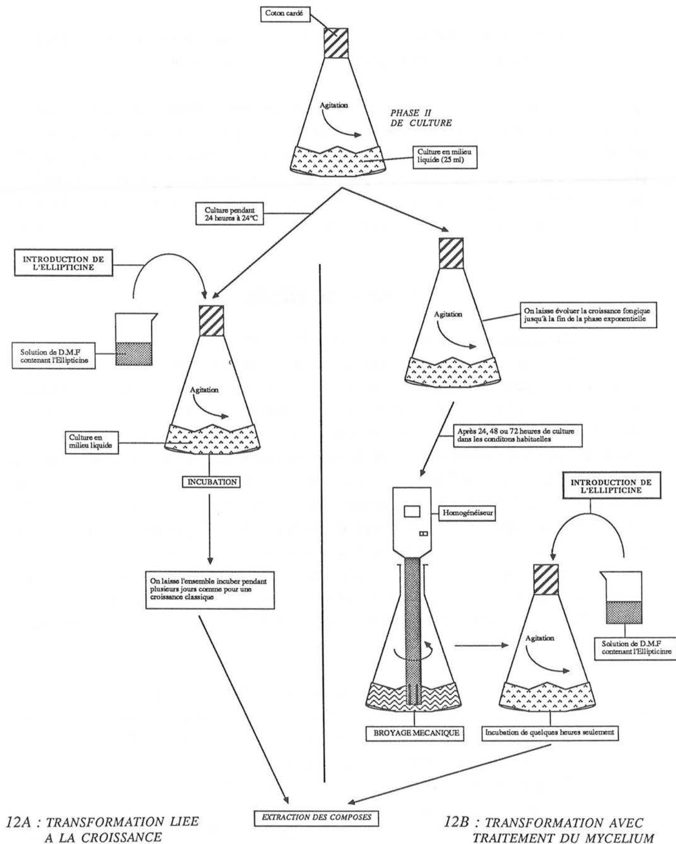
FIGURE IL.12A ET 12B : METHODOLOGIE COMPAREE DE LA BIOCONVERSION DE L'ELLIPTICINE.
