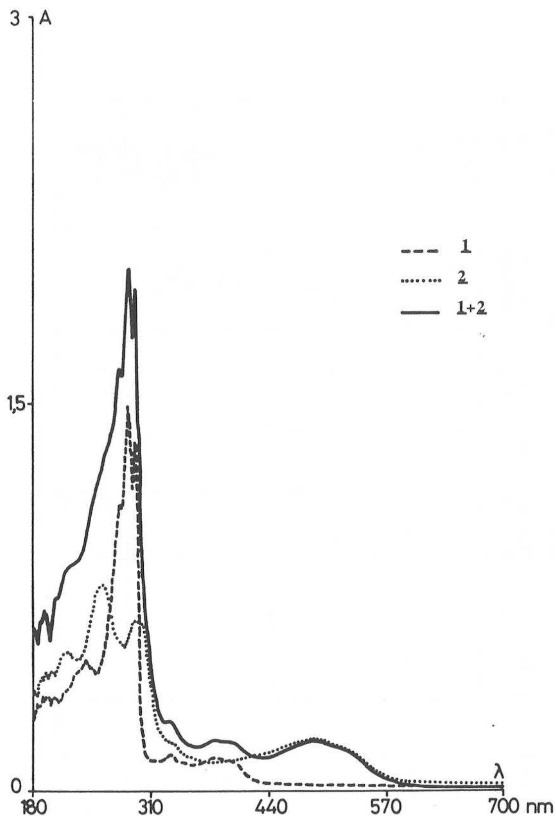
FIGURE III.7 : SPECTRE D'ABSORPTION DES SOLUTIONS OXYDEES. (1 = ELLIPTICINE, 2 = 9-OH ELLIPTICINE EN SOLUTION DANS DU METHANOL PUR A LA CONCENTRATION DE 5 \mu\text{g}.\text{ml}^{-1} ).
