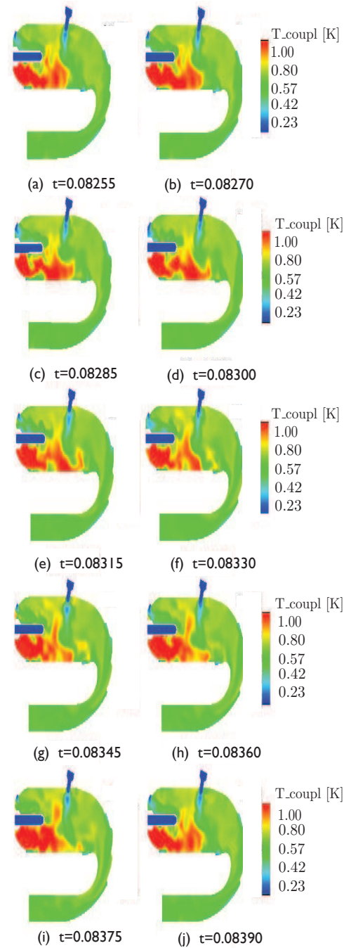
FIGURE 6.6 : Evolution temporelle du champ de température dans le plan z = 0 m. Les temps sont donnés en secondes.
