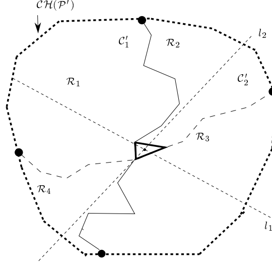
FIG. 3.5 – Partitionnement en régions de \mathcal{P}' suivant \mathcal{C}_1 et \mathcal{C}_2 .
