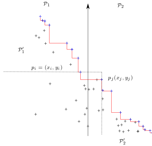
FIG. 3.7 – Les maxima définissent une structure en escalier ( |\mathcal{P}| = 100 et |\mathcal{M}(\mathcal{P})| = 18 où \mathcal{M}(\mathcal{P}) est l'ensemble des maxima de \mathcal{P} ).
