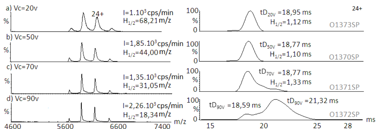
Figure 15 : Effet de la tension d'accélération Vc sur les spectres MS et IM-MS. Analyse de l'ADH (1 μM en tétramère) dessalée 2 fois par filtration sur gel (Zeba, tampon AcNH 4 150 mM pH 6.8). Panel de gauche : spectres de masse accumulés, sur 19 scans de 4 secondes. L'intensité est indiquée en coups/min. Panel de droite : mobilogrammes extraits de l'état de charge 24+. a-d) Effet de la tension d'accélération Vc (Trap CE = 10V, Transfer CE = 0V, Bias = 50V, Pi = 6 mbar, Q He /Q N2 = 180/90).
