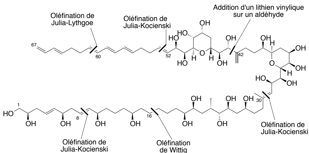
Schéma 25 : Schéma des disconnections proposées par L.A. Paquette
