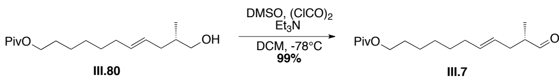
Schéma 174 : Oxydation de Swern de III.80
