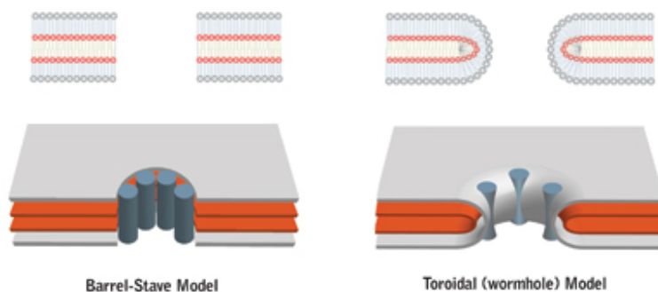
Figure 2 : Schémas de pores en tonneaux et toroïdaux
