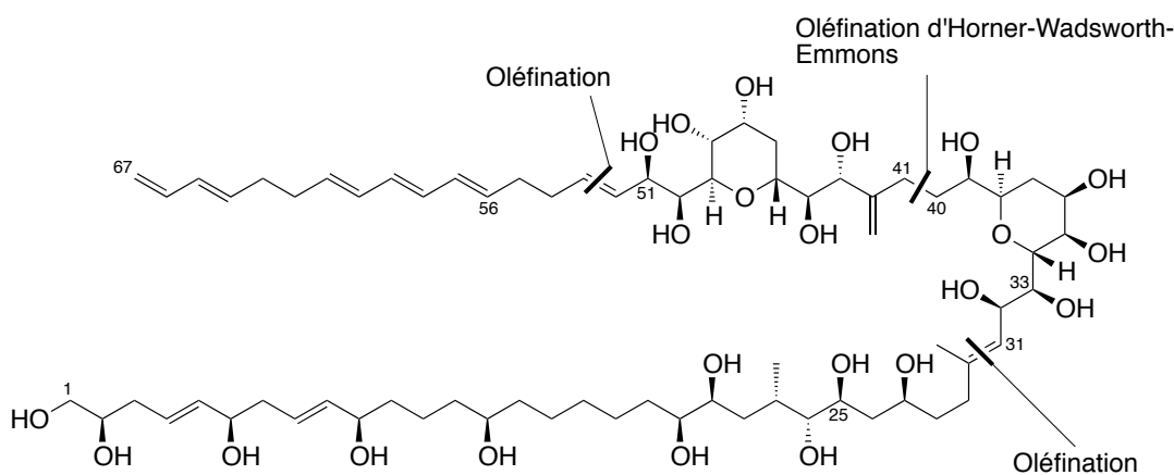
Schéma 69 : Schéma des disconnections proposées par M. T. Crimmins
