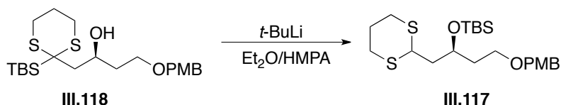
Schéma 190 : Réarrangement de Brook de III.118
