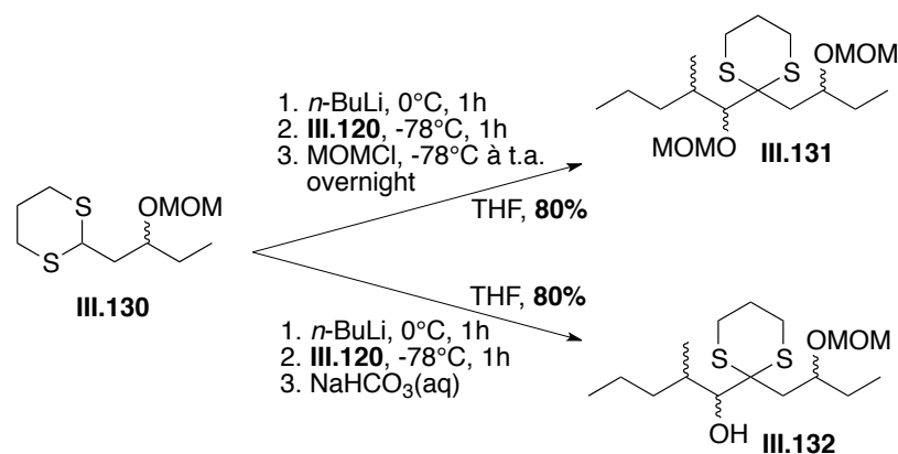
Schéma 198 : Coupages entre III.130 et III.120
