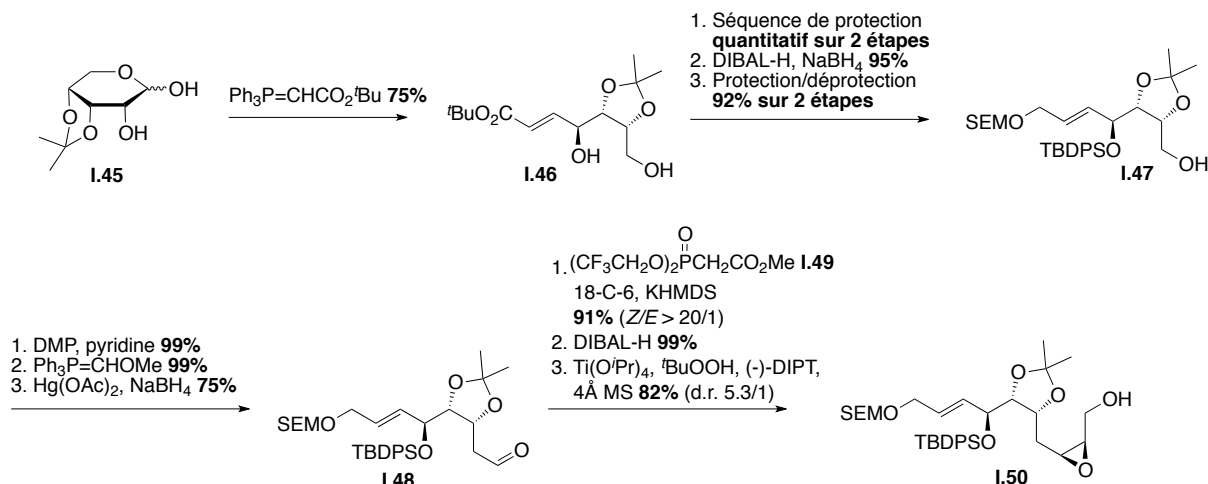
Schéma 27 : Synthèse de l'époxyde I.50
