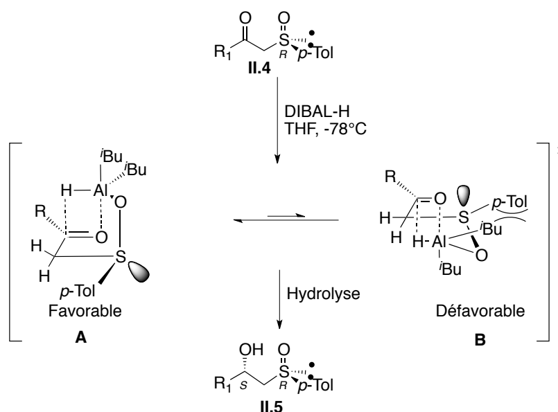
Schéma 86 : Etats de transition de la réduction d'un \beta -cétosulfoxyde par le DIBAL-H
