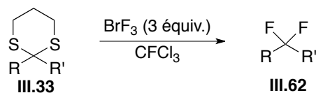
Schéma 157 : Fluoration de 1,3-dithianes
