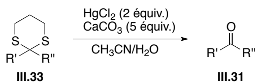
Schéma 148 : Hydrolyse des 1,3-dithianes catalysée par \text{HgCl}_2
