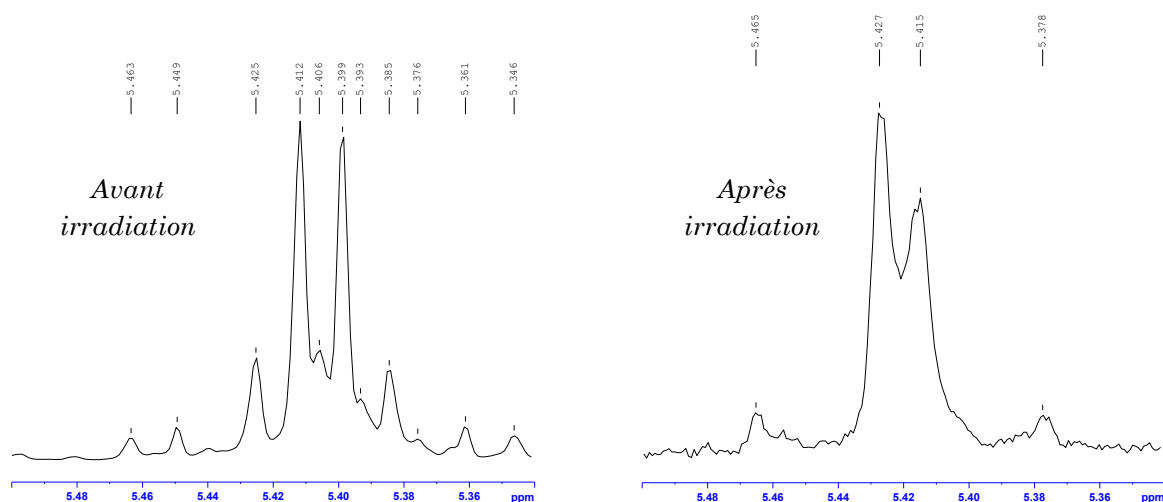
Figure 3 : Spectre 400 MHz RMN ^1\text{H} des protons vinyliques avant et après irradiation
