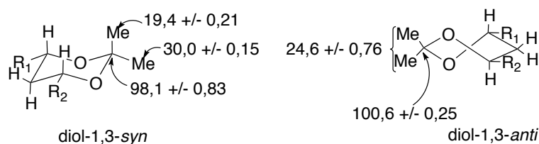
Schéma 99 : Déplacements chimiques des carbones d'un acétone-1,3 en fonction de la configuration relative des deux alcools (ppm)
