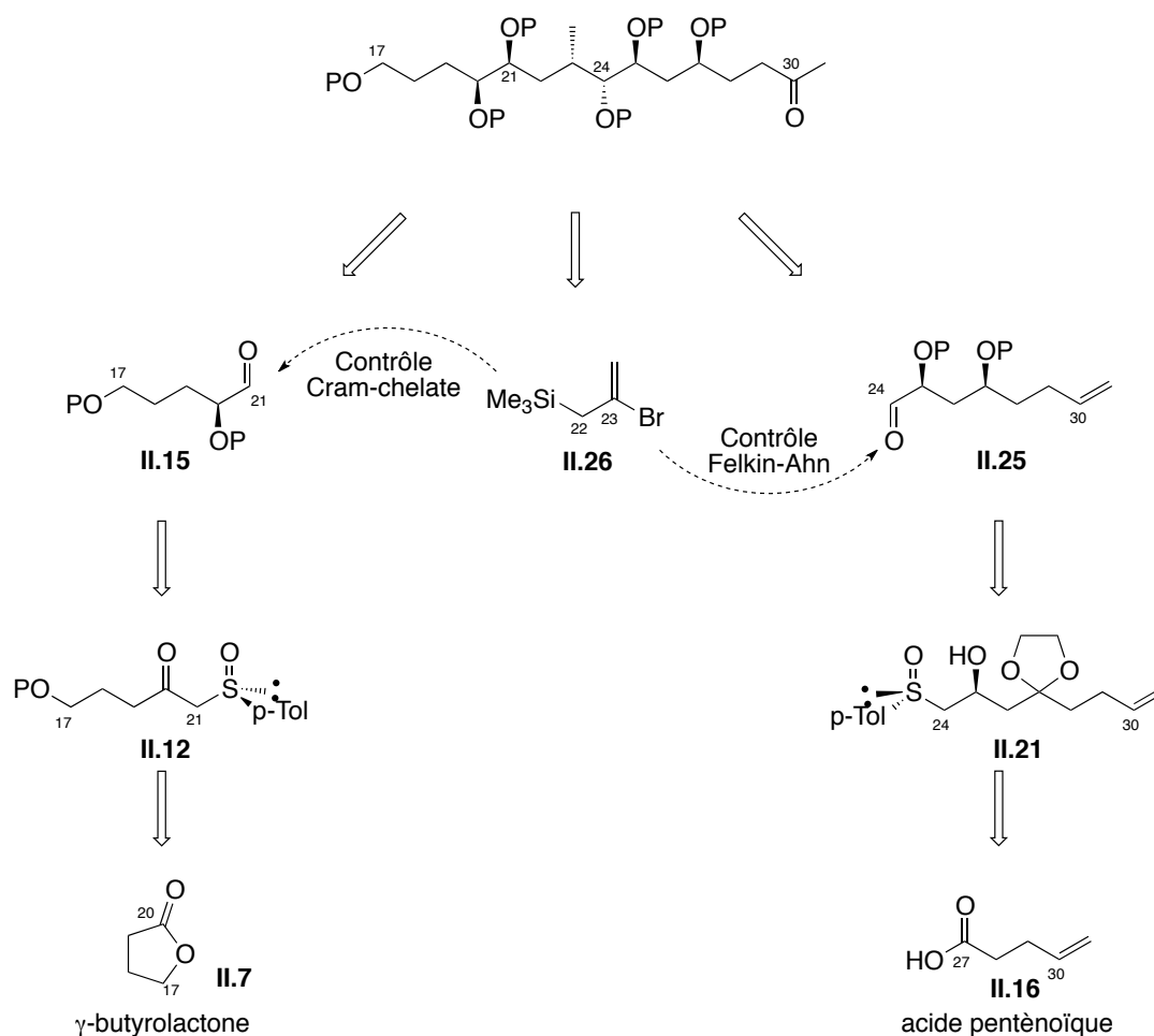
Schéma 79 : Schéma rétrosynthétique du fragment C17-C30
