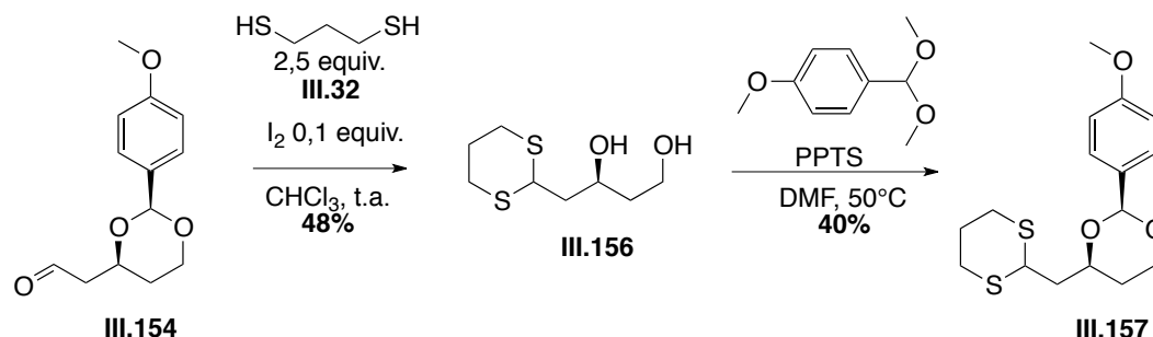
Schéma 213 : Synthèse du dithiane III.157
