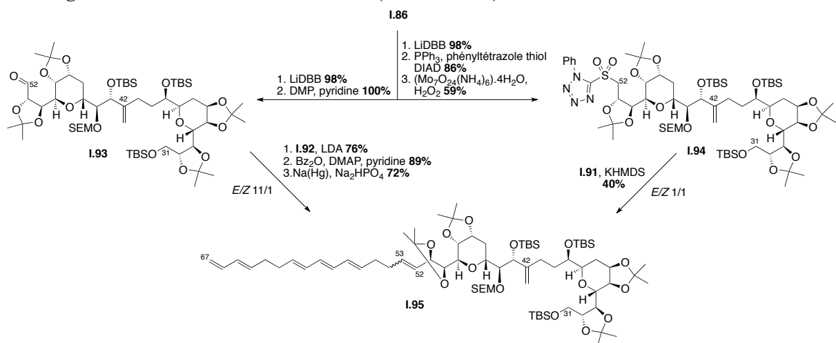
Schéma 43 : Synthèse du fragment C31-C67
