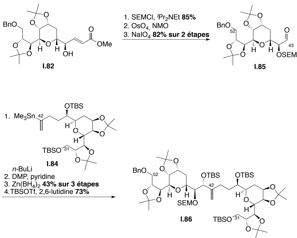
Schéma 39 : Synthèse du fragment C31-C52
