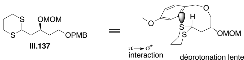
Schéma 208 : Interaction entre les électrons \pi du groupement PMB et l'orbitale \sigma^*
