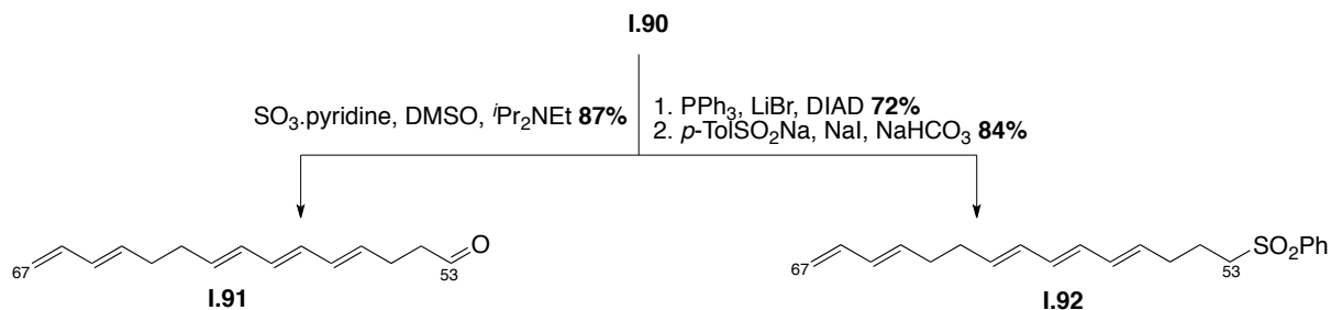
Schéma 42 : Synthèse des deux précurseurs du fragment C53-C67
