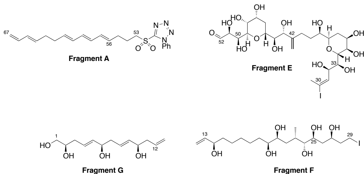
Schéma 129 : Fragments issus des nouvelles disconnections
