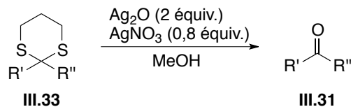
Schéma 150 : Hydrolyse des 1,3-dithianes catalysée par \text{Ag}_2\text{O}
