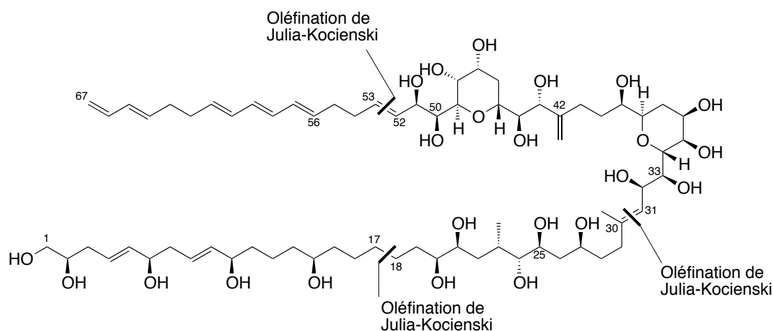
Schéma 56 : Disconnections proposées par J. Cossy/F. Colobert/I.E. Makó
