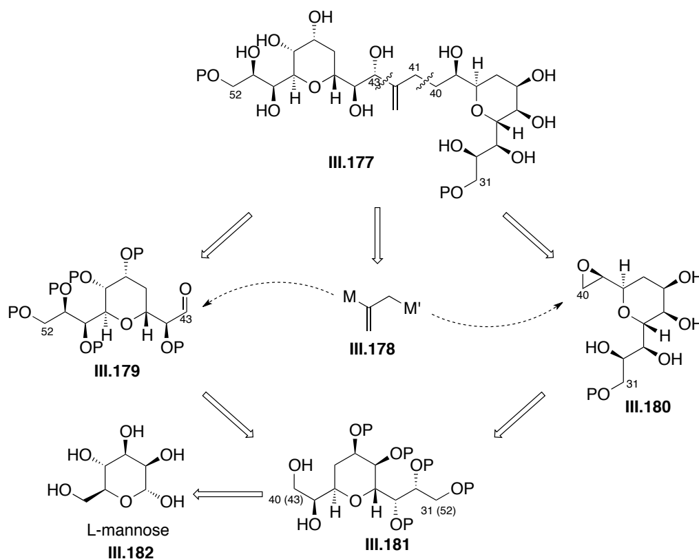
Sch  ma 229 : R  trosynth  se du fragment t  trahydropyranique envisag   par le groupe de J. Cossy
