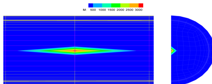
Figure (IV.35) : Anomalie de la solution reconstruite issue d'une variation de rayon
