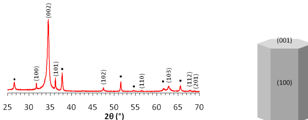
Figure III-11 : Diagramme de DRX du ZnO poreux électrodéposé
