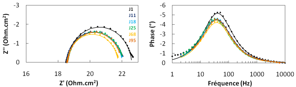
Figure IV-38 : Spectres d'impédance à la V_{OC} sous 1 soleil AM 1,5G dans le temps des cellules ZnO/D149/D131/acide octanoïque
