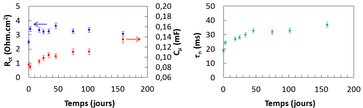
Figure IV-36 : Evolution des paramètres R_{ct} , C_{\mu} et \tau_n d'une cellule ZnO/D149/acide octanoïque
