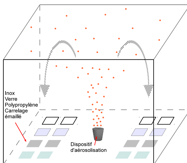
FIGURE 4.1: Schéma du dispositif expérimental
