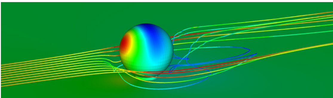
FIGURE 7.12: Écoulement autour d'une sphère à Reynolds local = 100. Pression sur la sphère et vitesse sur les lignes de champ.
