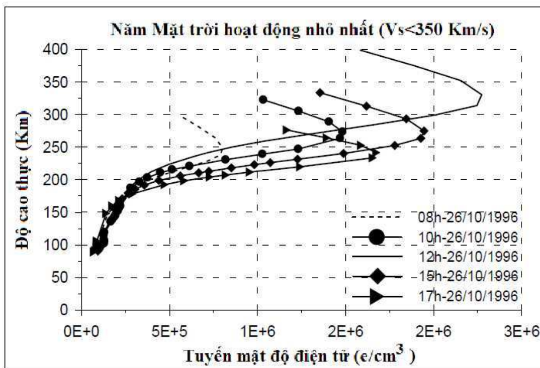
Hình 1. Tuyến mật độ điện tử ở các giờ khác nhau của ngày 26/10/1996 ở năm Mặt trời hoạt động nhỏ nhất đặc trưng cho các thời điểm của mùa thu.
