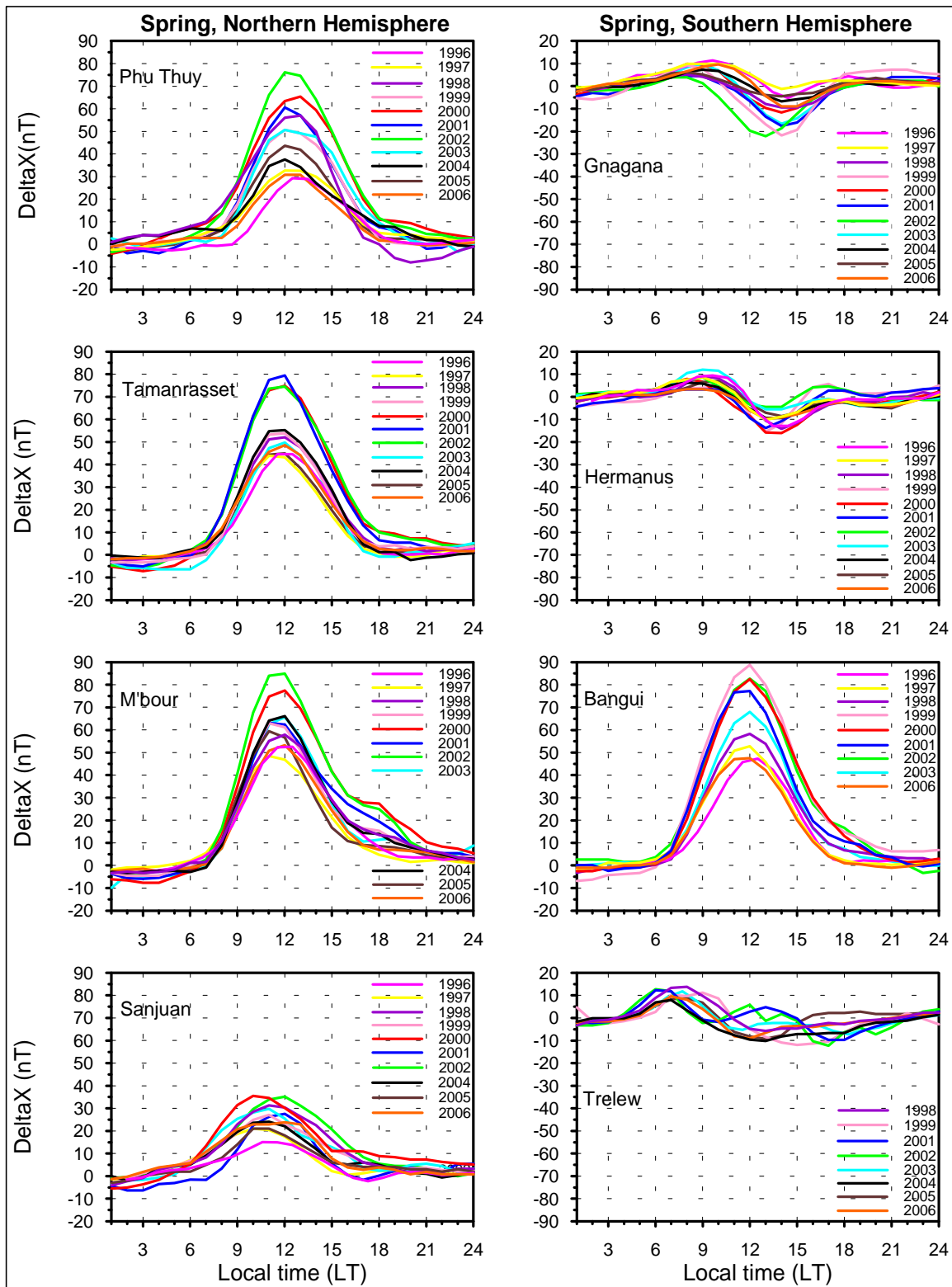
Figure 3.28: Variation diurne de \Delta X en printemps à Phu Thuy, Gnanagara, Tamnarasset, Hermanus, M'Bour, Bangui, San Juan et Trelew, pour les années de 1996 à 2006 avec am < 20nT
