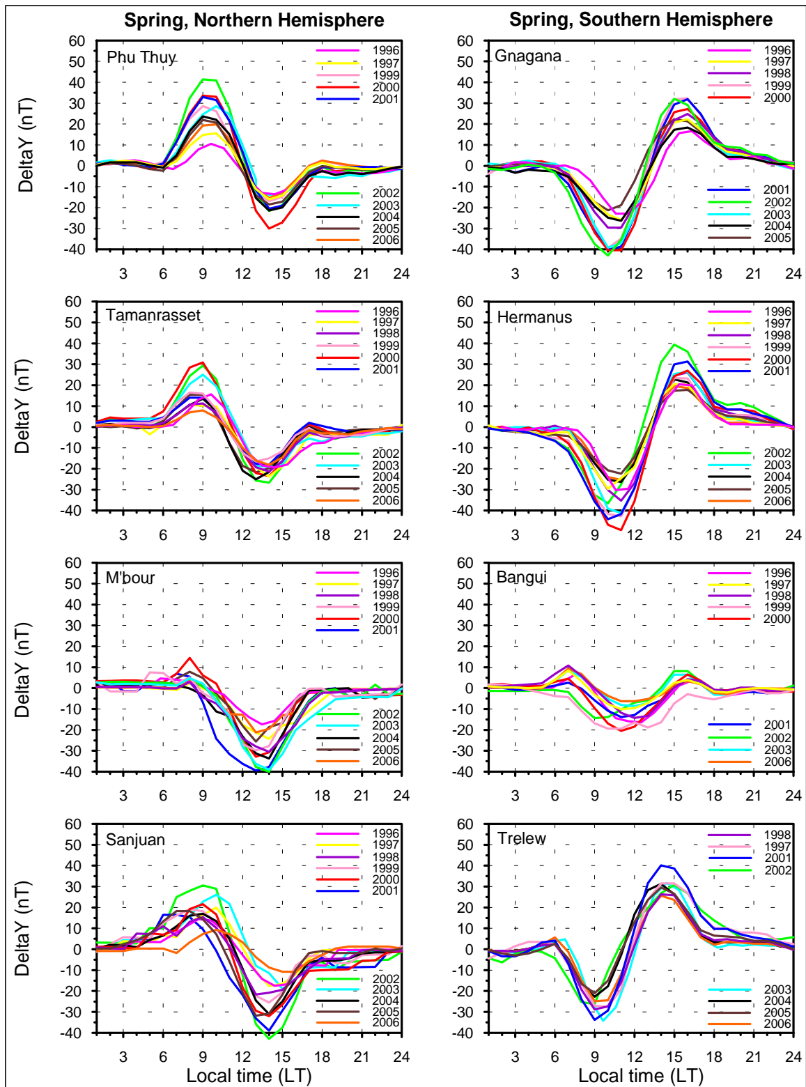
Figure 3.29: Variation diurne de \Delta Y en printemps à Phu thuy, Gnangara, Tamnarasset, Hermanus, M'Bour, Bangui, San Juan et Trelew, pour les années de 1996 à 2006 avec am < 20nT
