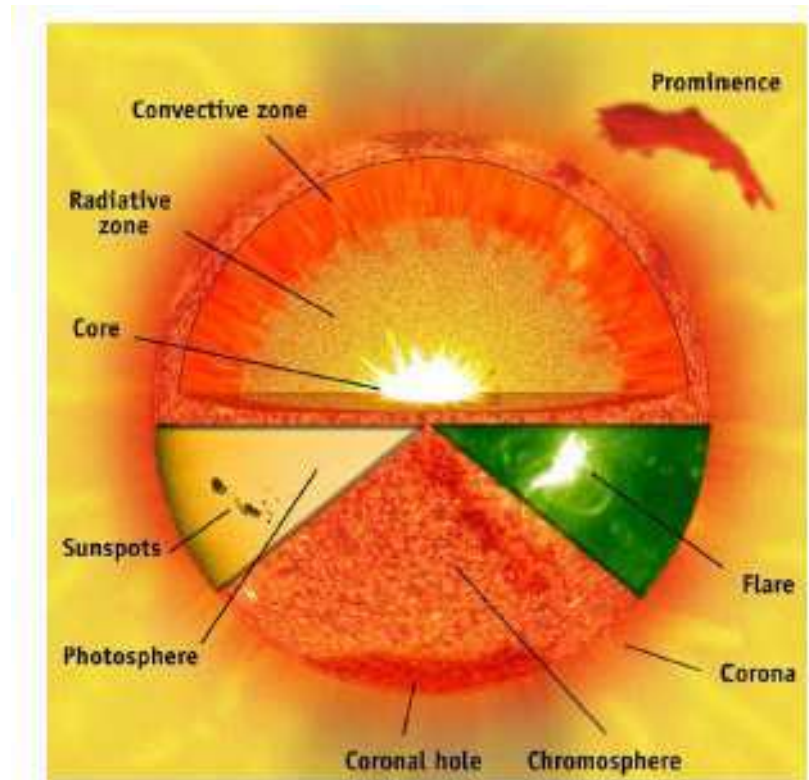
Figure 1.1 Présentation de la structure interne et de quelques particularités de la surface comme les taches solaires du Soleil. ESA, NASA
