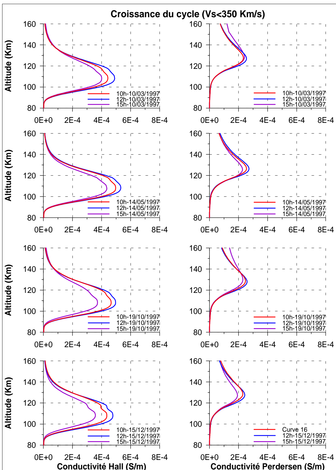
Figure 3.16: Les profils des conductivités ionosphériques de Hall, de Pedersen à différentes heures des journées pour les 10/03/1997, 14/05/1997, 19/10/1997 et 15/12/1997 à la phase croissante cycle.
