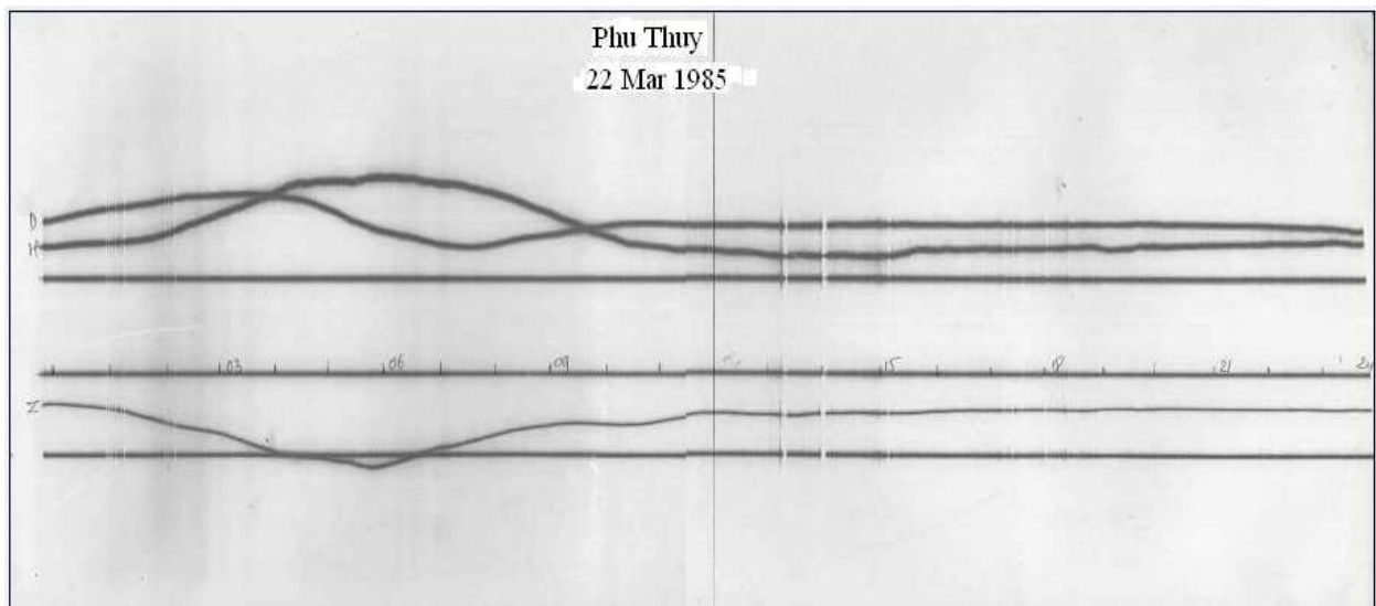
Figure 2.6: Une magnétogramme à Phu Thuy le 22 Mars 1985.
