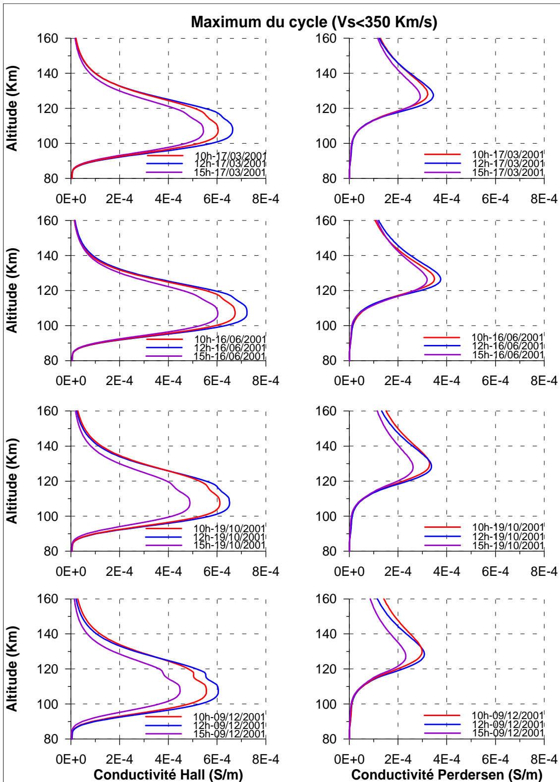
Figure 3.17: Les profils des conductivités ionosphériques de Hall, de Pedersen à différentes heures des journées pour les 17/03/2001, 16/06/2001, 19/10/2001 et 09/12/2001 au maximum du cycle de taches.
