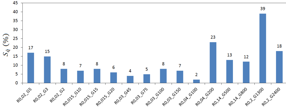
FIGURE 3.29 – Pourcentage de déséquilibre du flux de chaleur entre l'entrée et la sortie du canal dans un plan 2D, pour un canal adiabatique.
