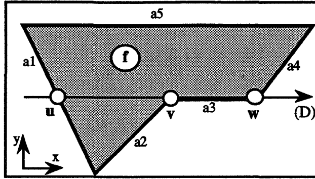
Figure 10. La face f présente 5 contacts avec le plan Q (droite D sur la figure), qui sont: c_1 = (u, 1, \text{nil}, a_1) , c_2 = (v, 0, \text{nil}, \text{nil}) , c_3 = (v, 0, a_3, \text{nil}) , c_4 = (w, 0, \text{nil}, \text{nil}) , c_5 = (w, 1, \text{nil}, \text{nil}) . On note que c_1 porte une sécante a_1 ; c_3 porte une tangente a_3 ; c_2 et c_3 coïncident au point v ; c_4 et c_5 coïncident au point w . Sur l'exemple, on suppose que les points au "dessus" du plan Q (la droite D de la figure) ont des puissances positives.
