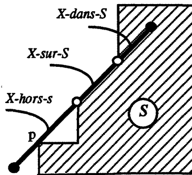
Figure 2. Classification d'un segment X par rapport à un polygone S . Le point p , bien qu'appartenant à \partial S , est exclu de X\text{-sur-}S par régularisation.
