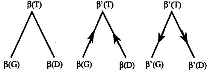
Figure 9. A gauche, l'état initial des boîtes en un nœud T donné. Au centre, l'état des boîtes après une montée : \beta'(T) = \beta(T) \sqcap (\beta(G) \% \beta(D)) , où \% désigne l'opération portée par T . A droite, l'état final des boîtes après une phase supplémentaire de descente : \beta'(G) = \beta'(T) \sqcap \beta(G) et \beta'(D) = \beta'(T) \sqcap \beta(D) .
