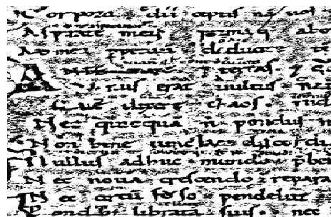
(Sauvola, [1997])
