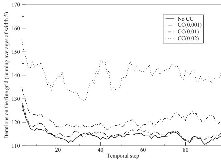
FIGURE 6.28 – Nombre d’itérations du solveur sur le maillage fin à chaque pas de temps, pour différentes valeurs de C_N , pour une simulation sur 4 coeurs de calcul sur un maillage à 1,7 millions d’éléments du brûleur Preccinsta .
