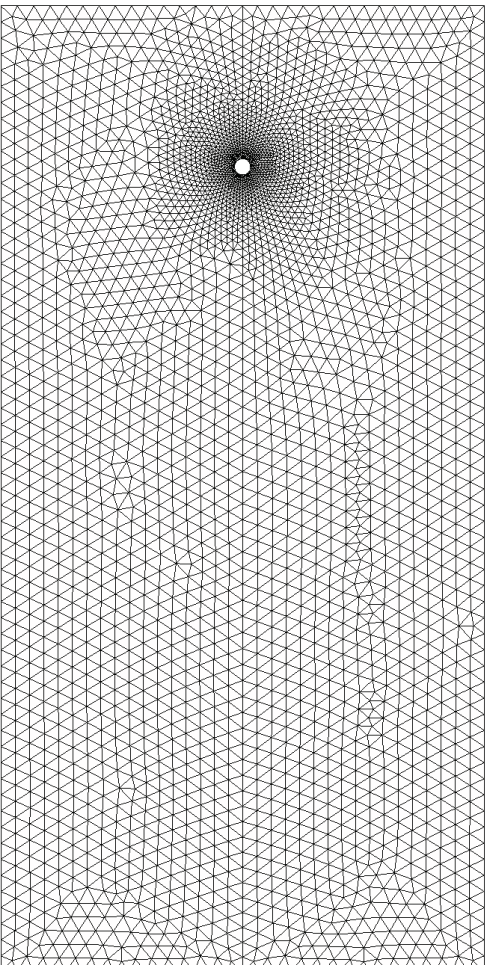
FIGURE 6.21 – Vue du dessus d'un maillage de 491 000 éléments sur le domaine du cas-test Cylindre_3D.
