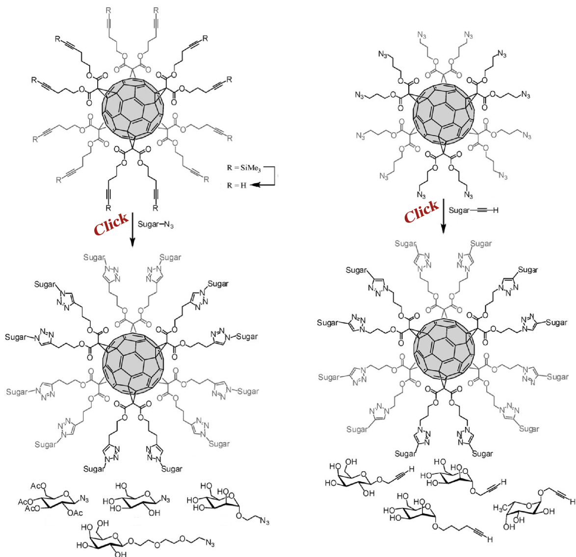
Figure 4.4: Méthodologie développée au laboratoire pour incorporer de façon régiosélective 12 sucres. 14 Les deux synthons hexa-adduits alcyne (vrais ou protégés) et azoture permettent d'obtenir de façon relativement aisée des composés sucres inaccessibles par une autre voie de synthèse.
