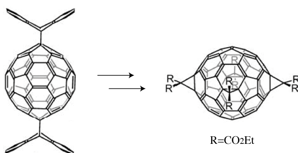
Figure 5.8: Addition topo-chimique d'anthracènes sur la position trans-1 menant à la formation régio-spécifique d'un tétra-adduit.
