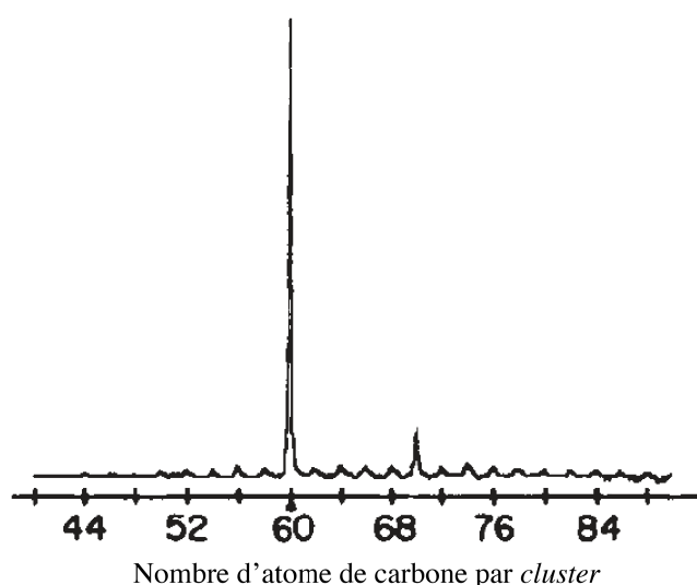
Figure 1.1: Spectre de masse (MALDI-TOF) obtenu par Smalley, Curl et Kroto. 5
