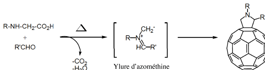
Figure 1.9: Cycladdition 1,3-dipolaire. La formation de fulleropyrrolidines passe par un intermédiaire réactionnel, un ylore d'azométhine.
