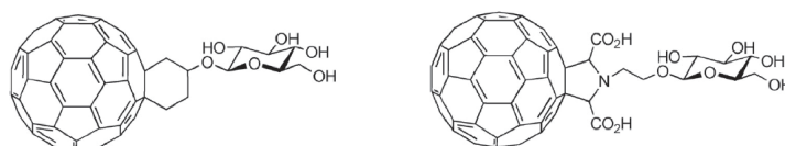
Figure 4.2: Fullerènes synthétisés par le groupe de Toshima 5,6 photodégradant la protéase du VIH-1.
