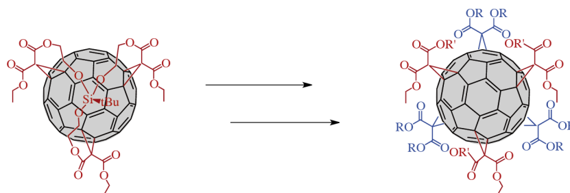
Figure 5.27: Groupe directeur permettant une répartition des fonctions en deux zones topologiques. Une troisième zone topologique peut être envisagée en remplaçant les éthyles par une autre fonctionnalité.
