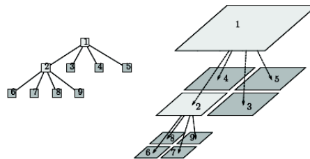
FIGURE 2.16 – Représentation d'une cellule quad-tree. Les cellules blanches sont des cellules parents et les cellules grises sont des cellules enfants [126].
