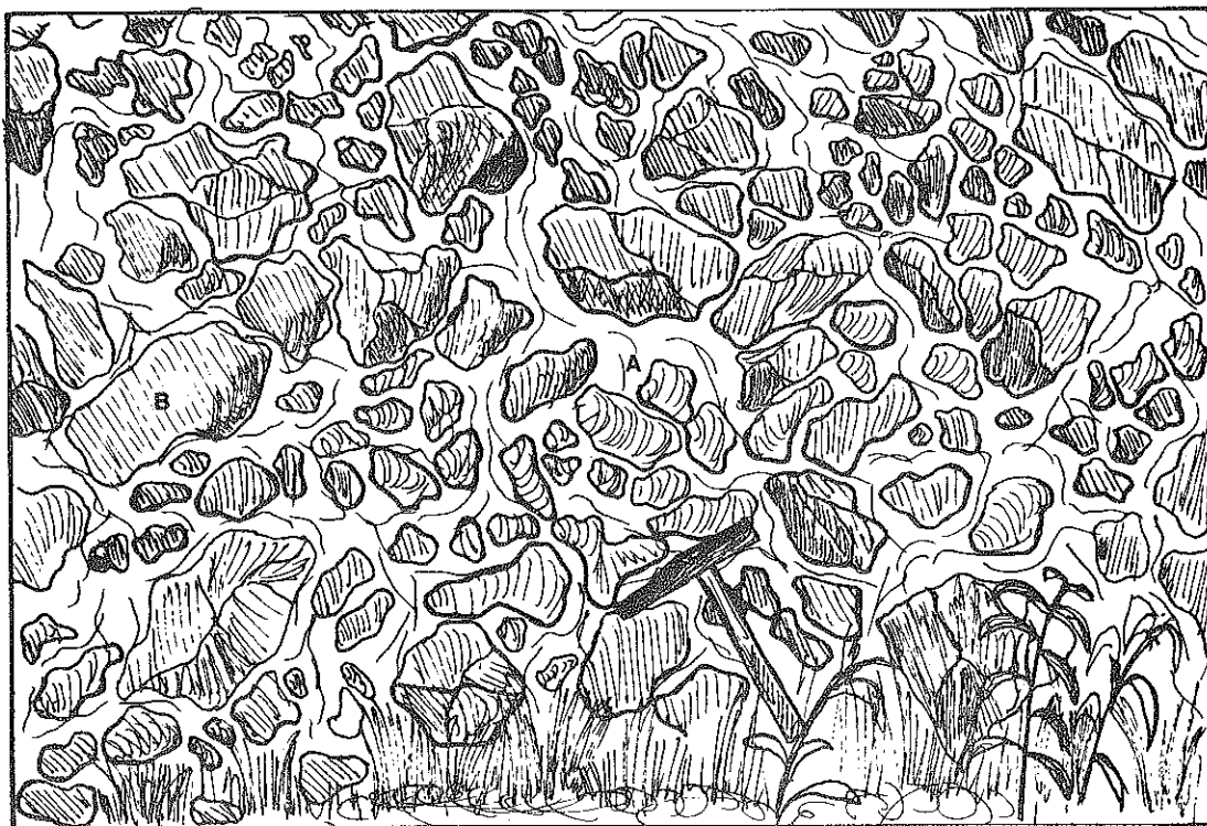
Fig. 25 : AFFLEUREMENT AU N.W. DE LA MAISON - RADA
