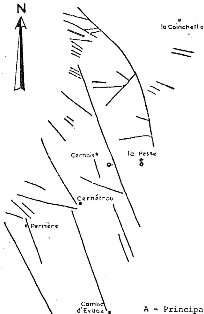
Fig. 57 - FRACTURATION AUX ABORDS DE LA GROTTTE EMERGENCE DU CERNOIS (ou du Grand - Cernois) JU 88 - Commune de la Pesse
