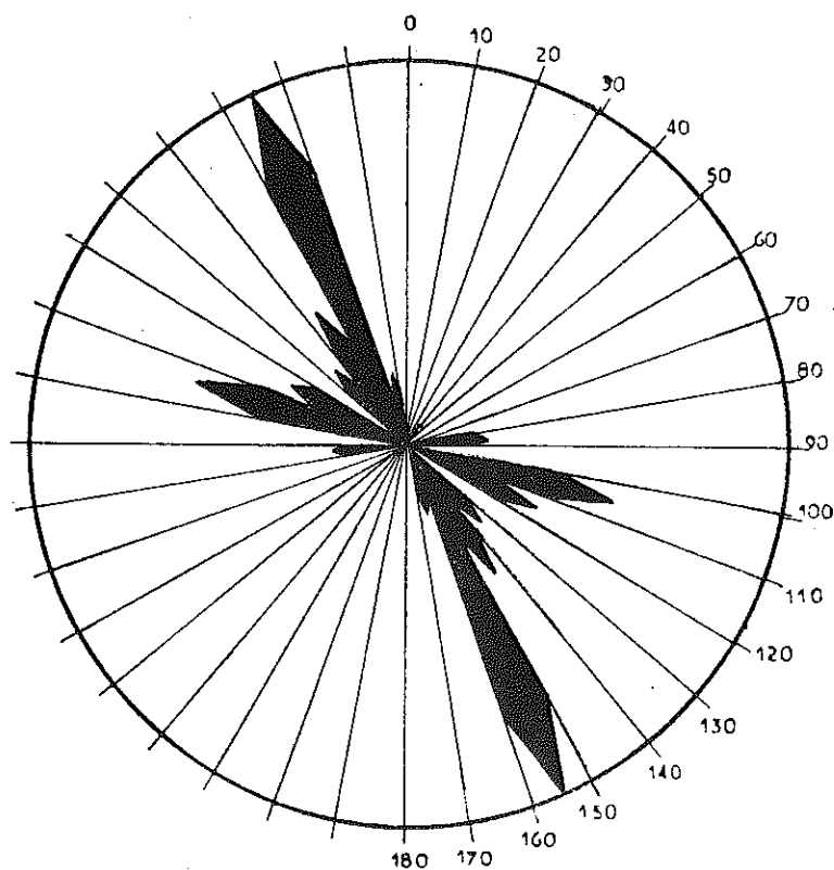
B - Rosace des directions de fractures visibles sur les photographies aériennes
