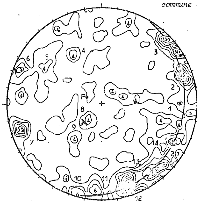
Fig. 56 : FRACTURATION AUX ABORDS DE LA GROTTÉ-ÉMERGENCE DU CERNOIS (ou du Grand-Cernois) JU 88 (XIII) commune de la Pesse
