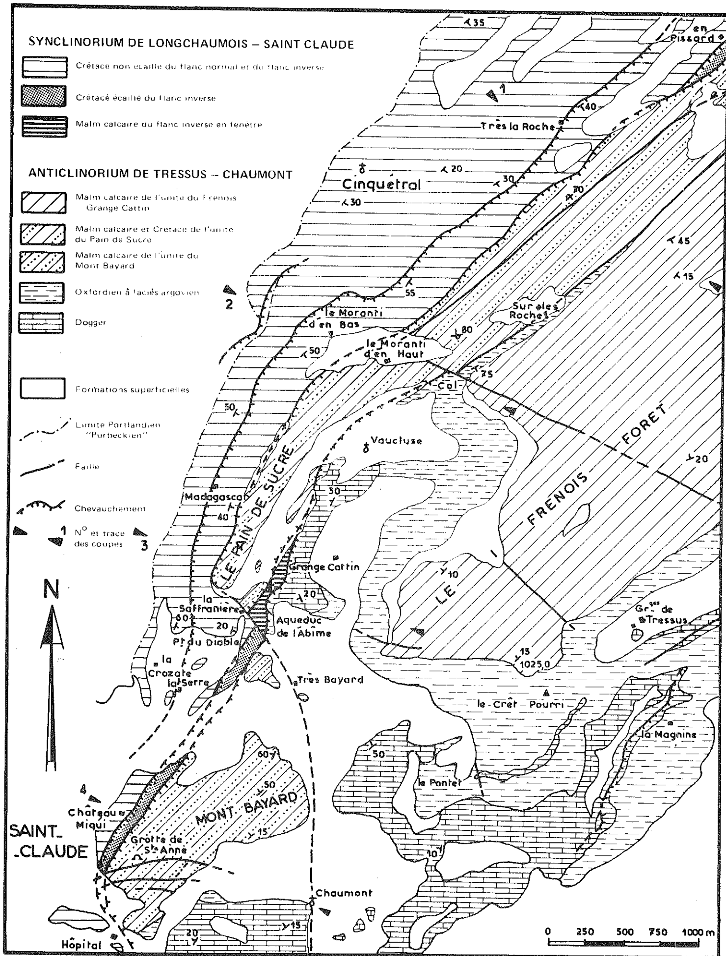
Fig. 33 : CHEVAUCEMENT DE SAINT - CLAUDE : SCHEMA STRUCTURAL
