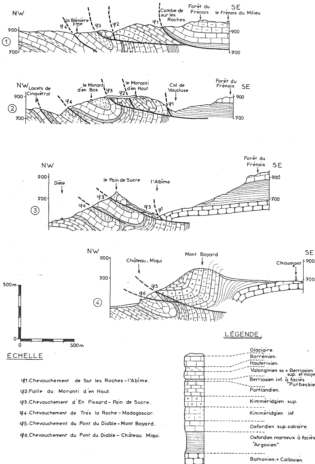
Fig. 34 : CHEVAUCHEMENT DE SAINT - CLAUDE : COUPES NW-SE
