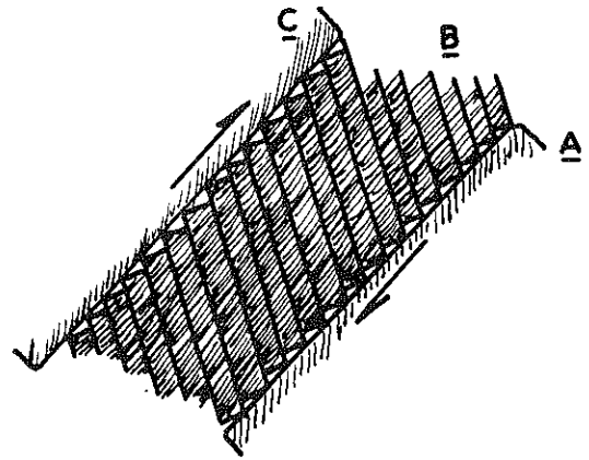
Fig. 48 : Interprétation des joints d'extension et des microlithons.
