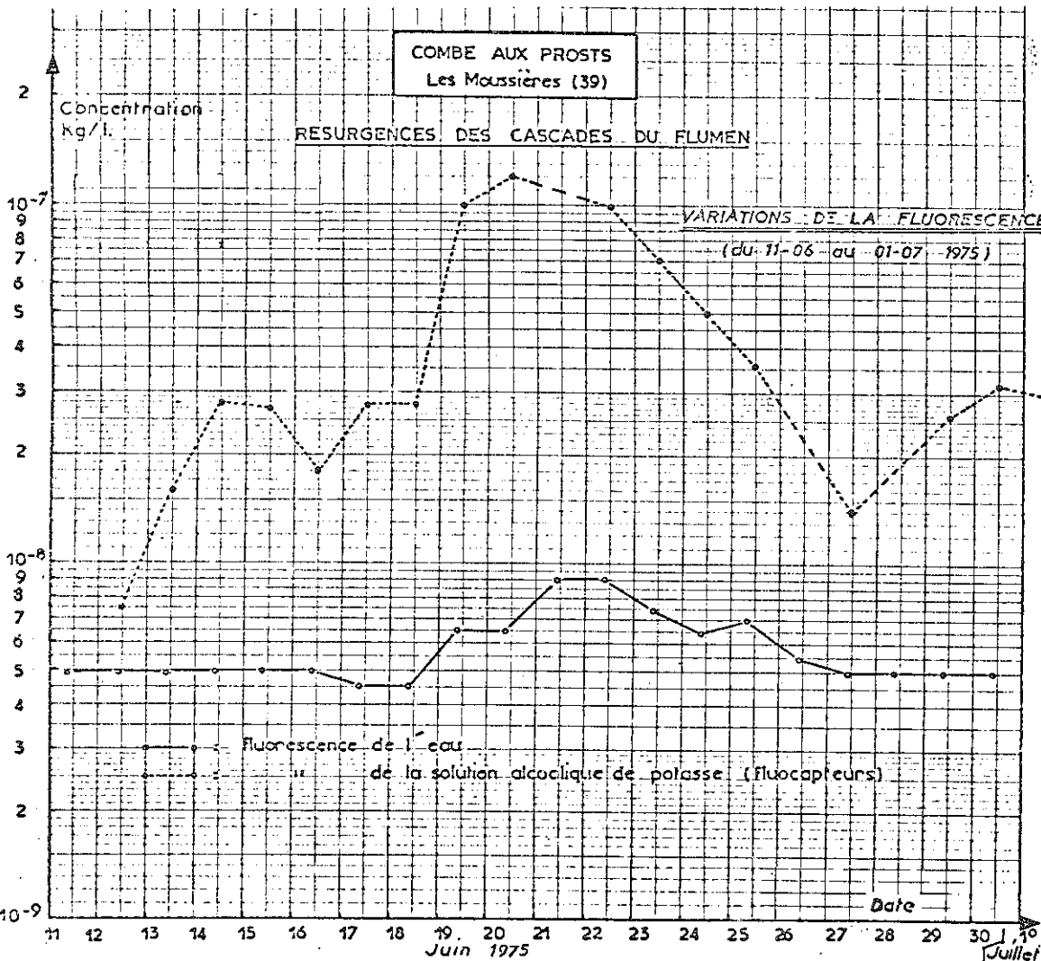
Fig.71 : ESSAIS DE TRACAGE 1975: RESTITUTION DE LA FLUORESCINE AUX CASCADES DU FLUMEN.
