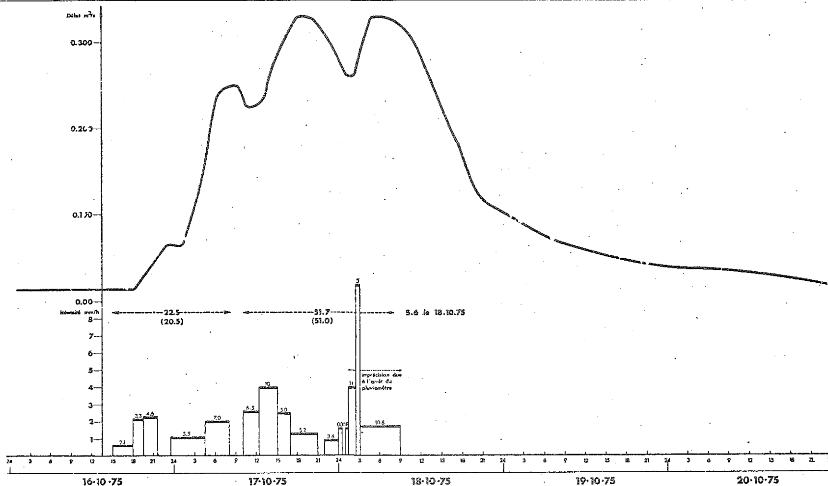
Fig. 80 : HYDROGRAMME DE CRUE - 16 au 20 OCTOBRE 1975
