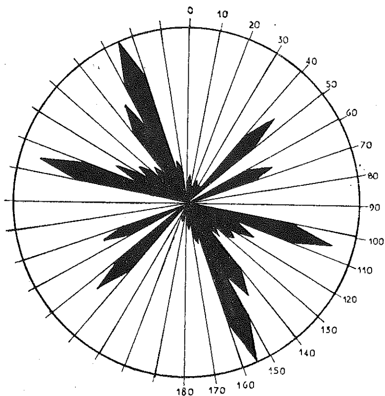
D - Rosace des directions de galeries de la Grotte-Exsurgence du Cernois (JU 88)
