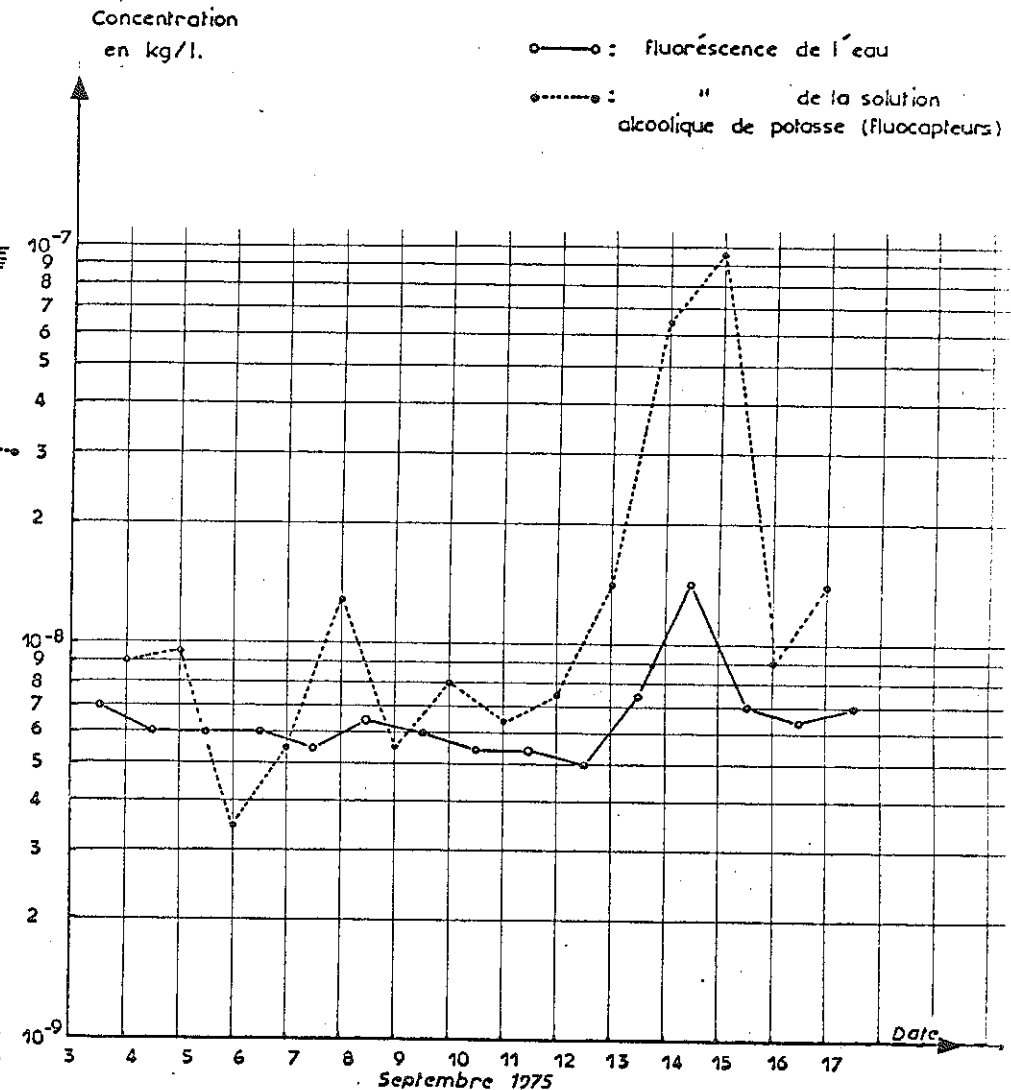
Fig.71 : ESSAIS DE TRACAGE 1975: RESTITUTION DE LA FLUORESCINE AUX CASCADES DU FLUMEN.
