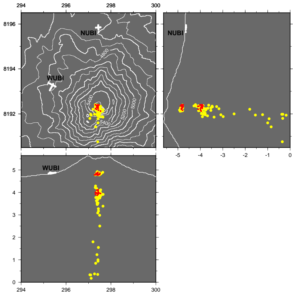
Figure 3: Carte de la topographie avec des localisation des sources à Ubinas 2009, rouge: des explosions vulcanienne et jaune: des longue période
