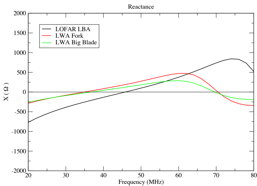
Fig 10. Antenna input impedance of the LOFAR LBA «string» antenna (black), LWA Fork antenna (red), LWA Big Blade «filled» antenna (green).
