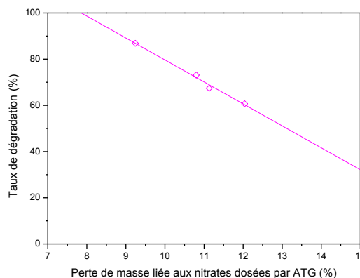
Figure 98. Evolution du taux de dégradation de \text{NH}_3 en fonction de la quantité de nitrate dosée par ATG sur le catalyseur FINNTI100 après test.
