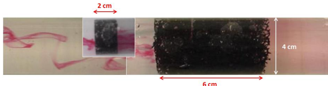
Figure 34. Illustration de l'effet de mélangeur statique en milieu liquide avec une mousse de polyuréthane (colorant : rouge amarante) 67 .
