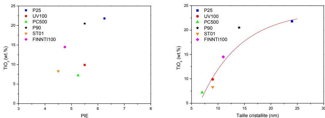
Figure 156. Teneur en \text{TiO}_2 des photocatalyseurs \text{TiO}_2/\beta\text{-SiC} (mousse 5400\ \mu\text{m} ), obtenus par imprégnation en voie humide ( 5\ \text{trempes } 100\text{g.L}^{-1} ) en fonction du PIE et de la taille de cristallite des \text{TiO}_2 commerciaux.
