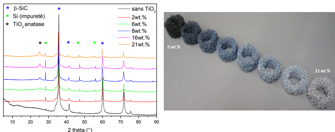
Figure 123. Diffractogrammes des rayons X (g.) et aspect (d.) des mousses de \beta -SiC à différentes teneurs en \text{TiO}_2 UV100.
