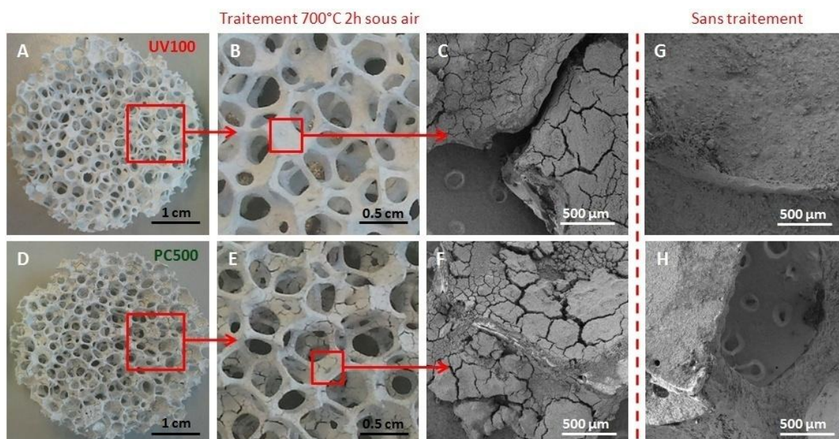
Figure 165. Aspect des revêtements de \text{TiO}_2 UV100 et PC500 sur mousse de \beta\text{-SiC} ( 5400\ \mu\text{m} ) avant (G-H) et après (A-F) traitement à 700^\circ\text{C} sous air durant 2h.
