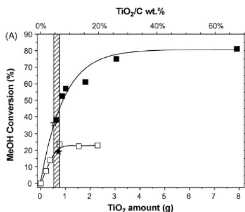
Figure 39. Conversion du méthanol en fonction de la quantité de \text{TiO}_2 pour un réacteur structuré avec des mousses de carbone ( \blacksquare ), avec du papier ALHSTROM ( \star ), avec le média QUARTZEL ( \star ), ou avec un dépôt sur ses parois ( \circ ) 70 .
