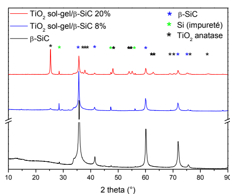
Figure 129. Diffractogramme des mousses de \beta -SiC avant et après imprégnation par du \text{TiO}_2 sol-gel.
