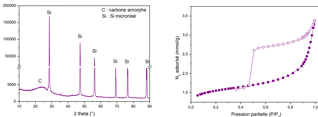
Figure 177. Diagramme de diffraction des rayons X et isotherme de désorption et d'adsorption d'azote des mousses de précurseurs de \beta -SiC.
