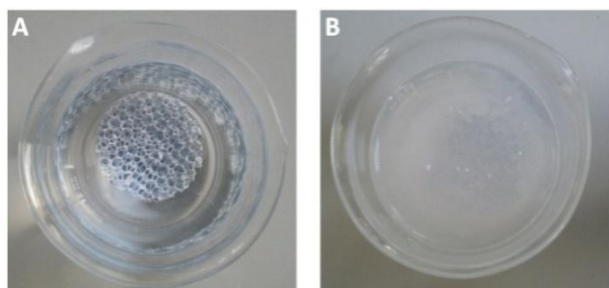
Figure 162. visualisation de la résistance à un lavage simple à l'eau d'une mousse de \text{TiO}_2/\beta\text{-SiC} ( 5400\mu\text{m} ), imprégnée de \text{TiO}_2 UV100 pour 2 méthodes d'imprégnation différentes : (A) avec rinçage entre chaque trempe (B) sans rinçage.
