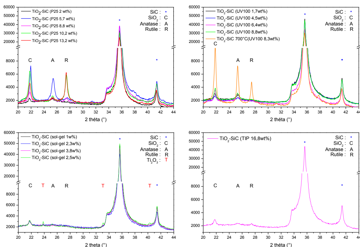
Figure 182. Diffractogrammes des mousses de \text{TiO}_2 - \beta -SiC en fonction de la teneur et de la source du précurseur de \text{TiO}_2 .
