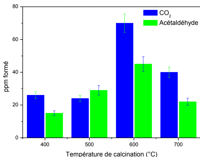
Figure 176. Concentrations de \text{CO}_2 et d'acétaldéhyde produites avec les mousses mixtes \text{TiO}_2(16\%)\text{-}\beta\text{-SiC} lors des tests de dégradation de la MEC, en fonction de la température de calcination des mousses de \text{TiC-}\beta\text{-SiC} sous air (6h).
