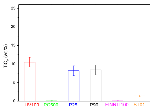
Figure 161. Teneur en \text{TiO}_2 des photocatalyseurs \text{TiO}_2/\beta\text{-SiC} (mousse 5400\mu\text{m} ), après 5 cycles d'imprégnation ( \text{TiO}_2 à 100\text{ g.L}^{-1} dans de l'éthanol), lavage et séchage, pour différentes poudres commerciales.
