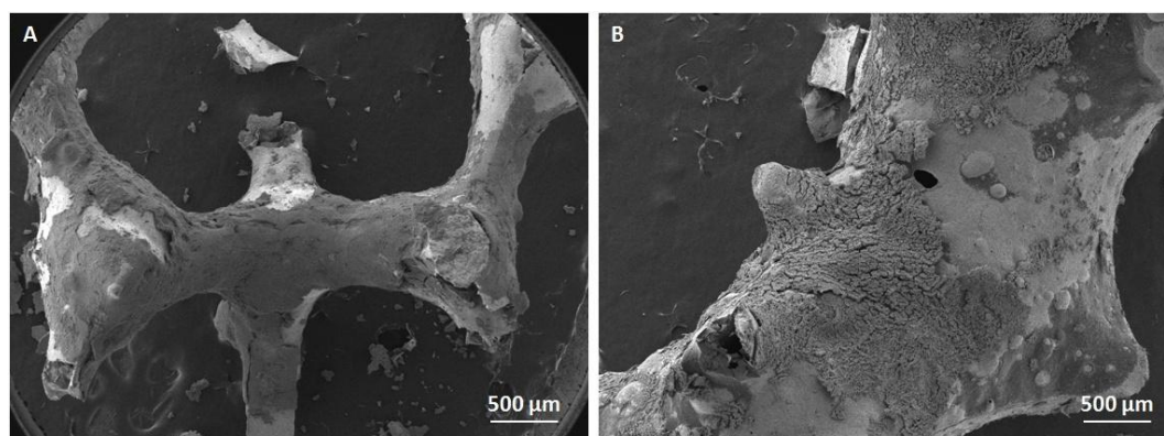
Figure 183. Clichés MEB d'une mousse (A) \text{TiC} - \beta -SiC avant oxydation et d'une mousse (B) \text{TiO}_2 - \beta -SiC (UV100 8,8%) après oxydation thermique à 500°C (2h).
