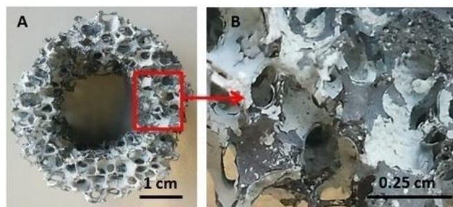
Figure 187. Mise en évidence du décrochage du revêtement de \text{TiO}_2 sur une mousse mixte à 8,3wt.% en UV100 initialement, calcinée à 700°C.
