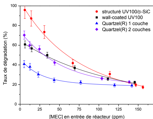
Figure 137. Comparaison des réacteurs en fonction de la concentration d'entrée, pour un débit d'air de 20 \text{ L.min}^{-1} .
