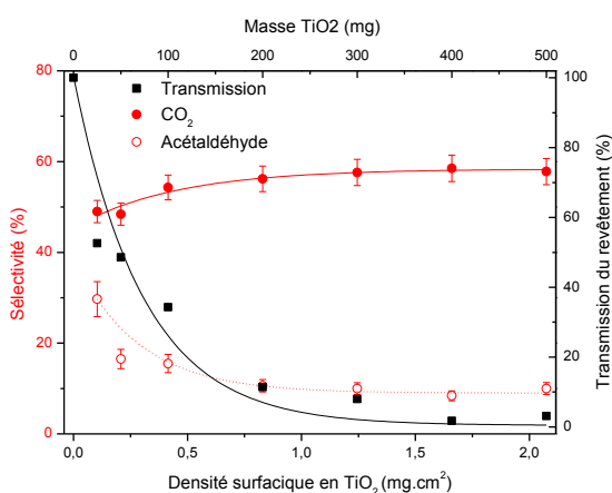
Figure 90. Evolution de la sélectivité en \text{CO}_2 (●) et en acétaldéhyde (○) et de la transmission des UV-A du revêtement photocatalytique (■) en fonction de la densité surfacique en \text{TiO}_2 UV100.
