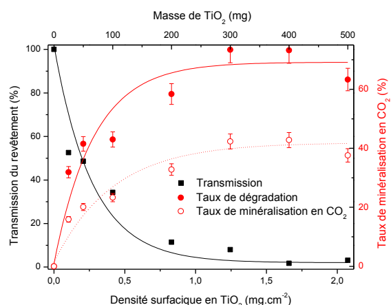
Figure 89. Evolution du taux de dégradation de la MEC (●), du taux de minéralisation en \text{CO}_2 (○) et de la transmission des UV-A du revêtement photocatalytique (■) en fonction de la densité surfacique en \text{TiO}_2 UV100.
