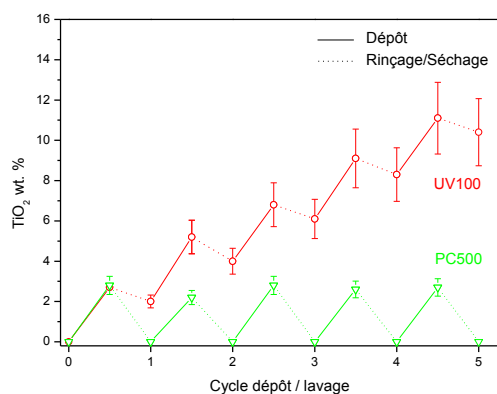
Figure 160. Evolution de la teneur en \text{TiO}_2 UV100 (○) et PC500 (Δ) des photocatalyseurs \text{TiO}_2/\beta -SiC (mousse 5400 \mu\text{m} ), en fonction du nombre d'imprégnation ( \text{TiO}_2 100 g.L -1 dans éthanol) et de rinçage/séchage.
