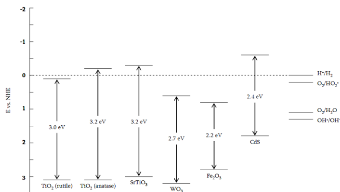
Figure 14. Schéma de la position des bandes de valence et de conduction de différents semi-conducteurs utilisés en photocatalyse 20 .
