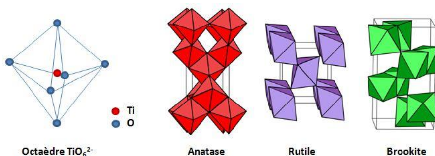
Figure 15. Schéma d'octaèdre TiO 6 2- , maille élémentaire de l'anatase, du rutile et de la brookite 21 .
