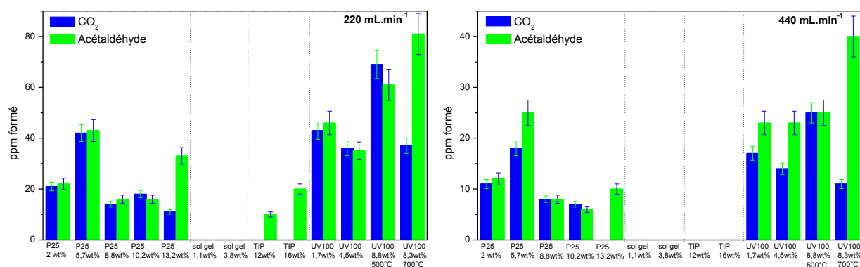
Figure 185. Concentrations de \text{CO}_2 et d'acétaldéhyde obtenues avec les mousses mixtes \text{TiO}_2 - \beta -SiC lors des tests de dégradation de la MEC en fonction de la nature et de la quantité du précurseur de \text{TiO}_2 , (g.) à 220 \text{ mL.min}^{-1} , (a) et 440 \text{ mL.min}^{-1} (b) en conditions standard.
