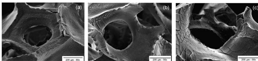
Figure 43. D p t de \text{TiO}_2   (a) 25 \text{g.L}^{-1} (b) 75 \text{g.L}^{-1} (c) 100 \text{g.L}^{-1} sur une mousse de \beta -SiC fournie par la soci t  SICAT 85 .
