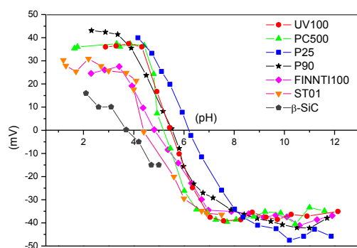
Figure 159. Mesure du point isoélectrique du \beta -SiC synthétisé par synthèse SMS ainsi que des \text{TiO}_2 UV100 ( \circ ), PC500 ( \Delta ), P25 ( \square ), P90 ( \star ), FINNT1100 ( \diamond ) et ST01 ( \nabla ).
