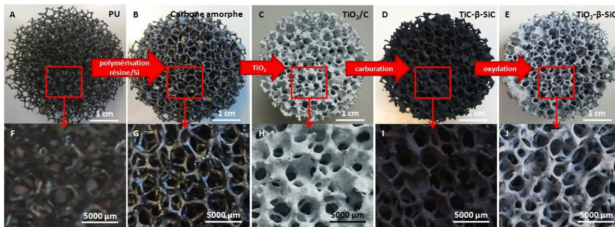
Figure 179. (A) Mousse de polyuréthane, (B) précurseur de \beta -SiC, (C) après imprégnation de \text{TiO}_2 (UV100 8,8%), (D) après carburation (mousse de \text{TiC-}\beta\text{-SiC} ), (E) après oxydation (mousse de \text{TiO}_2 - \beta -SiC).
