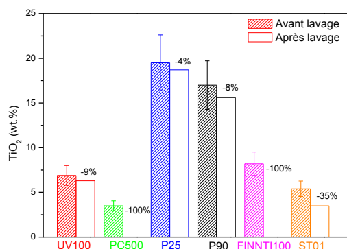
Figure 164. Teneur en \text{TiO}_2 des photocatalyseurs \text{TiO}_2/\beta\text{-SiC} (mousse 5400\ \mu\text{m} ) obtenus par imprégnation en voie humide ( 5\ \text{trempes } 100\text{g.L}^{-1} dans éthanol pur), sans rinçage et traités à 700^\circ\text{C} , avant et après lavage à l'eau. Le pourcentage de perte au lavage est précisé sur l'histogramme de chaque \text{TiO}_2 commercial.
