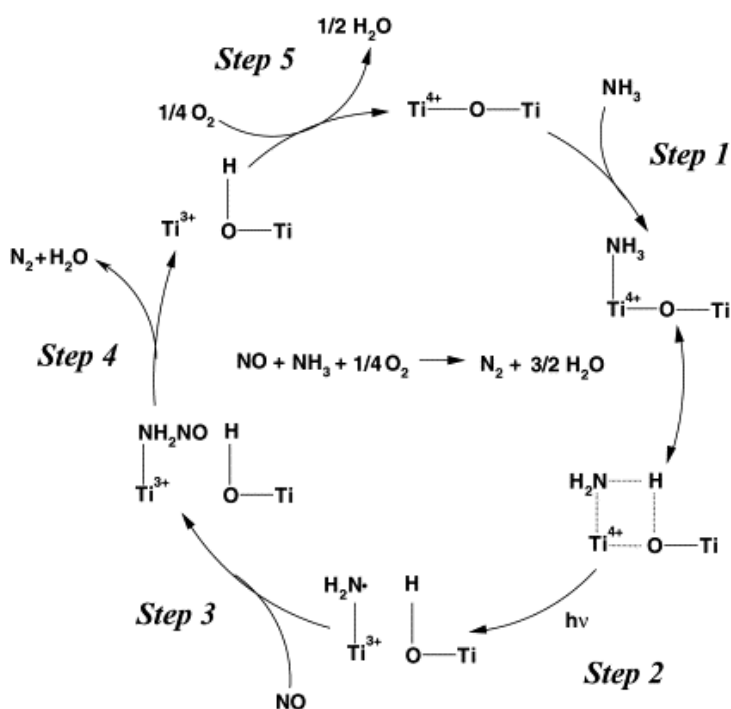
Figure 54. Mécanisme de dégradation photocatalytique de \text{NH}_3 en présence de \text{NO} (SCR : Selective Catalytic Reduction par \text{NH}_3 ), proposé par Teramura et al. 124 .
