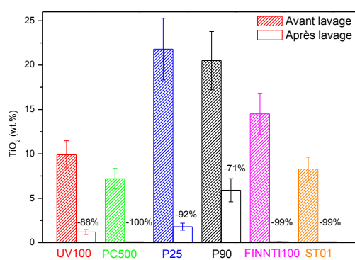
Figure 155. (g.) Teneur en \text{TiO}_2 des photocatalyseurs \text{TiO}_2/\beta -SiC (mousse 5400 \mu\text{m} ), obtenus par imprégnation en voie humide (5 trempes 100 \text{ g.L}^{-1} ), avant et après lavage pour les différentes poudres commerciales étudiées. Le pourcentage de perte au lavage est précisé sur l'histogramme de chaque \text{TiO}_2 commercial. (d.) Rappel du point isoélectrique et de la taille de cristallite des poudres commerciales.
