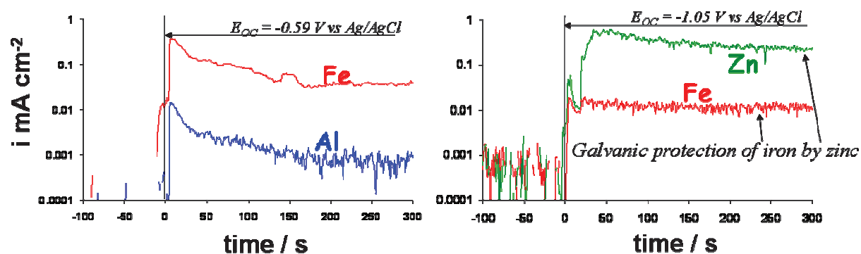
Figure 1. La corrosion spontanée des systèmes avec les peintures contenant les pigments d'Al (gauche) et de Zn (droite) dans un liant organique.
