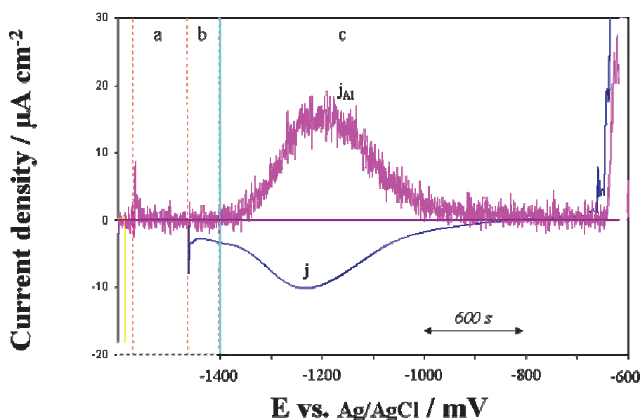
Figure 3. La réactivité (courant électrochimique, j , et dissolution d'Al, j_{\text{Al}} ) en 3% NaCl (pH 6.1) : (a) – la réaction spontanée, (b) – potentielle appliquée (-1.4 V), (c) – courbe de polarisation cathodique.
