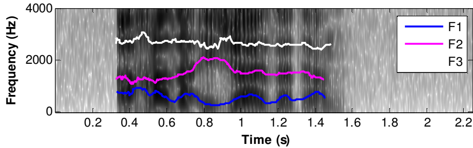
Figure 1. 2 : Représentation des trois premiers formants (F1, F2 et F3) superposés sur le spectrogramme du signal « أَخَذَ إِجَازَةً. ” 3axaḍa 3ija:zatan ” « Il a pris des vacances » : où il y a une alternance de sons voisés et non voisés. Dans le cas voisé, une structure formantique est présentée.
