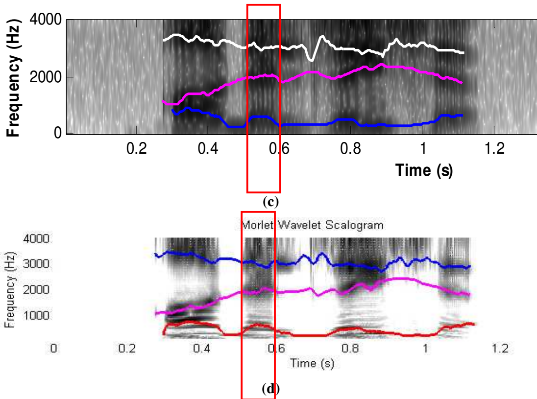
Figure 5.7 : Trajectoires formantiques estimées du signal sonore «قَادَ الْجَيْشِ ا» « qa:da ljaysa » prononcée par la locutrice W4 (a) Etiquetage formantique manuel de référence, (b) Trajectoires formantiques estimées utilisant Praat (c) Trajectoires formantiques estimées utilisant les crêtes de Fourier et (d) Trajectoires formantiques estimées utilisant les crêtes d'ondelette cmor10-1
