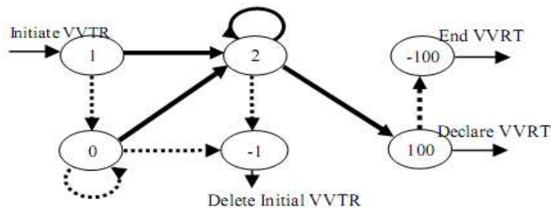
Figure 2. 17 : Schéma expliquant les différents stades de la phase de décisions début/fin des trajectoires VVTR
