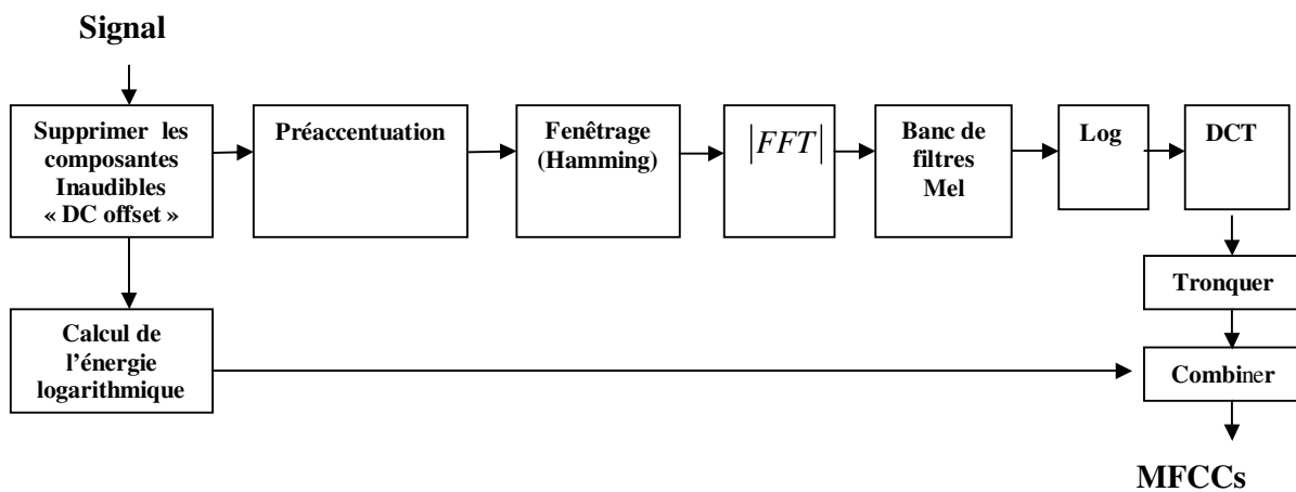
Figure 2. 13 : Schéma détaillé de l'extraction des vecteurs MFCC selon la norme standard de « ETSI Aurora » (Darch.J 2005)
