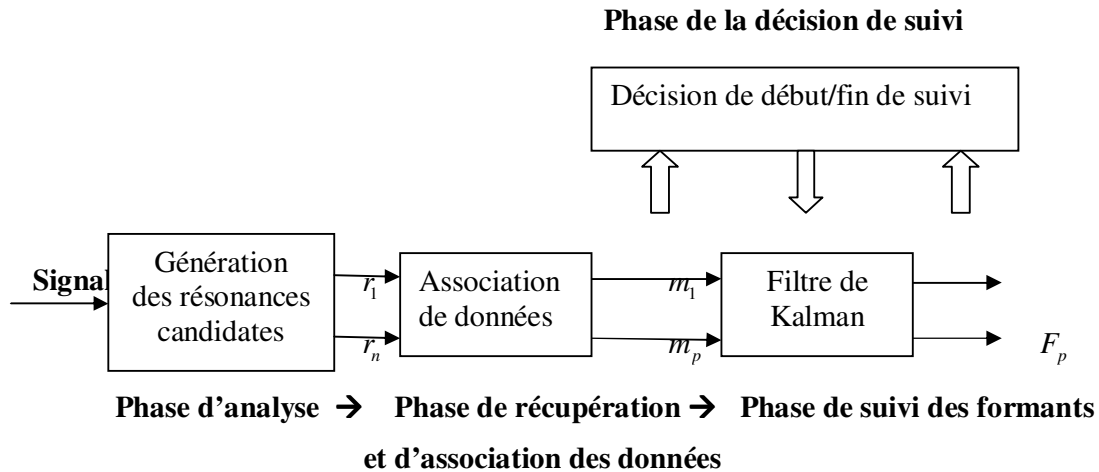
Figure 2. 16 : Schéma global de l'algorithme de suivi de formants proposé par (Özbek.Y.I 2006)
