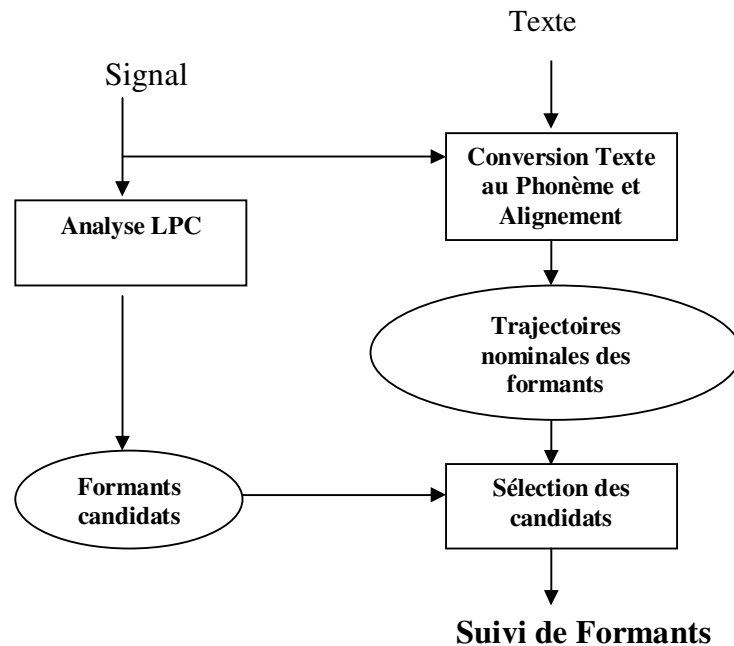
Figure 2. 11 : Schéma global de l'algorithme de suivi de formants proposé par (Lee.M 2005)
