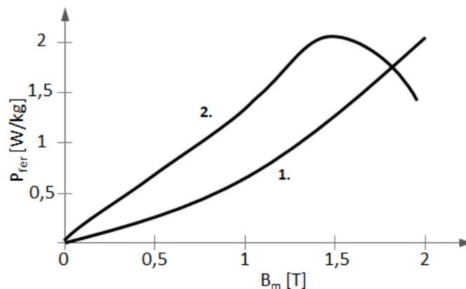
Figure 1.10 Pertes magnétiques 1) en champ unidirectionnel et 2) en champ tournant
