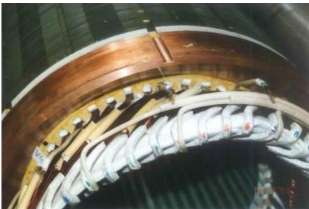
a) Têtes des bobines statoriques
