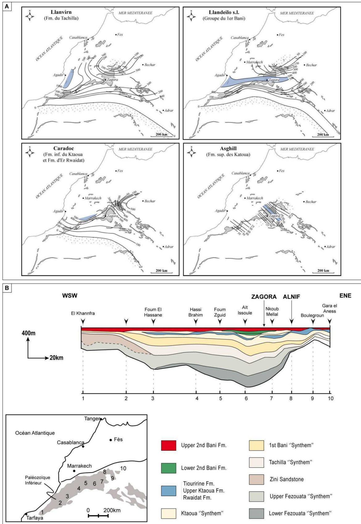
Figure 3.11 : A) Carte des isopaques à l'Ordovicien supérieur dans l'Anti-Atlas et le chaînon de l'Ougarta. La région se Zagora se caractérise par une subsidence très marquée à l'Asghill (D'après Destombes et al., 1985, in Marante, 2008). B) Coupe transversale à travers l'Anti-Atlas illustrant la géométrie des dépôts ordoviciens contrôlée par la subsidence à l'aplomb de la suture panafricaine (D'après Destombes et al., 1985 ; Hamoumi, 1999).
