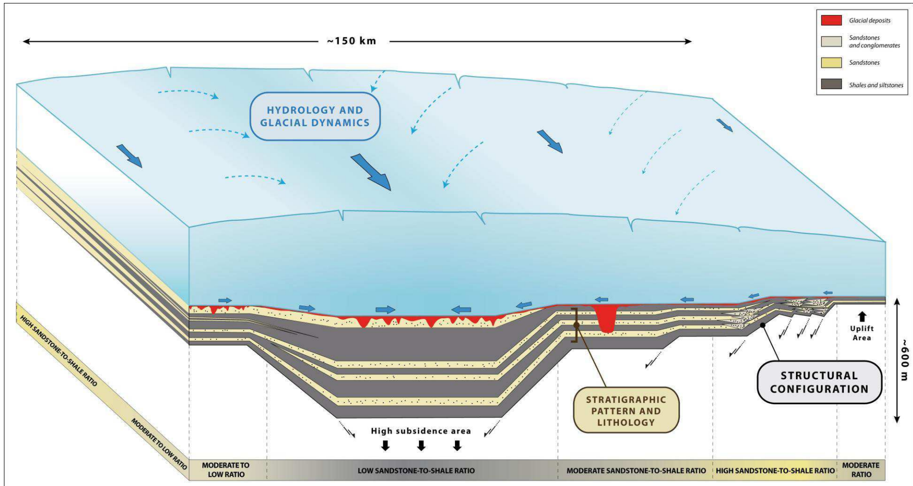
Figure 4.12 : Modèle de distribution des vallées tunnel. La densité et la morphologie des vallées tunnel sont directement contrôlées par (1) la lithologie du préglaciaire (ratio argiles/grès) et (2) la dynamique glaciaire et les flux d'eau de fonte à la base de la calotte. Ces deux paramètres sont sous le contrôle direct de la structuration du bassin, et donc de l'héritage structural.
