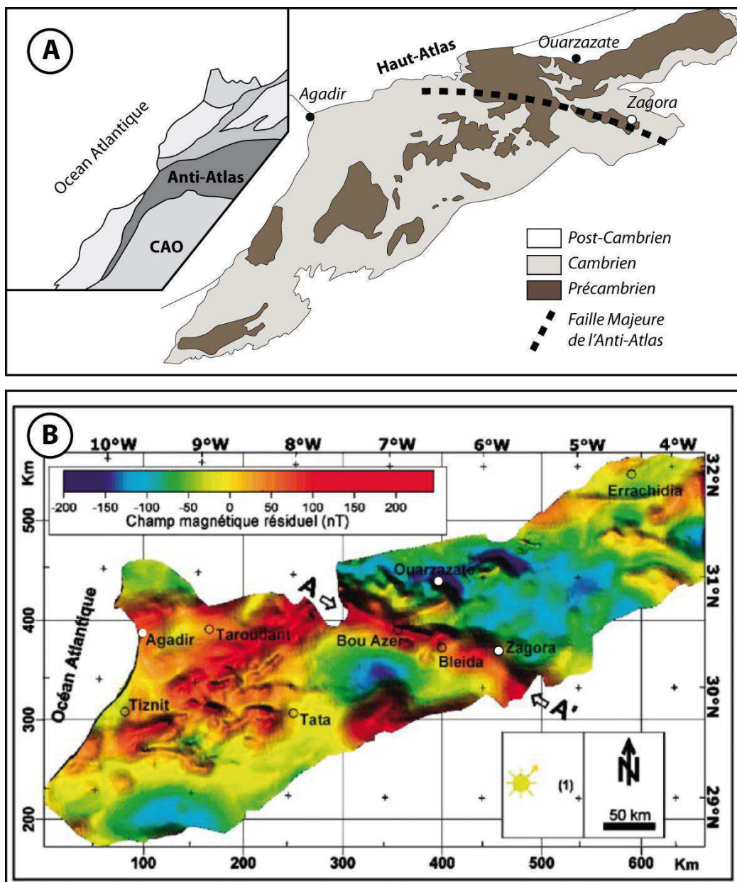
Figure 4.2 : A) Carte géologique simplifiée de l'Anti-Atlas, illustrant les « boutonnières » précambriennes, les séries cambriennes et la position de la faille majeure de l'Anti-Atlas B) Cartographie du champ magnétique résiduel de l'Anti-Atlas. Les fortes valeurs observées sur l'axe A-A' entre Zagora et Bou Azer, correspondent à l'anomalie magnétique associée à la faille majeure de l'Anti-Atlas, héritée de l'orogénèse panafricaine (Modifié d'après Soulaïmani et al., 2006)
