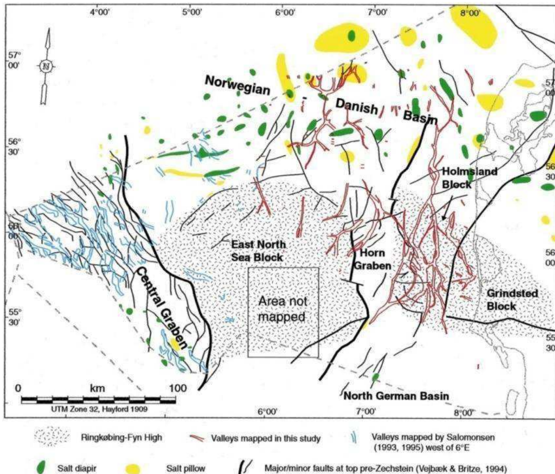
Figure 1.29 : Cartographie des vallées tunnel, des structures salifères et des principaux accidents structuraux en Mer du Nord (d'après Vejbaek & Britze, 1994 , in Huuse & Lykke-Andersen, 2000 )
