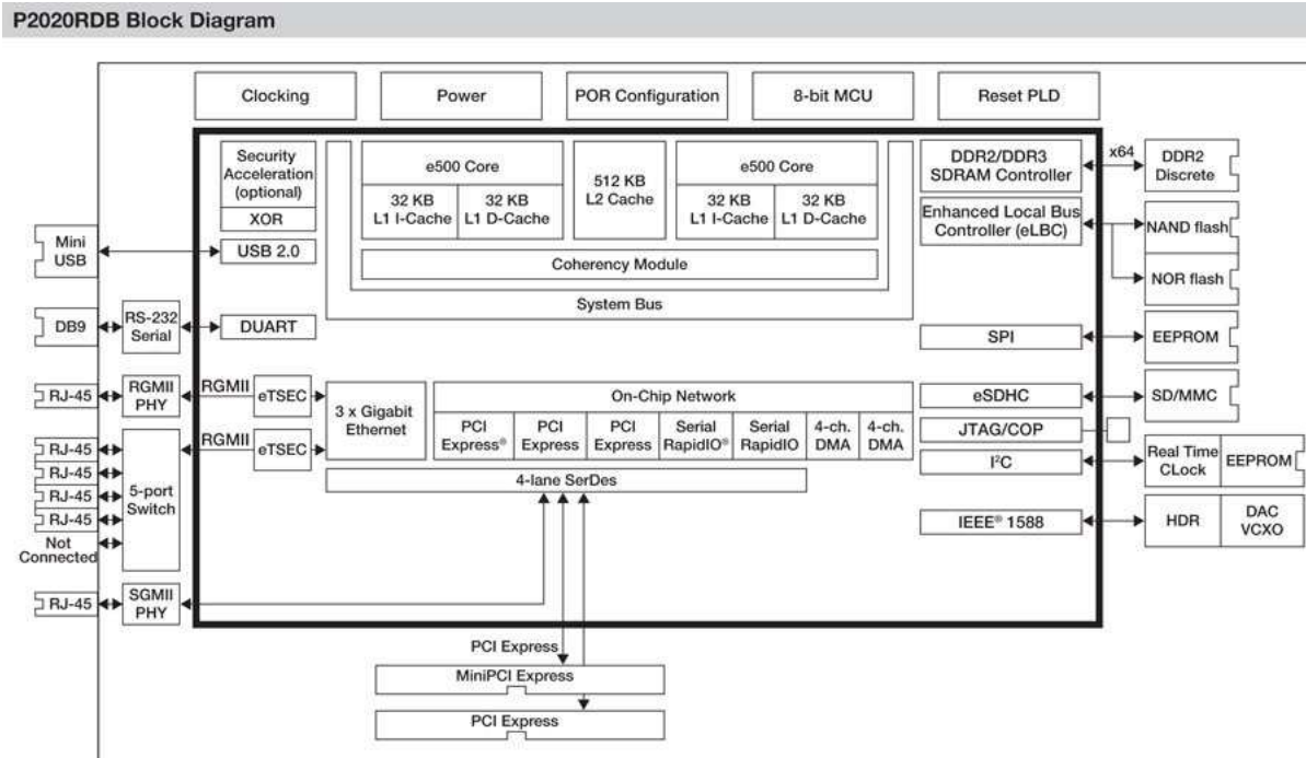
FIGURE 5.3: Schéma bloc du QorIQ P2020
