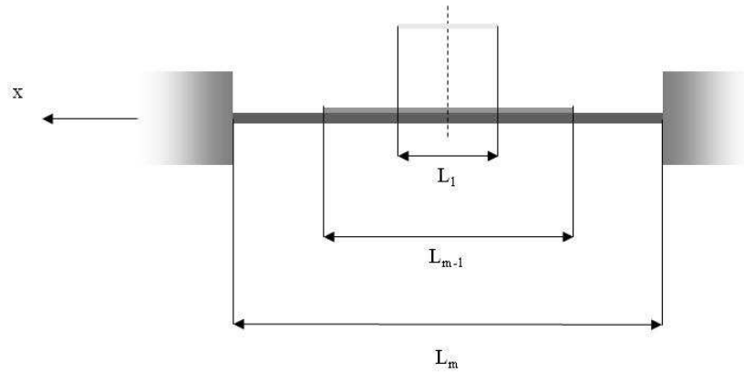
Figure 2.33 Vue de coté d'une poutre multicouche avec des longueurs de couche différentes
