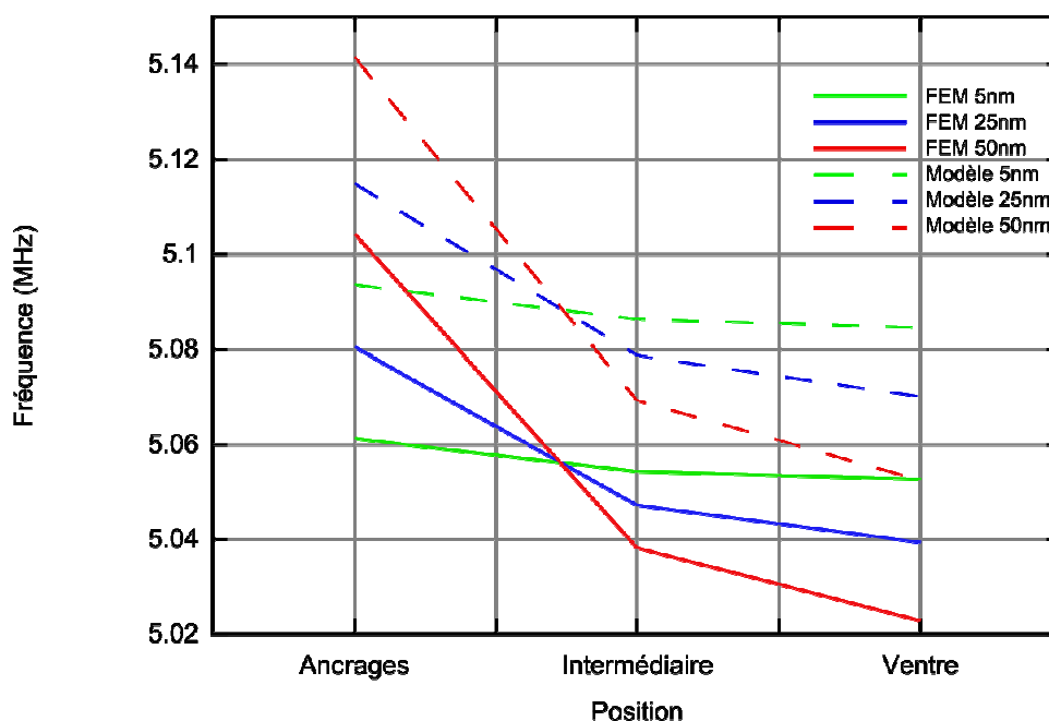
Figure 2.41 Comparaison du modèle et des simulations pour une correction localisée en différents lieux pour plusieurs épaisseurs de matériau ajouté ( L=20\mu m , W=1.5\mu m , Longueur patch = 2x9\mu m )
