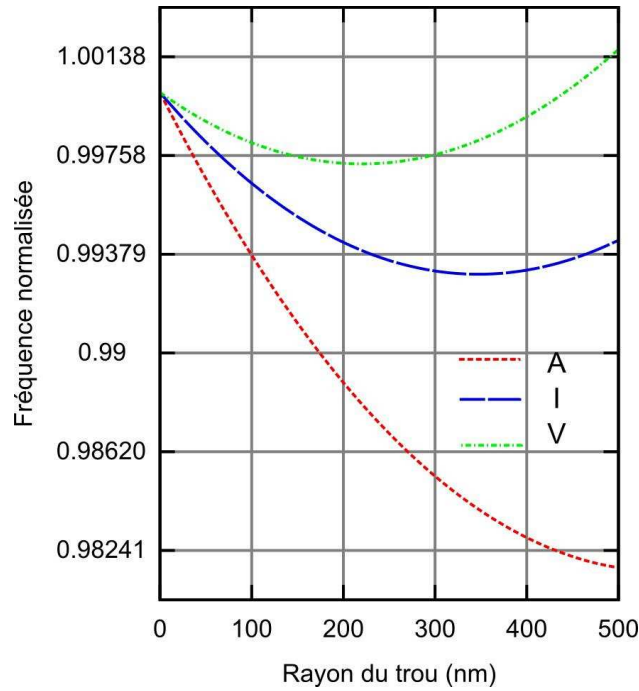
Figure 2.23 Variation de la fréquence fonction de la taille d'un trou pour les 3 zones (« V » = 25\mu m , « I » = 10\mu m , « A » = 5\mu m )
