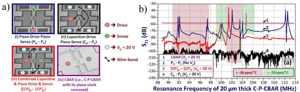
Figure 1.5 Combinaison des transductions capacitives et piézoélectriques (a), mesures électriques des différentes combinaisons sur un même dispositif (b)
