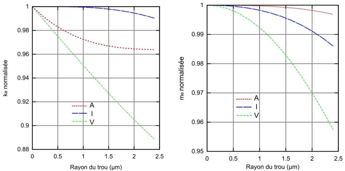
Figure 2.5 Variation de la raideur et de la masse effectives en fonction de la taille d'un trou pour les 3 zones (« V » = 25µm, « I » = 10µm, « A » = 5µm, f_i = 4.9192\text{MHz} )
