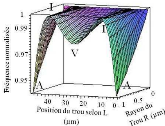
Figure 2.3 Variation de la fréquence de résonance en fonction du rayon d'un trou et de la position de ce dernier ( L = 50 \mu\text{m} , W = 20 \mu\text{m} , h = 1.4 \mu\text{m} , f_i = 4.9192 \text{ MHz} )
