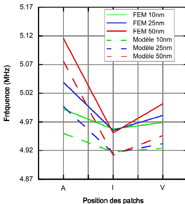
Figure 2.40 Comparaison des simulations et du modèle dans le cadre de la correction localisée ( A, I, V : patches\ 2x9x20\mu m^2 ) pour plusieurs épaisseurs
