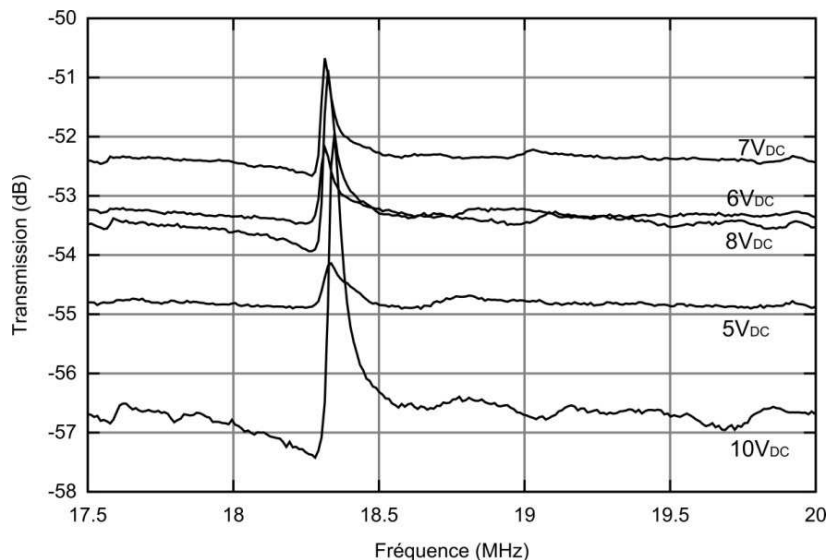
Figure 4.24 Mesure électrique d'une plaque fonction de la tension V_{DC}
