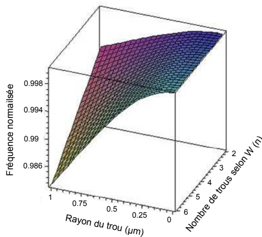
Figure 2.14 Variation de la fréquence en fonction du nombre de trous suivant la largeur ( n ) et du rayon d'un trou ( m=4, a_m=2,5\mu m, f_i = 4.9192MHz )
