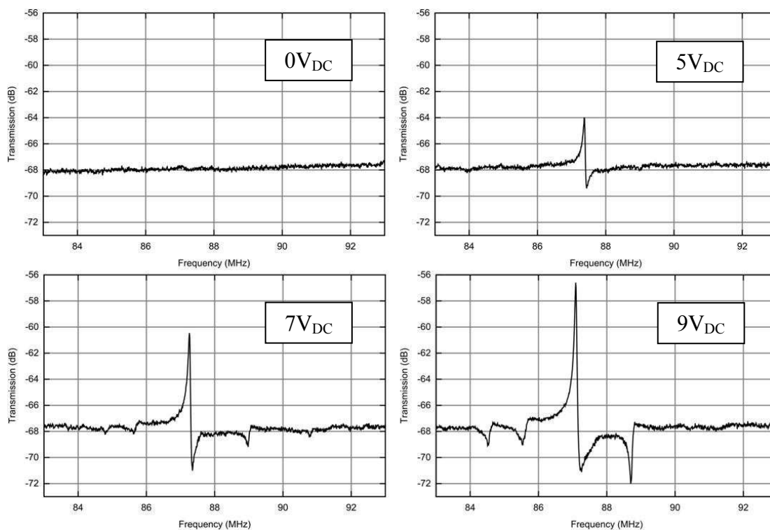
Figure 4.25 Mesure électrique d'un disque pour différentes valeurs de V_{\text{DC}}
