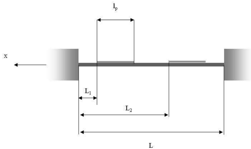
Figure 2.34 Correction à deux patches (vue de coté)
