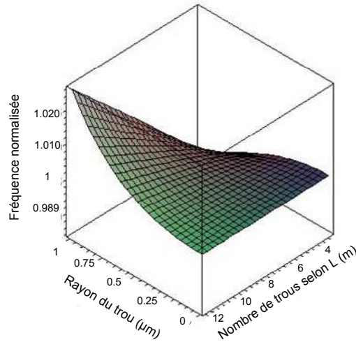
Figure 2.13 Variation de la fréquence en fonction du nombre de trous suivant la longueur ( m ) et du rayon d'un trou ( n=4, f_i = 4.9192MHz )
