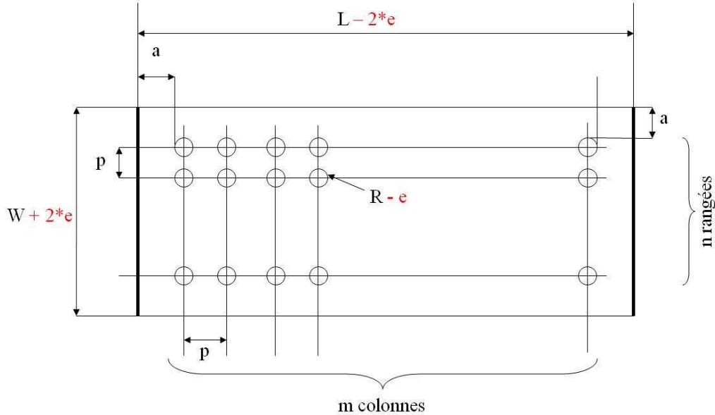
Figure 2.35 Schéma d'une poutre pour correction par épitaxie
