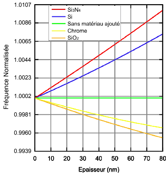
Figure 2.36 Variation de la fréquence d'une poutre pourvu d'un patch en position "V" en fonction de l'épaisseur et de la nature de ce dernier ( f_i = 4.9192MHz )
