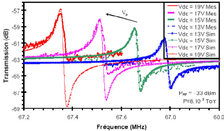
Figure 1.36 Réponse fréquentielle d'une poutre bi-encastée pour différentes tensions de polarisation (expérimentales et simulations) [69]
