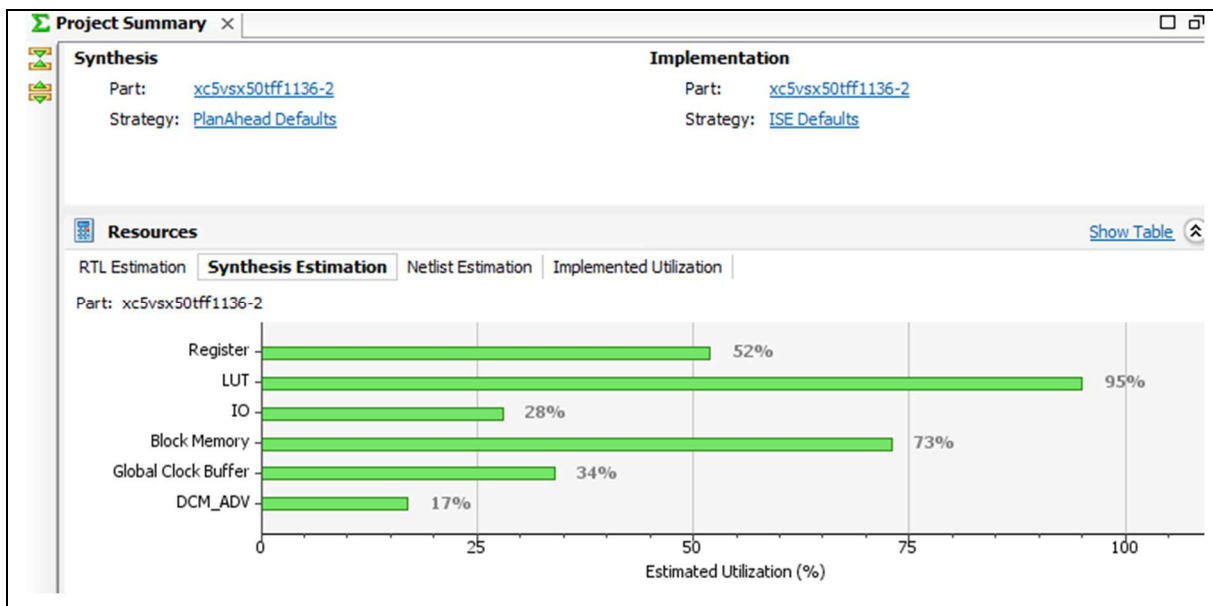
Figure 5-17 : Rapport de synthèse pour FPGA xc5vsx50t
