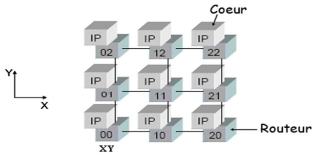
Figure 4-1 : Topologie maillée 2D du NoC Hermes.
