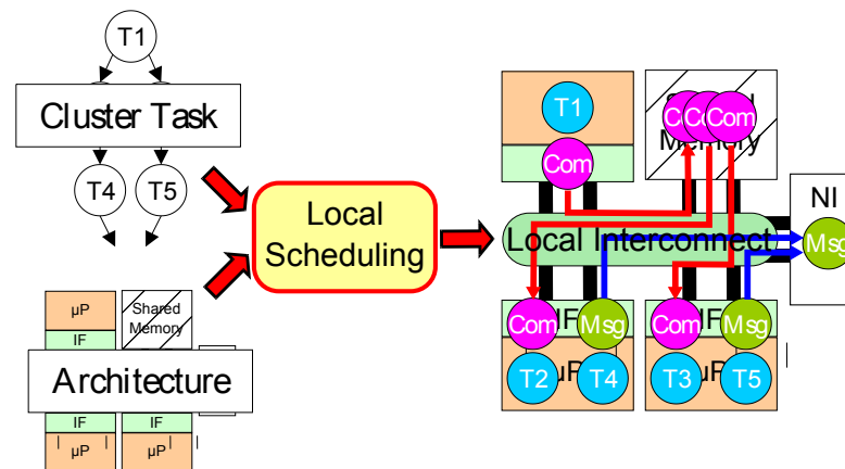
Figure 3.3 – Exemple d'ordonnancement de TC1 localement à un cluster
