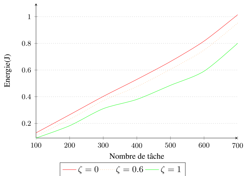
Figure 9.3 – Energie consommée vs. charge de travail (en nombre de tâche), pour différents facteurs de relaxation, suivant le scénario de variabilité sc.2
