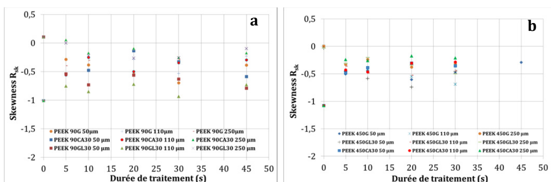
Figure II. 41. Evolution de la Skewness en fonction des conditions du traitement. a) PEEK 90G et ses composites et b) PEEK 450G et ses composites.
