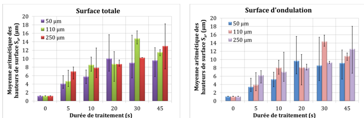
Figure II. 49. Evolution des paramètres ( S_a ) en fonction des conditions de traitement (durée de traitement et taille moyenne des particules) : a) surface brute et b) surface d'ondulation. PEEK APC2/AS4.
