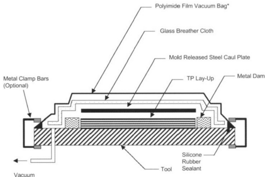
Figure I. 12. Schéma de principe (échelle non respectée) d'un assemblage drapé type sous bâche à vide (Campbell 2004).
