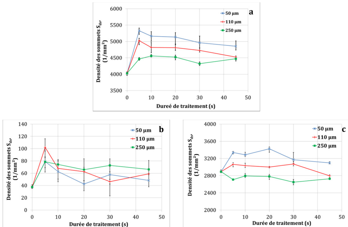
Figure II. 53. Evolution du paramètre ( S_{ds} ) en fonction des conditions de traitement (durée de traitement et taille moyenne des particules) : a) surface brute, b) surface d'ondulation et c) surface de microrugosité. PEEK APC2/AS4.
