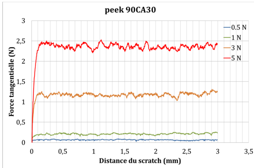
Figure I. 59. Variation de la force tangentielle ( F_t ) en fonction de la force normale ( F_n ) appliquée et la distance du rayage.
