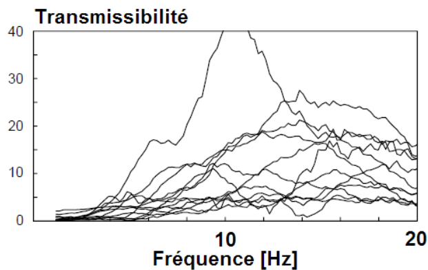
Figure 2.3 La masse apparente (le module [Kg]) et la transmissibilité du siège (le module [rad/s 2 /m/s 2 ]) vers le bassin, posture dénommée stricte. Adaptée de [MG 02b].
