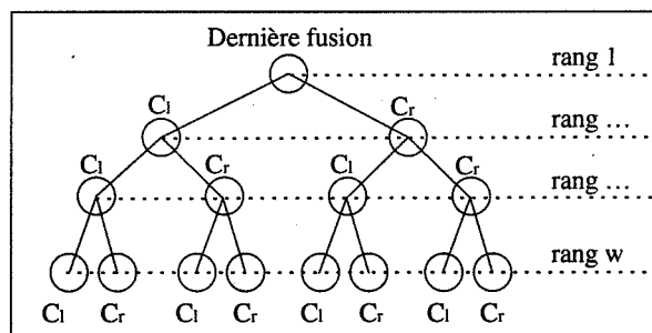
Figure IV.42 : Arbre de fusion d'un ensemble de 2^w chaînes initiales.
