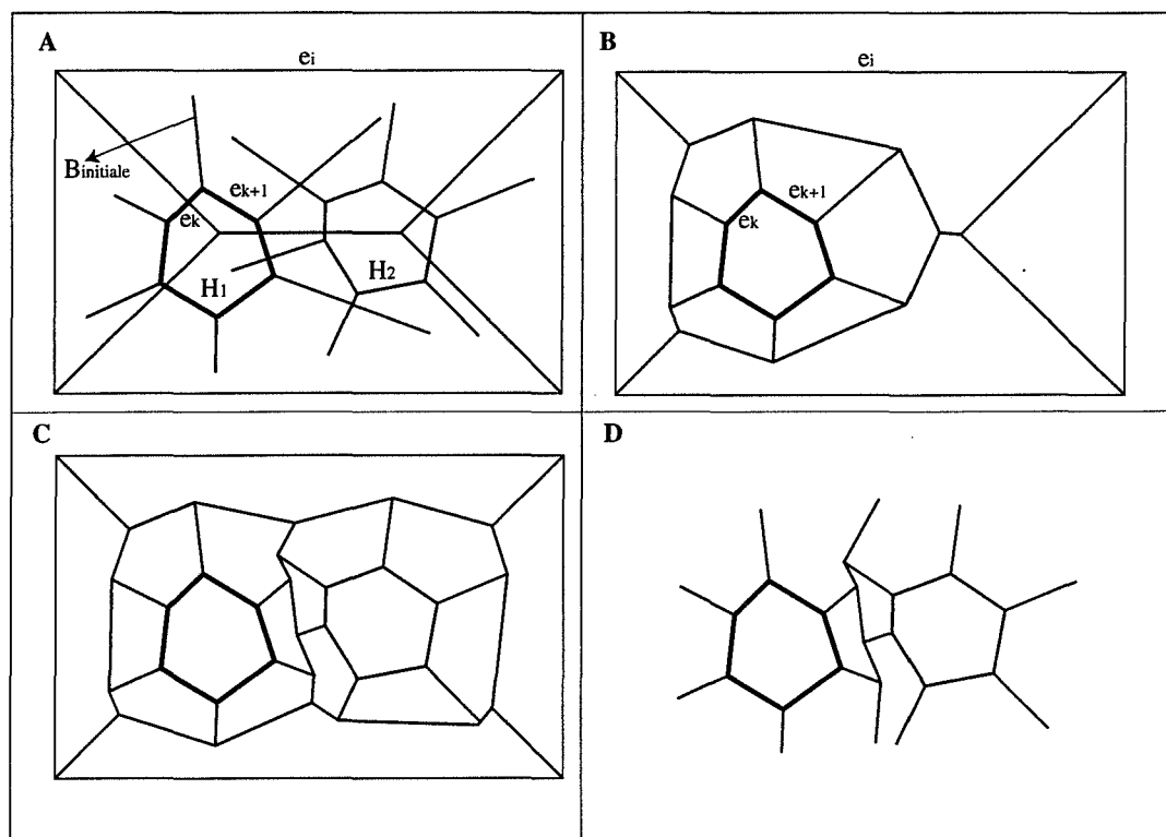
Figure IV.50 : Simplification de la procédure de construction d'un réseau bissecteur externe par ajout d'un contour externe situé à l'infini. (Pour les besoins de l'illustration le rectangle choisi est trop petit. Ainsi, il ne permet pas de déterminer le réseau bissecteur complet.)
