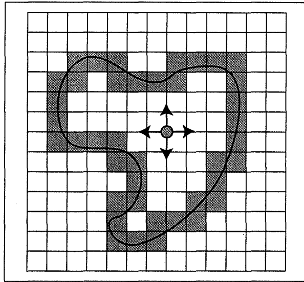
Figure II.33 : La détermination des nœuds situés à l'intérieur des contours permet de prendre en compte l'information topologique associée à la section de l'objet.
