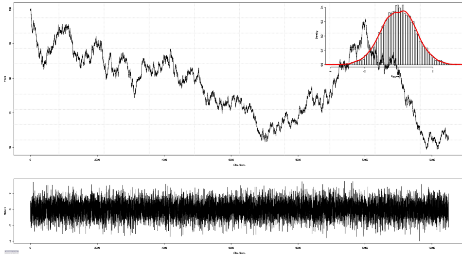
Fig. 3.14: Pseudo-chronique financière engendrée par la séquence des décimales de \pi . En haut les cours, en haut à droite, la distribution des pseudo-rentabilités, en bas leur chronique.
