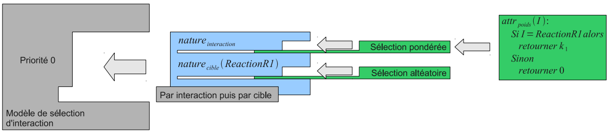
(a) Politique de sélection équivalente à l'unité de sélection décrite dans l'algorithme 13(a) de la page 206.
