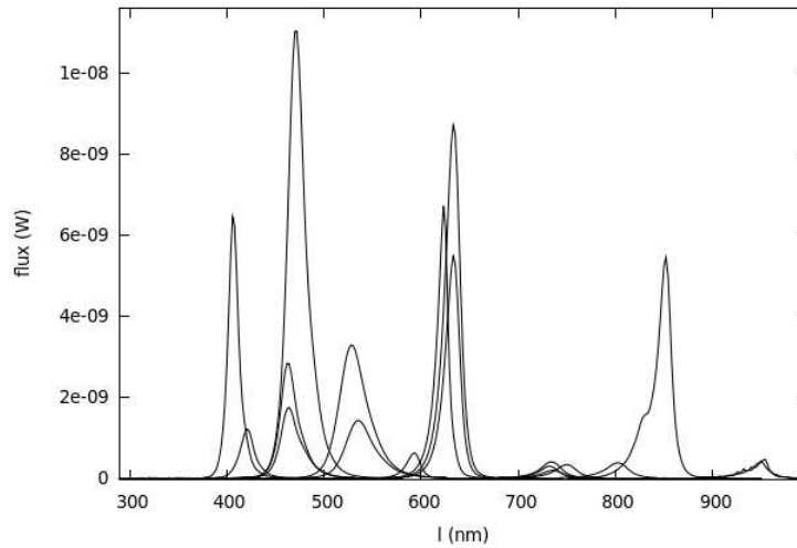
Fig. 4.7.: Les spectres d'émission des LEDs choisies pour SNDice. Les mesures ont été effectuées à température ambiante et au courant d'alimentation nominal. Les flux ont été normalisés, ce qui permet de vérifier les intensités relatives des faisceaux. Ainsi il est possible remarquer que les LEDs ultraviolettes et les LEDs rouges à basse puissance (Marubeni) fournissent un flux plus faibles de 1-2 ordre de grandeur par rapport à la LED la plus puissante.
