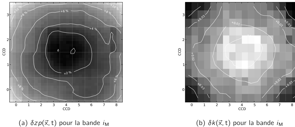
Fig. 3.15.: Exemple des cartes des corrections \delta zp(\vec{x}, t) et \delta k(\vec{x}, t) pour la bande i_M obtenues à partir de la grille photométrique observée en 2005. La carte (a) montre que la mesure du flux d'une étoile peut varier jusqu'à 12% entre le centre et les coins de la caméra. Les variations en (b) reproduisent le motif radial déjà mis en évidence par l'entreprise constructrice des filtres 3.2.2. Extraits de (Regnault et al., 2009).
