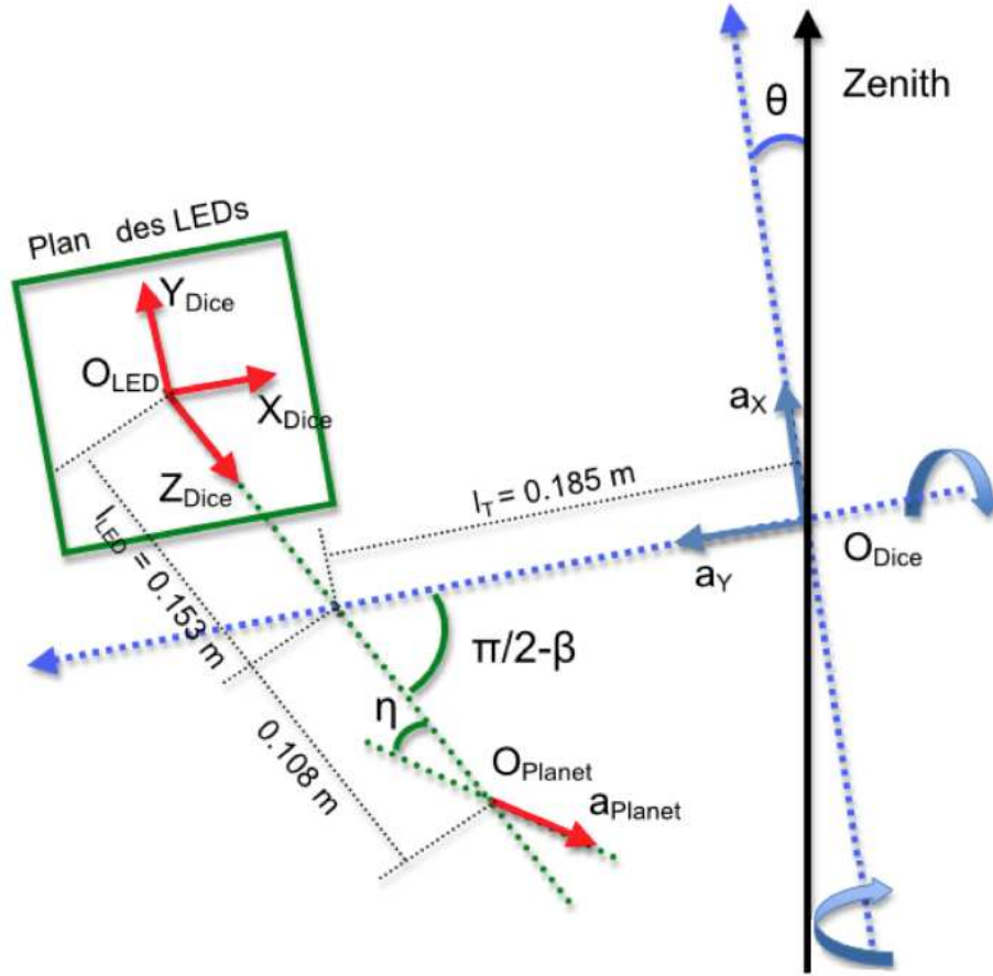
Fig. 7.7.: Schématisation des axes du repère SNDice dans le référentiel du dôme dans la position garage de la source de lumière. Les trois points, \mathcal{O}_{Dice} , \mathcal{O}_{LED} et \mathcal{O}_{Planet} avec les six axes associés sont représentés. \mathcal{O}_{Dice} se trouve à l'intersection des deux axes de rotations, \vec{a}_x et \vec{a}_y . \mathcal{O}_{LED} est placé au centre de la surface des LEDs. La position de \mathcal{O}_{Planet} coïncide avec le centre de la lentille de focalisation de la planète artificielle. Les vecteurs \vec{X}_{Dice} , \vec{Y}_{Dice} et \vec{Z}_{Dice} permettent de décrire l'orientation de SNDice. Les orientations de \vec{X}_{Dice} et \vec{Y}_{Dice} suivent celles de \vec{a}_x et \vec{a}_y , tandis que \vec{Z}_{Dice} coïncide avec l'axe optique \mathcal{A}_{LED} et point vers le est du dôme. L'orientation de la planète, \vec{a}_{Planet} , est dessinée légèrement inclinée ( \eta = 0.15^\circ ) par rapport à \vec{Z} , en respectant les désaxages causés par la lentille, (cf. §4.4.3). Il faut remarquer que les deux repères \mathcal{R}_{Dice} et \mathcal{R}_D ne sont pas alignés à cause des petits désaxages dans la monture de la source de lumière.
