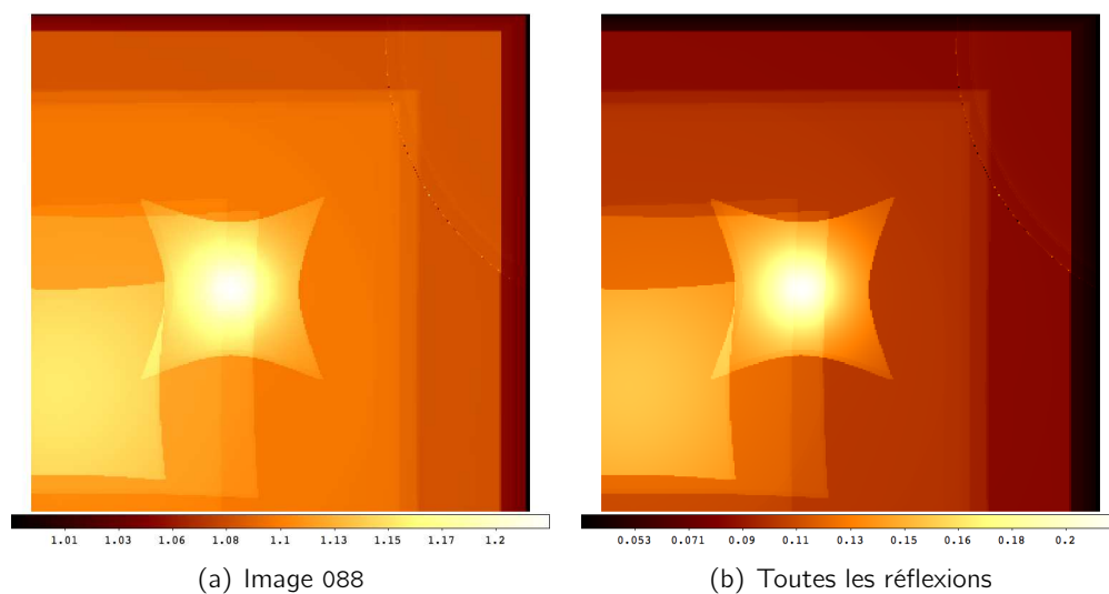
Fig. 8.13.: Simulation de la pose 088 du 12-10-2012, sur la figure (a), et des toutes les réflexions contribuant à l'illumination finale, sur la figure (b). La barre montre l'intensité de l'illumination exprimée comme pourcentage de la lumière directe. La pollution du plan focal peut atteindre environ 20% dans les régions de plus grande concentration des réflexions.
