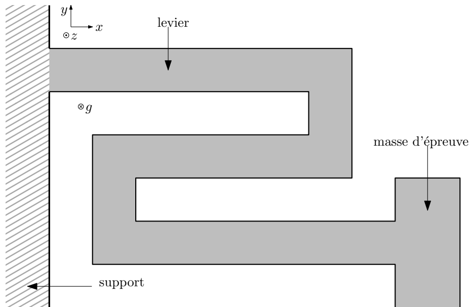
FIGURE 3.5: Gravimètre à levier replié avec poutre repliée, pour gagner en longueur de porte-à-faux tout en gardant une bonne compacité.
