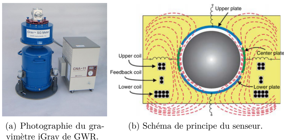
FIGURE 2.4: Gravimètre à supraconduction (images GWR).
