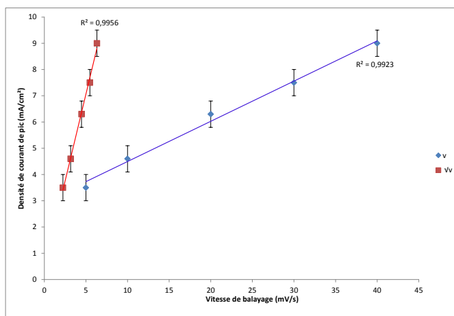
Figure 59. Effet de la vitesse de balayage v sur la densité de courant de pic de réduction de revêtements PPy/ \text{TS}^- d'épaisseur 10 \mu\text{m} élaborés à 1V/ECS. L'expérience est réalisée dans une solution aqueuse 0,1M \text{LiClO}_4 .
