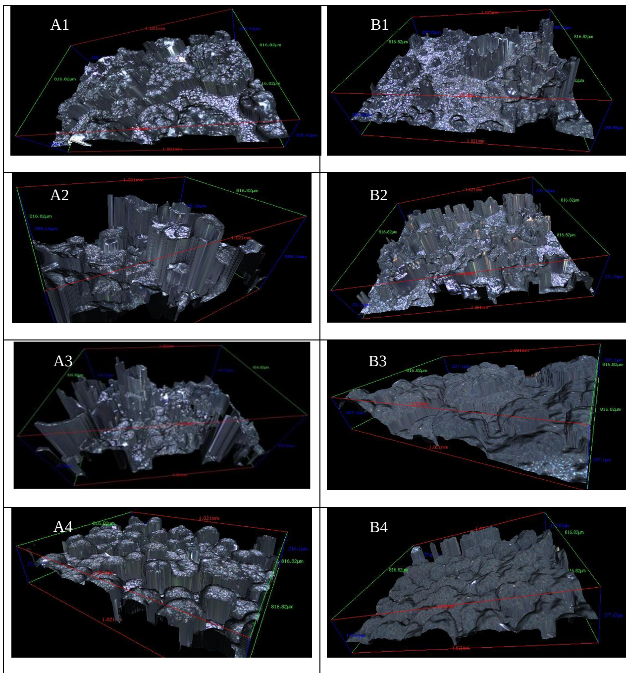
Figure 96. Images de profilométrie optique pour des films PPy électrosynthétisés (A) sans ultrasons et (B) sous ultrasons en solution aqueuse contenant (0.5M Py + 0.2M tartrate + 5 mM molybdate). Les films sont déposés à 3 V/ECS pour des densités de charge de (A1; B1) 3 C/cm 2 (A2; B2) 4 C/cm 2 (A3; B3) 5 C/cm 2 (A4; B4) 6 C/cm 2 .
