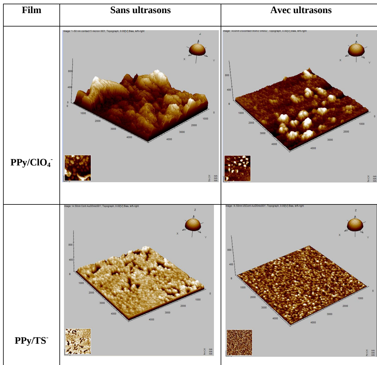
Figure 50. Images AFM de films PPy/ \text{ClO}_4^- et PPy/ \text{TS}^- sur FTO élaborés à 1V/ECS sans et sous ultrasons. Quantité de charge lors du dépôt: 25 mC/cm 2 .
