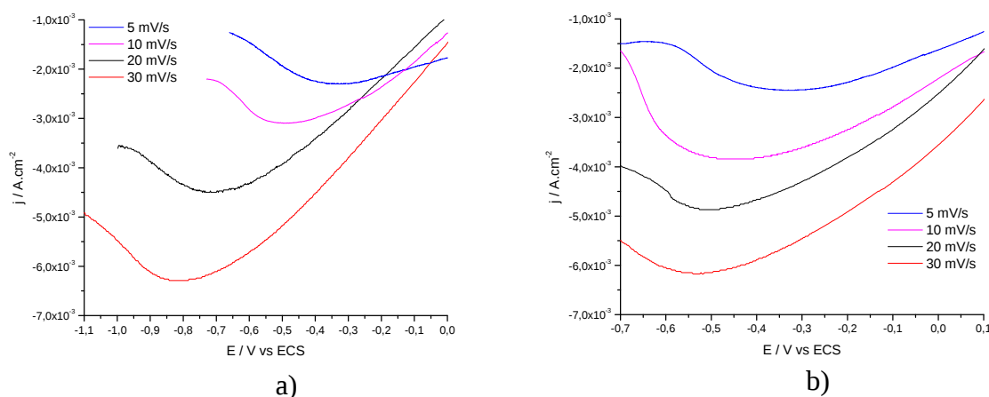
Figure 54. Courbes de polarisation cathodique de revêtements PPy/ClO 4 - d'épaisseur 10 µm élaborés a) sans ultrasons et b) sous ultrasons à 1V/ECS. L'expérience est réalisée dans une solution aqueuse 0,1M LiClO 4 .
