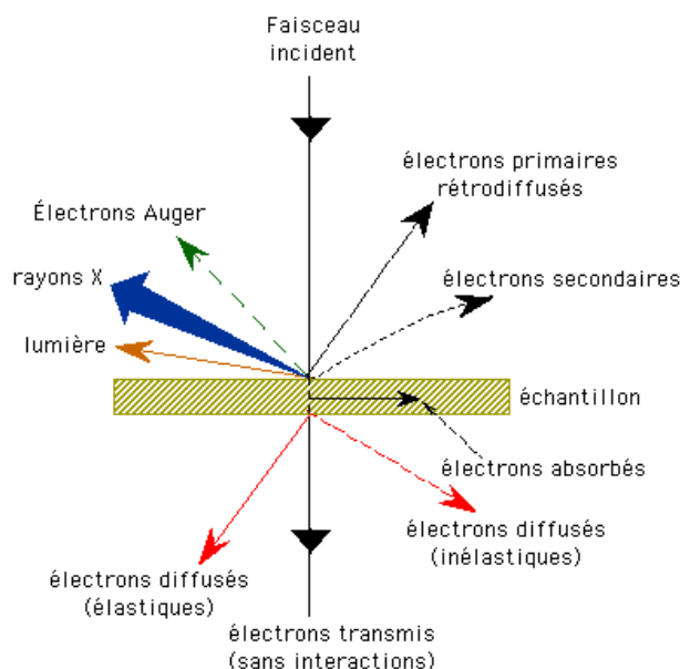
Figure 123. Phénomènes induits par l'interaction faisceau électronique/matériau.
