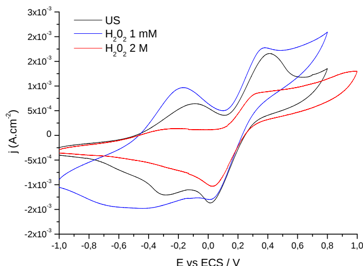
Figure 73. Cyclovoltampérométrie en solution aqueuse 10^{-2} M \text{K}_4\text{Fe}(\text{CN})_6 d'un film PPy élaboré sous ultrasons (US) en milieu (0,1\text{M Py} + 10^{-2} \text{ M } \text{K}_4\text{Fe}(\text{CN})_6) et en milieu (0,1\text{M Py} + 10^{-2} \text{ M } \text{K}_4\text{Fe}(\text{CN})_6 + 1\text{mM} ou 2 \text{ M } \text{H}_2\text{O}_2) . Vitesse de balayage : 10 \text{ mV/s} .
