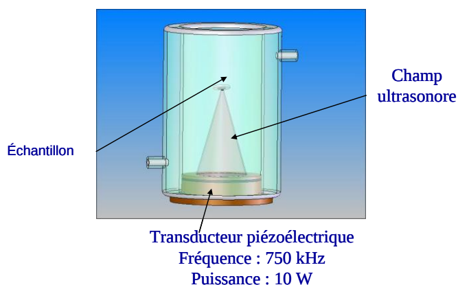
Figure 118. Schéma du montage pour le masquage sélectif aux ultrasons.
