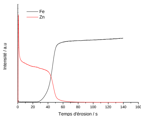
Figure 92. Profil SDL du substrat d'acier électrozingué
