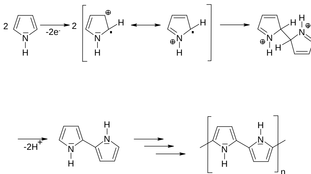
Figure 10. Mécanisme de polymérisation du polypyrrole.
