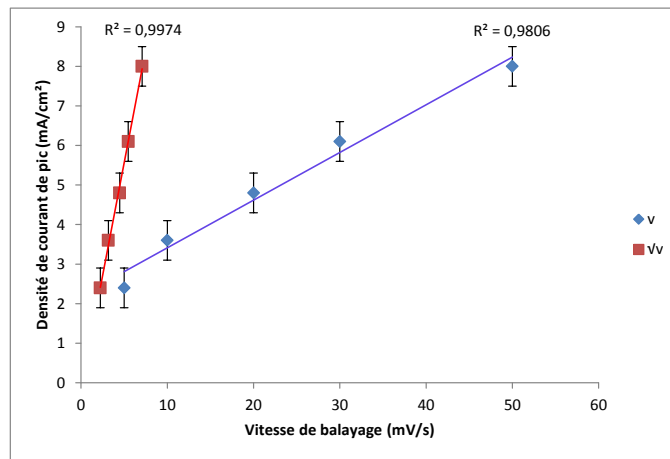
Figure 56. Effet de la vitesse de balayage v sur la densité de courant de pic de réduction de revêtements PPy/ \text{ClO}_4^- d'épaisseur 10 \mu\text{m} élaborés à 1V/ECS sous ultrasons. L'expérience est réalisée dans une solution aqueuse 0,1M \text{LiClO}_4 .
