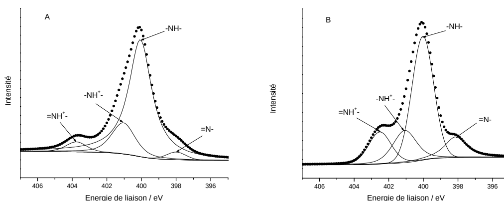
Figure 78. Région N1s du spectre XPS obtenu pour un film \text{PPy}/\text{ClO}_4^- synthétisé A) en conditions silencieuses et B) sous ultrasons.
