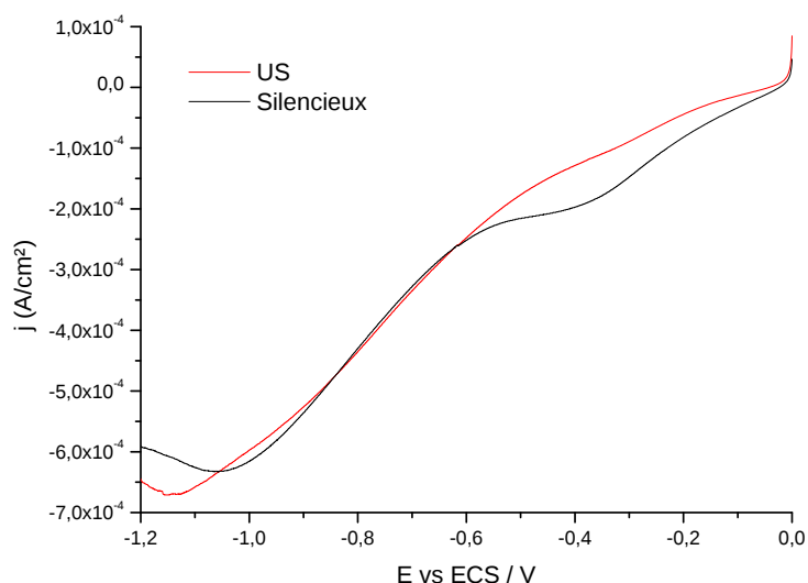
Figure 61. Dédopage électrochimique d'un film PPy/MoO 4 2- de 2 \mu\text{m} électrosynthétisé sans et sous irradiation ultrasonore. L'expérience est réalisée dans une solution aqueuse 5 mM \text{Na}_2\text{MoO}_4 . Vitesse de balayage : 5 mV/s.
