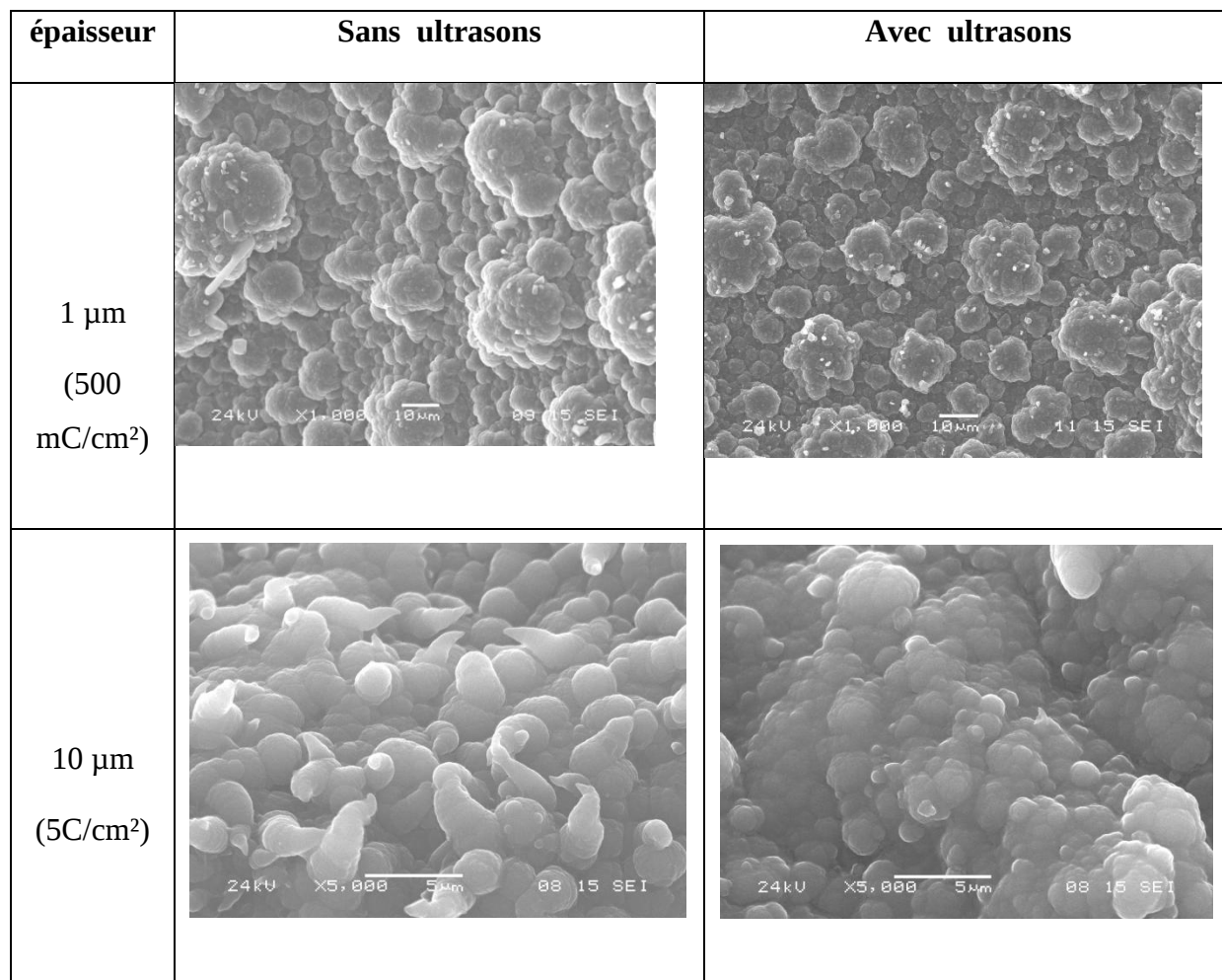
Figure 51. Images MEB de films PPy/ClO 4 - sur FTO élaborés à 1V/ECS sans et sous ultrasons.
