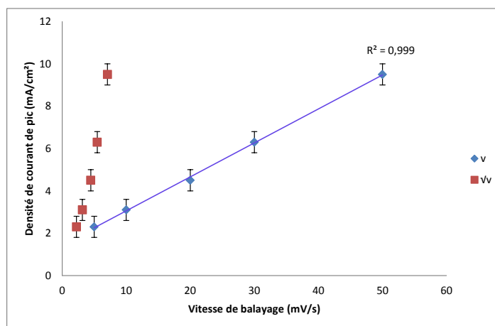
Figure 55. Effet de la vitesse de balayage v sur la densité de courant de pic de réduction de revêtements PPy/ClO 4 - d'épaisseur 10 µm élaborés à 1V/ECS en conditions silencieuses. L'expérience est réalisée dans une solution aqueuse 0,1M LiClO 4 .
