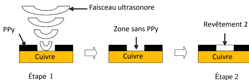
Figure 107. Étapes d'élaboration du substrat biphasé.
