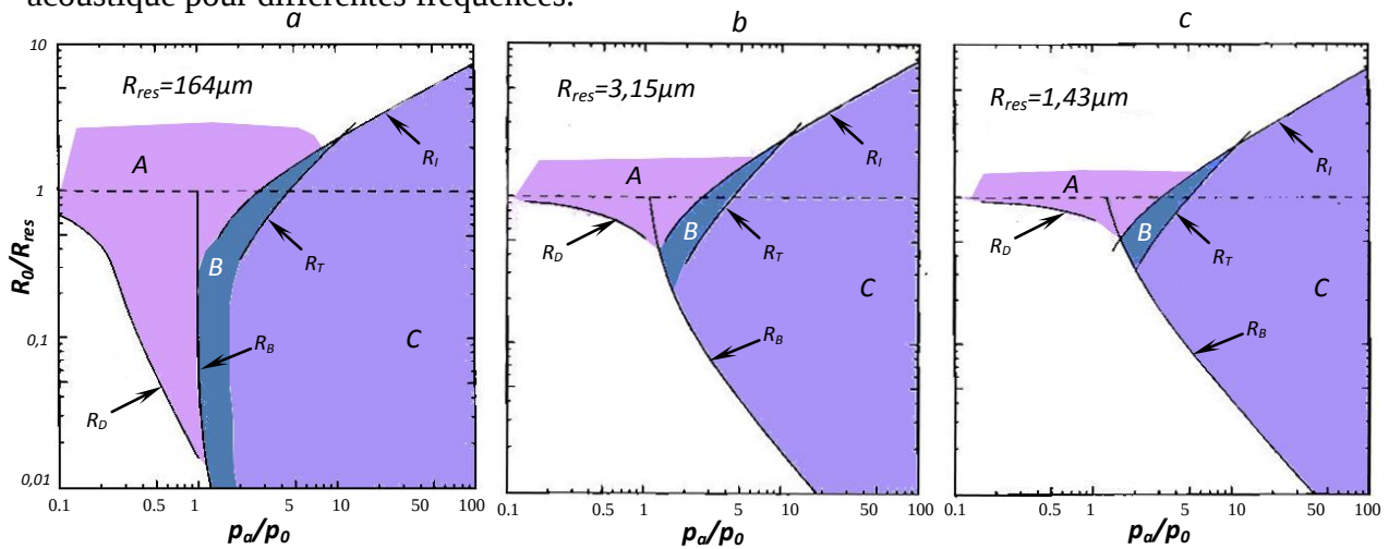
Figure 132. Prédiction de la cavitation dans l'eau saturée d'air à des fréquences de 20 kHz (a), 1 MHz (b), 2,5 MHz (c). On retrouve en abscisse le rapport de pression et le rapport des rayons en ordonnée.
