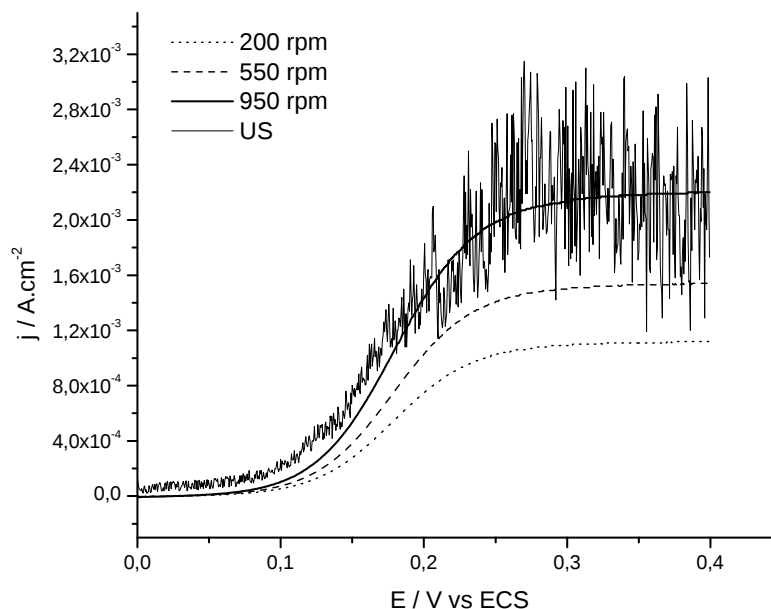
Figure 45. Polarisation anodique d'une solution aqueuse contenant 5 mM en \text{Fe(CN)}_6^{4-} + 0,2M en NaOH. Vitesse de balayage : 2 \text{ mV/s} .
