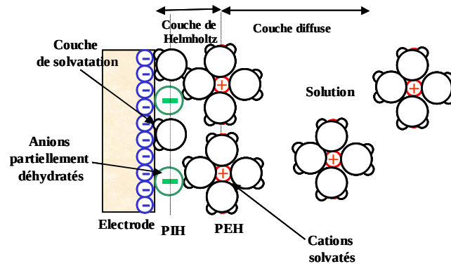
Figure 6. Modèle de Grahame de la double couche électrochimique.
