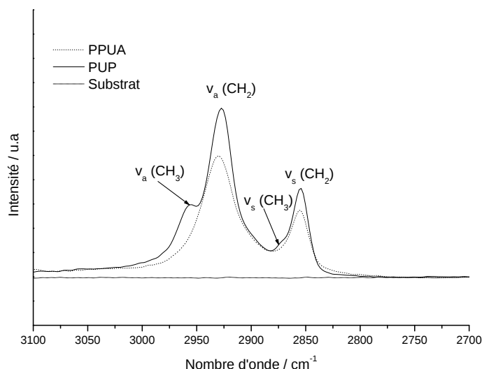
Figure 84. Région 2700-3100 cm -1 du spectre PM-IRRAS des films PPUA et PUP élaborés sur platine.
