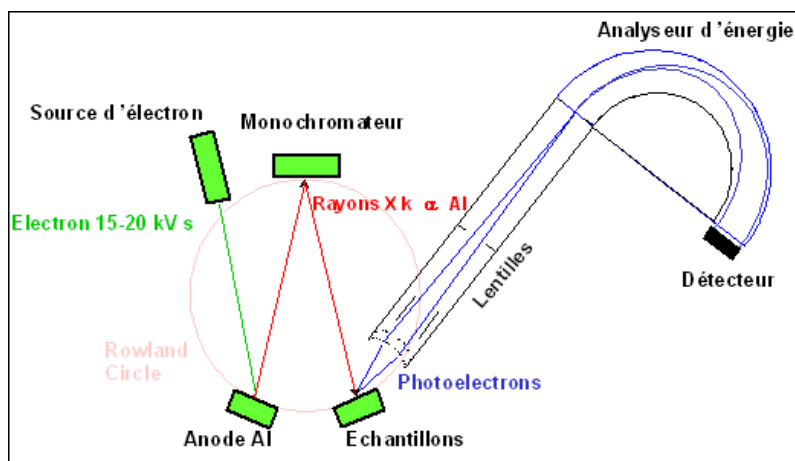
Figure 129. Représentation schématique d'un spectromètre XPS.
