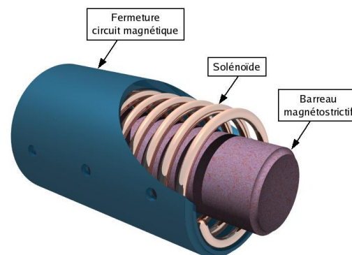
Figure 19. Principe d'un matériau magnétostrictif.
