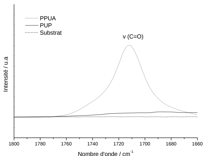
Figure 85. Région 1660-1800 cm -1 du spectre PM-IRRAS des films PPUA et PUP élaborés sur platine.
