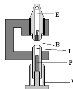
Figure 18. Sifflet de Galton.
