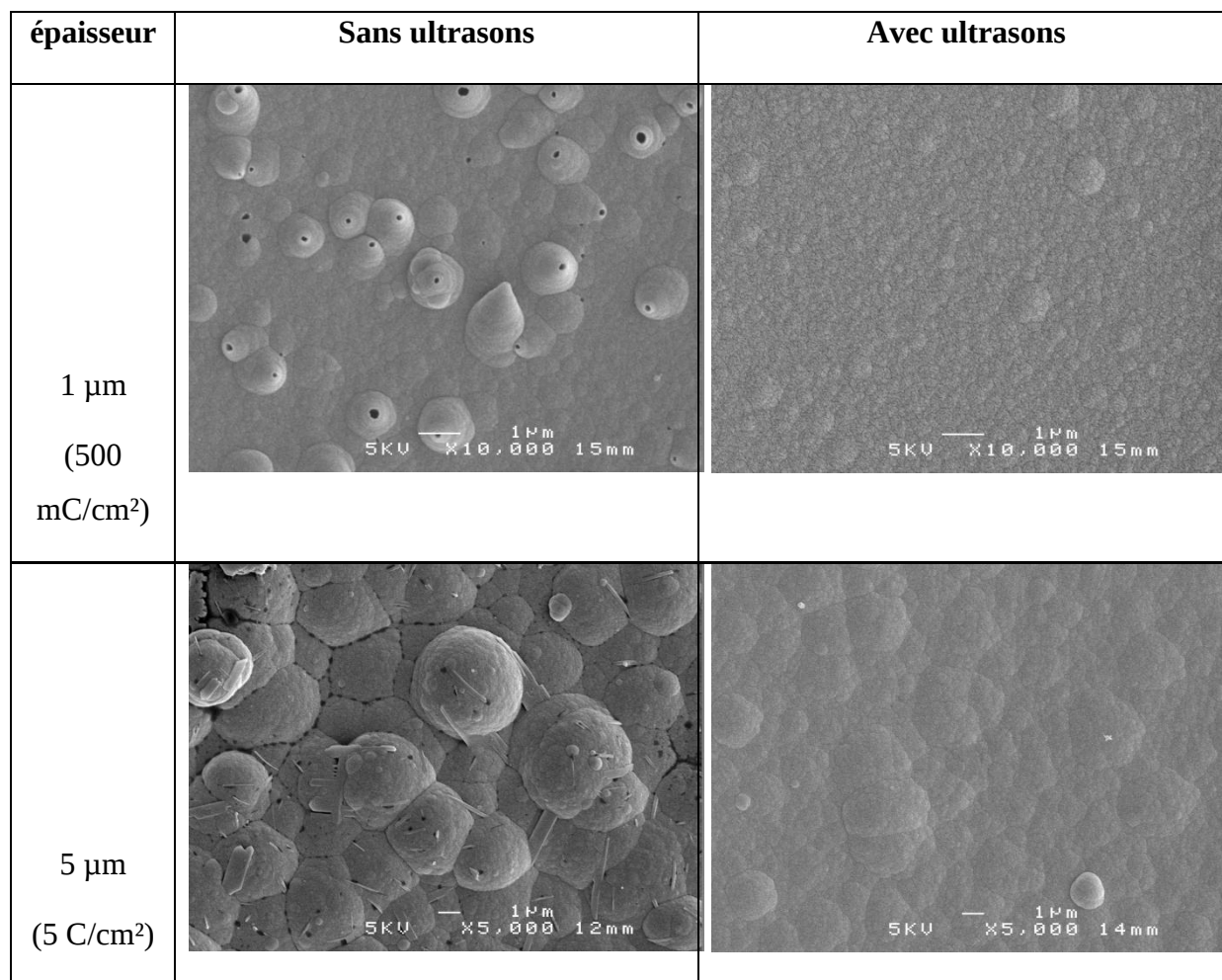
Figure 52. Images MEB de films PPy/TS - sur FTO élaborés à 1V/ECS sans et sous ultrasons.
