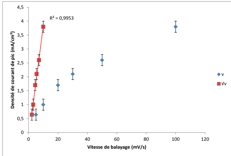
Figure 66. Effet de la vitesse de balayage v sur la densité de courant de pic de réduction (2 ème pic) de revêtements \text{PPy}/\text{MoO}_4^{2-} d'épaisseur 2\ \mu\text{m} . L'expérience est réalisée dans une solution aqueuse 5\ \text{mM}\ \text{Na}_2\text{MoO}_4 .
