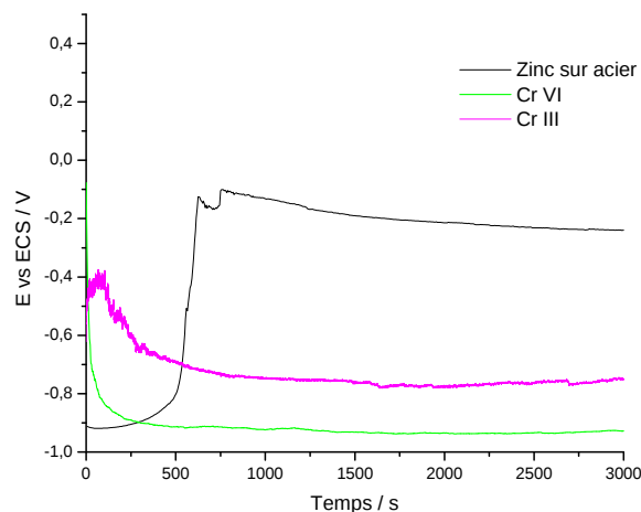
Figure 101. Chronopotentiométrie à j fixée ( 10 \text{ mA/cm}^2 ) dans une solution de NaCl (3,5% wt) d'un substrat d'acier zingué traité par revêtement Cr (III) et Cr (VI).
