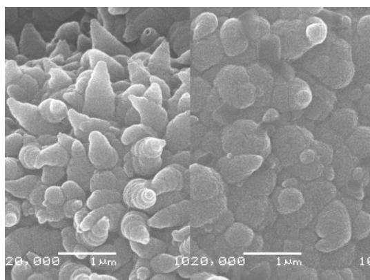
Figure 91. Images MEB d'un film PPy/ClO 4 - de 1 \mu\text{m} synthétisé à 1V/ECS sur platine en conditions silencieuses (à gauche) et sous ultrasons (droite).
