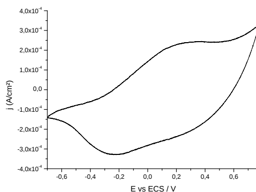
Figure 53. Cyclovoltamogramme d'un film \text{PPy}/\text{ClO}_4^- de 10 \mu\text{m} réalisé dans une solution aqueuse 0,1M \text{LiClO}_4 . Vitesse de balayage : 5 mV/s.
