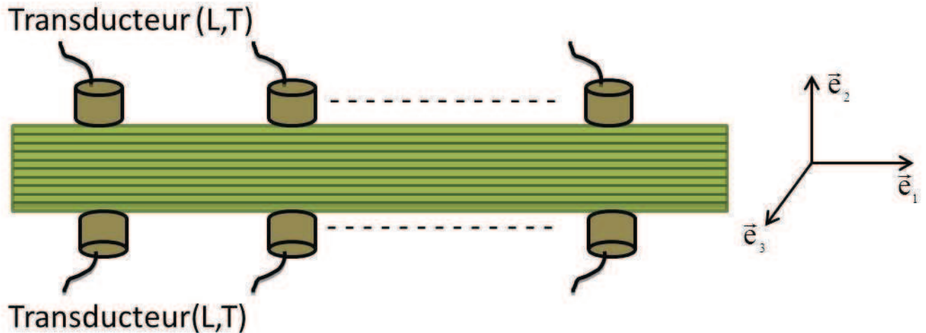
Figure 2.2 : Axes de symétrie du composite isotrope transverse.
