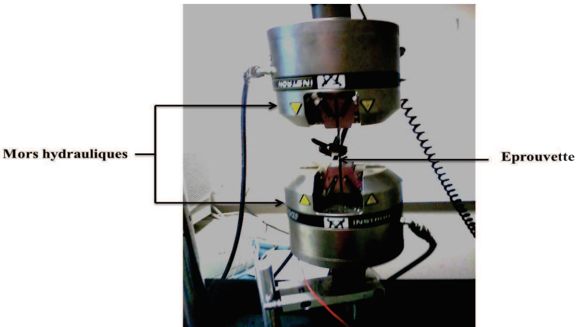
Figure 3.1 : Essai de fatigue exécuté sur un composite à matrice métallique.
