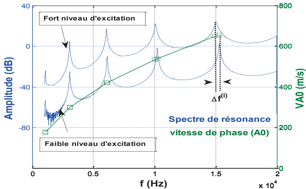
Figure 3.15 : Courbe de dispersion du mode de Lamb fondamental antisymétrique A0 obtenu à partir du spectre de la résonance des ondes de flexion dans le cas d'un composite à matrice métallique TA6V.
