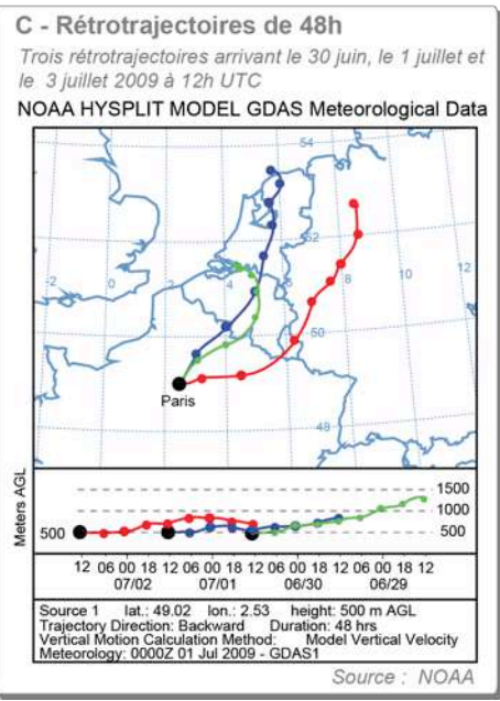
Figure VI.2 : Variabilité spatiale et temporelle des concentrations d'O 3 (A et B) et facteurs météorologiques explicatifs (C et D) du 30 juin au 2 juillet 2009
