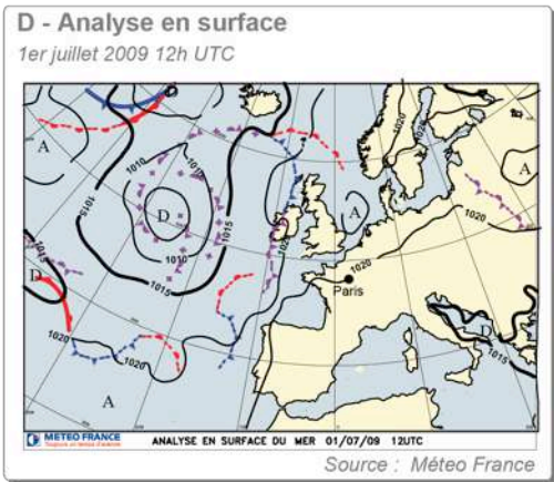
Figure VI.2 : Variabilité spatiale et temporelle des concentrations d'O 3 (A et B) et facteurs météorologiques explicatifs (C et D) du 30 juin au 2 juillet 2009
