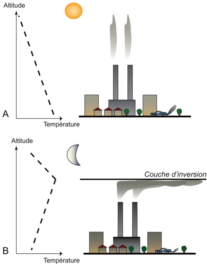
Figure I.6 : Variation de la couche limite urbaine entre le jour (A) et la nuit avec une inversion thermique (B)
