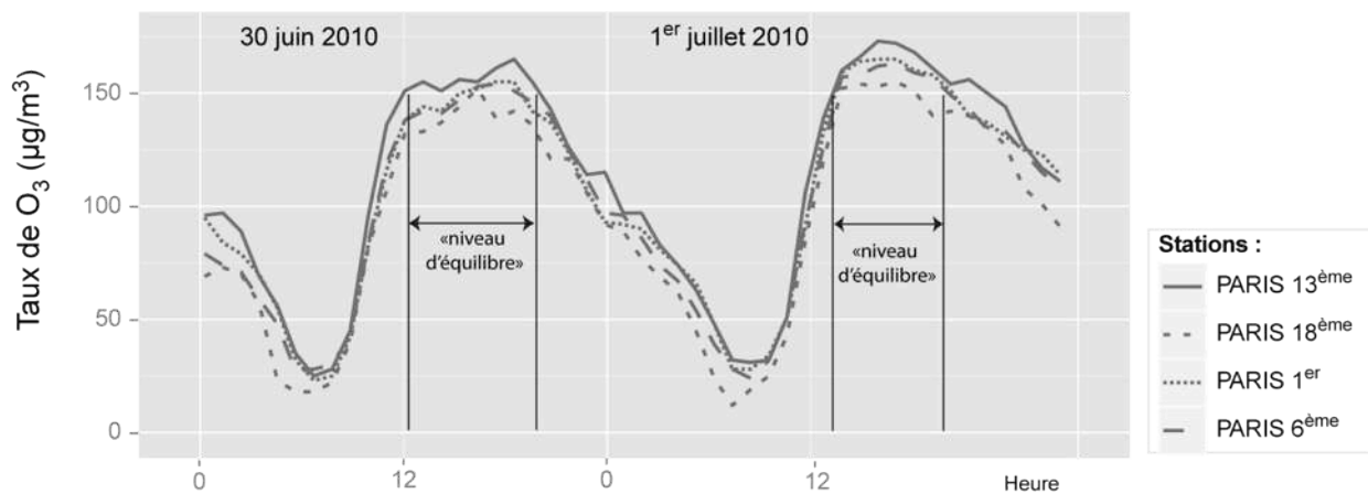
Figure VII.9 : Variabilité des concentrations horaires d'ozone mesurée dans les stations parisiennes du réseau Airparif ; source des données : Airparif*
