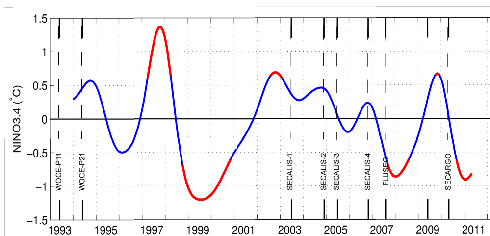
Figure V.2: Indice NINO3.4 (filtre Hanning à 25 mois) (Barnston et al. , 1997). Événement El Niño définit lorsque NINO3.4 > 0.6^\circ C ; Évènement La Niña définit lorsque NINO3.4 < -0.6^\circ C (en rouge).
