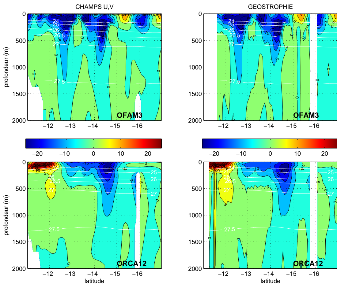
Figure III.13: Sections de vitesses totales (a,c) et géostrophiques (b,d) à 162.5^{\circ}\text{E} en \text{cm}\cdot\text{s}^{-1} issues du modèle OFAM3 au 1/10^{\circ} (a,b) et ORCA12 au 1/12^{\circ} (c,d) pour le mois de Novembre 2006. Les vitesses géostrophiques sont référencées à 2000 m. Les isopycnes \sigma=24, 25, 26, 26.5, 27 et 27.5 sont indiquées par les lignes blanches.
