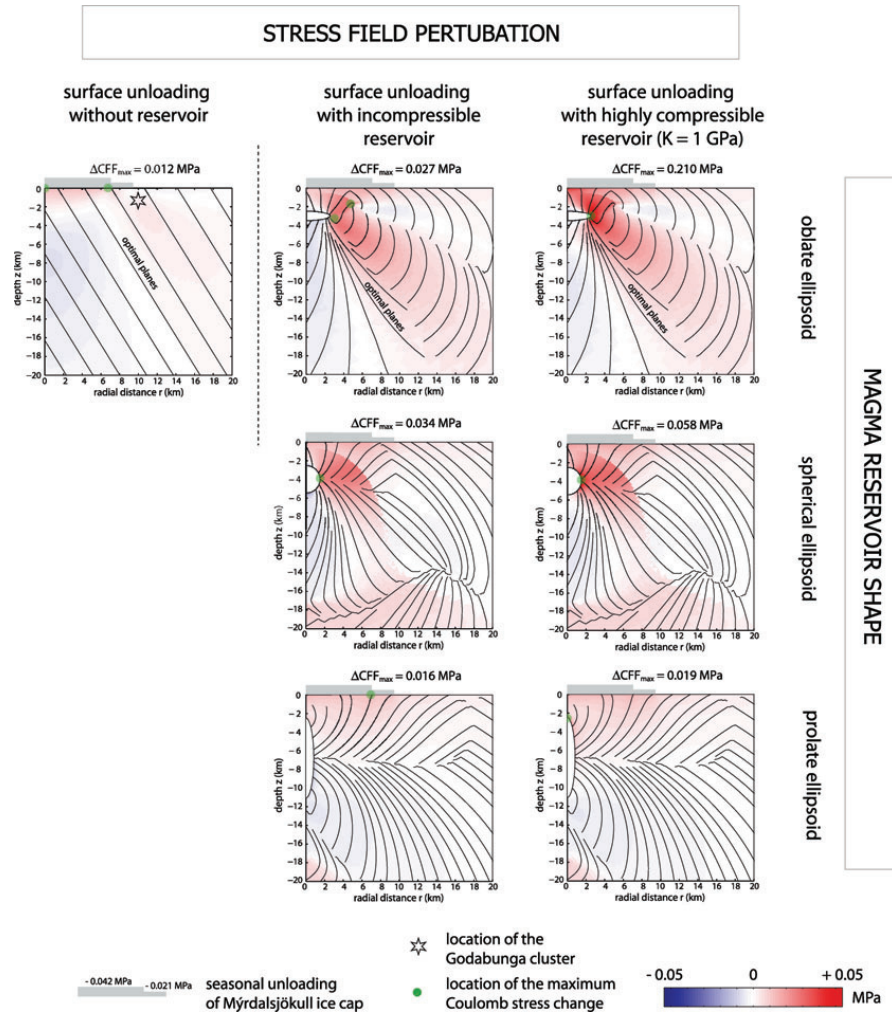
Figure 4.8. Variation de la contrainte de Coulomb induite par la fonte de la neige sur la calotte glaciaire de Myrdalsjökull en Islande. Même décharge, géométrie de réservoir et paramètre que dans la figure 4.7. Le coefficient de friction est pris égal à 0.5. Différentes formes de réservoir (ellipticité de 5, 1 et 2/5) et compressibilités du magma sont prises en compte. \Delta CFF est calculé pour des plans de failles radiaux induits par la pressurisation du réservoir. Le cas sans réservoir pour un régime de faille en contexte extensif est calculé comme référence. L'étoile noire est pour la localisation du cluster de sismicité saisonnière observé. Pour chaque modèle, la localisation et l'amplitude du maximum de variation de contrainte de Coulomb est reporté. D'après Albino et al. (2010).
