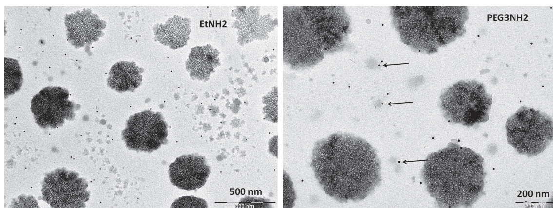
FIGURE 6.22 – Clichés de MET obtenus après incubation des NPs d’or-streptavidine avec les NPs à couronne P(AA 0,5 - co -APEO 0,5 ) 22 greffées biotine présentant différents liens entre la biotine et l’AA. Gauche : EtNH 2 . Droite : PEO 3 (NH) 2 . Les flèches représentent les possibles complexes NPs or-streptavidine/NPs polymères-biotine.
