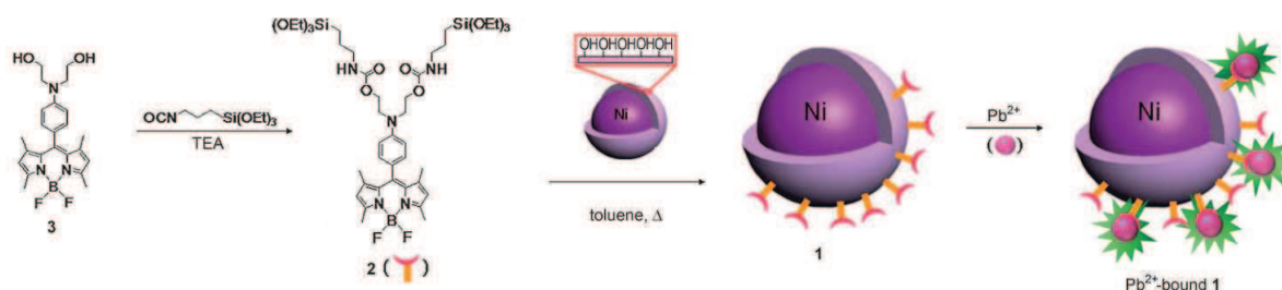
SCHÈME 1.3 – Synthèse des nanosenseurs au plomb, magnétiques, fonctionnalisés par du BODIPY de Jung et coll. [145]. Utilisé avec permission depuis Hye Young Lee et coll., A Selective Fluoroionophore Based on BODIPY-functionalized Magnetic Silica Nanoparticles : Removal of Pb 2+ from Human Blood, Angewandte Chemie International Edition, 48, 1239-1243, 2009. Droits d'auteur 2009 John Wiley and Sons.
