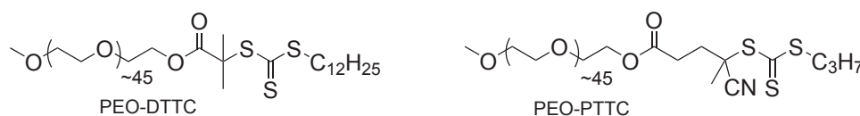
FIGURE 1.22 – Structure des macro-agents RAFT pegylés utilisés dans la référence [271] pour la polymérisation en miniémulsion du styrène.
