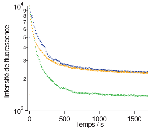
FIGURE 5.14 – Étude du photoblanchiment de NPFs à cœur BDPMA ( [BDPMA] \approx 0,1 \text{ mol/L}_S ) et à couronne PEO- b -PAA ( \dots ) ou P(AA 0,5 - co -APEO 0,5 ) 22 mesurées à trois jours d'intervalle (J : \dots , J + 3 : \dots ). Mesures réalisées sur une surface d'analyse de 3,25 \times 10^{-9} \text{ m}^2 avec une puissance laser de 3,1 mW ( \lambda_{exc} = 515 \text{ nm} , 10 MHz, 400 fs).
