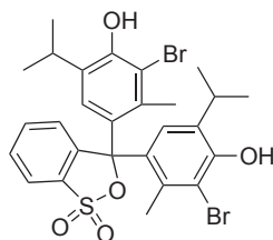
SCHÈME 6.2 – Bleu de Bromothymol sous sa forme acide.
