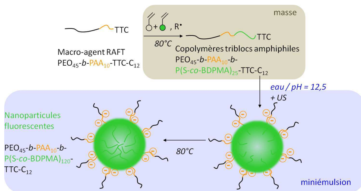
SCHÈME 2.4 – Synthèse de NPs fluorescentes à cœur poly(styrène-co-BDPMA), stabilisées par des macro-agents RAFT \text{PEO-}b\text{-PAA-TTC} , par une polymérisation RAFT en miniémulsion "one-pot", deux étapes.
