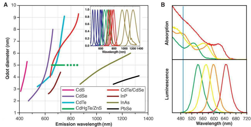
FIGURE 1.13 – A. Longueurs d'ondes maximales d'émission de luminescence corrélées à la taille et à la nature de cœur de différents QDs. Insert : spectres d'émission de luminescence pour certaines natures de cœur. B. Spectres d'absorption et d'émission de fluorescence de QDs CdSe/ZnS. Le trait plein correspond à la longueur d'onde d'un laser à argon ( \lambda_{exc} = 488 \text{ nm} ) pouvant être utilisé pour exciter les QDs (issu de [91])
