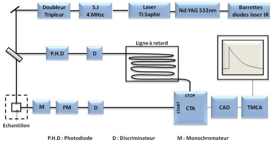
FIGURE 7.2 – Montage expérimental utilisé pour enregistrer les déclinés de fluorescence.
