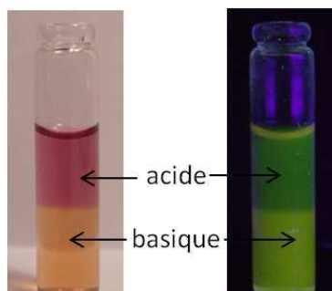
FIGURE 6.4 – Photographies des NPFs greffées NR en milieu acide (pH 2) (haut) et basique (pH 12) (bas). Gauche : à la lumière du jour et droite : sous éclairage UV ( \lambda_{exc} = 365 nm).
