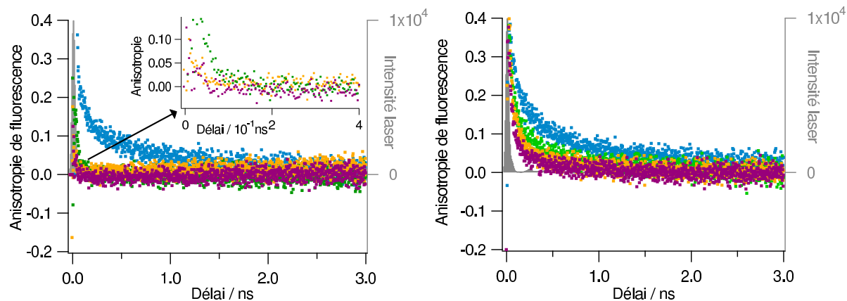
FIGURE 3.12 – Anisotropies résolues en temps des nanoparticules à différents taux de BDPMA par chaîne (0,3 \bullet\bullet\bullet , 1,1 \bullet\bullet\bullet , 2,1 \bullet\bullet\bullet , 3,0 \bullet\bullet\bullet ) ( \lambda_{exc} = 495 nm, \lambda_F = 543 nm) et impulsion laser (-). Gauche : dans l'eau. Droite : dans le toluène.
