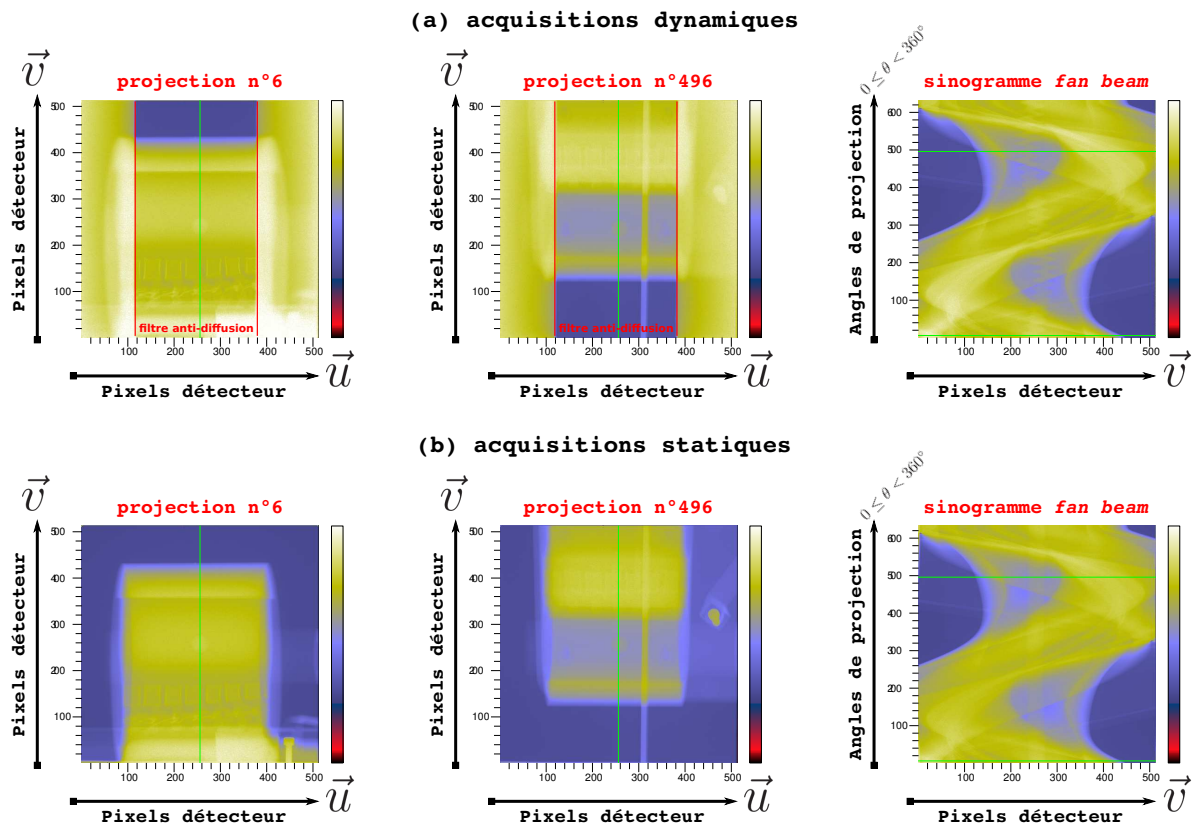
FIGURE 3.46: Données du fantôme dynamique mécanique, acquises sur le scanner Cone Beam du Centre Léon Bérard. (a) L'insert sphérique est animé d'un mouvement périodique sinusoïdal, au cours de l'acquisition des quelques 630 projections. (b) L'insert sphérique est immobile au cours de l'acquisition. La ligne détecteur horizontale médiane a été extraite pour obtenir des données fan beam permettant des reconstructions 2-D. Pour les acquisitions dynamiques, un filtre anti-diffusion a été appliqué avant le détecteur, dans la zone d'intérêt.
