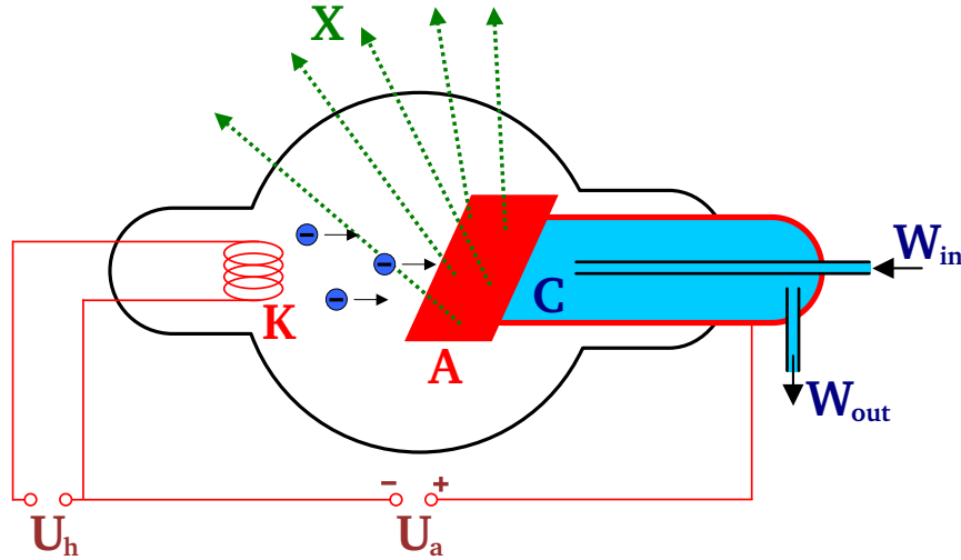
FIGURE 1.6: Schéma de principe d'un tube à rayons X de type Coolidge. Un filament de tungstène K , constituant la cathode, est chauffé par un courant électrique (créé sous la tension U_h ), lui arrachant des électrons. Ceux-ci sont accélérés par la différence de potentiel U_a entre la cathode et l'anode A , constituant la cible. Ces électrons viennent alors interagir avec les atomes de la cible en traversant leurs couches électroniques. Ces interactions — déviations, collisions — engendrent alors l'émission du rayonnement X. Source : http://commons.wikimedia.org/wiki/File%3ARoentgen-Roehre.svg .
