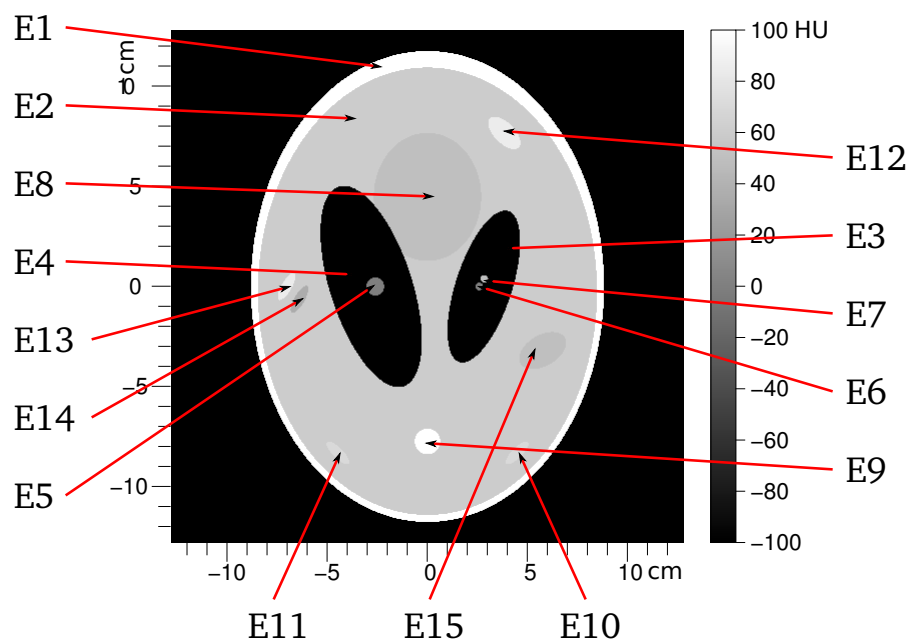
FIGURE 3.9: Tranche temporelle à \iota = 0 du fantôme dynamique type Shepp-Logan 25,6 \times 25,6\text{cm} , composé de 15 ellipses \mathcal{E}_i identifiées sur le graphe. La dynamique des valeurs d'atténuation est affichée en unités Hounsfield, avec \mu_{\text{eau}} = 0,1928\text{cm}^{-1} .
