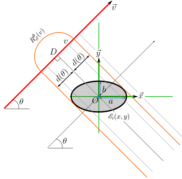
FIGURE 1.17: Schéma de la transformée de Radon R_{\mathcal{E}_i}^\theta(v) d'une ellipse \mathcal{E}_i centrée (x_0 = y_0 = 0) et non-inclinée (\alpha = 0) , pour un mode de propagation parallèle des rayons X et une orientation \theta du détecteur.
