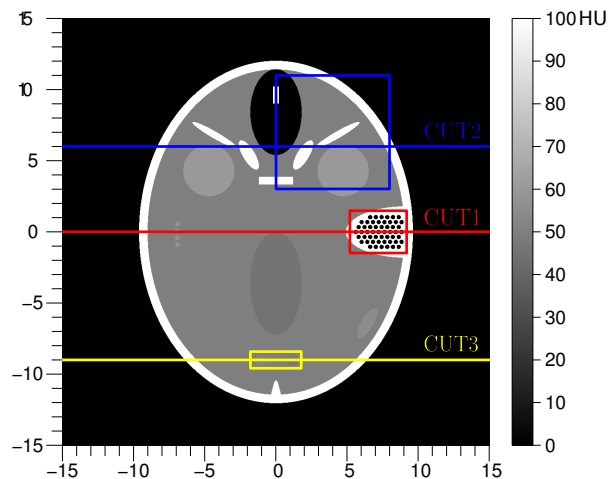
FIGURE 2.43: Identification sur le fantôme de référence FORBILD f_{\text{ref}} 1000 \times 1000 , des trois coupes CUT1 (rouge), CUT2 (bleu) et CUT3 (jaune), définies pour la comparaison des reconstructions 2-D.
